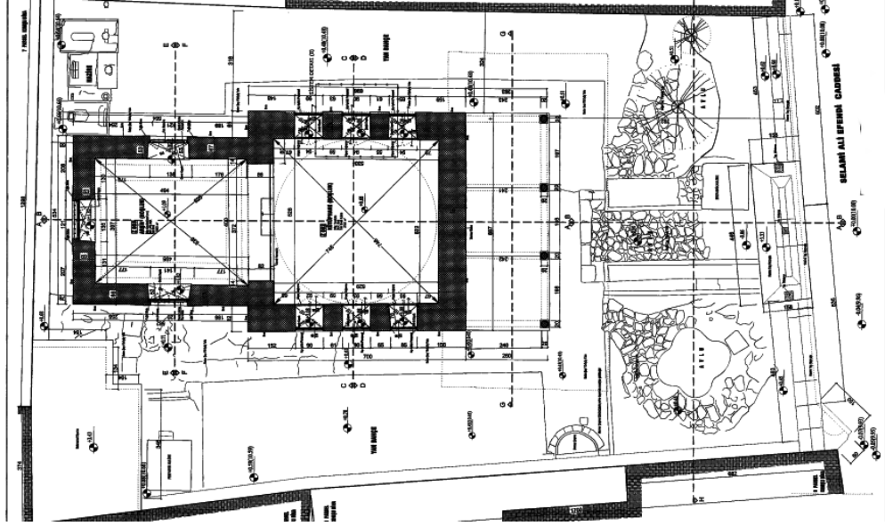
Şekil 4.97: Hacı Selim Ağa Kütüphanesi planı (KTVKK İstanbul 6 numaralı Bölge Müdürlüğü).
