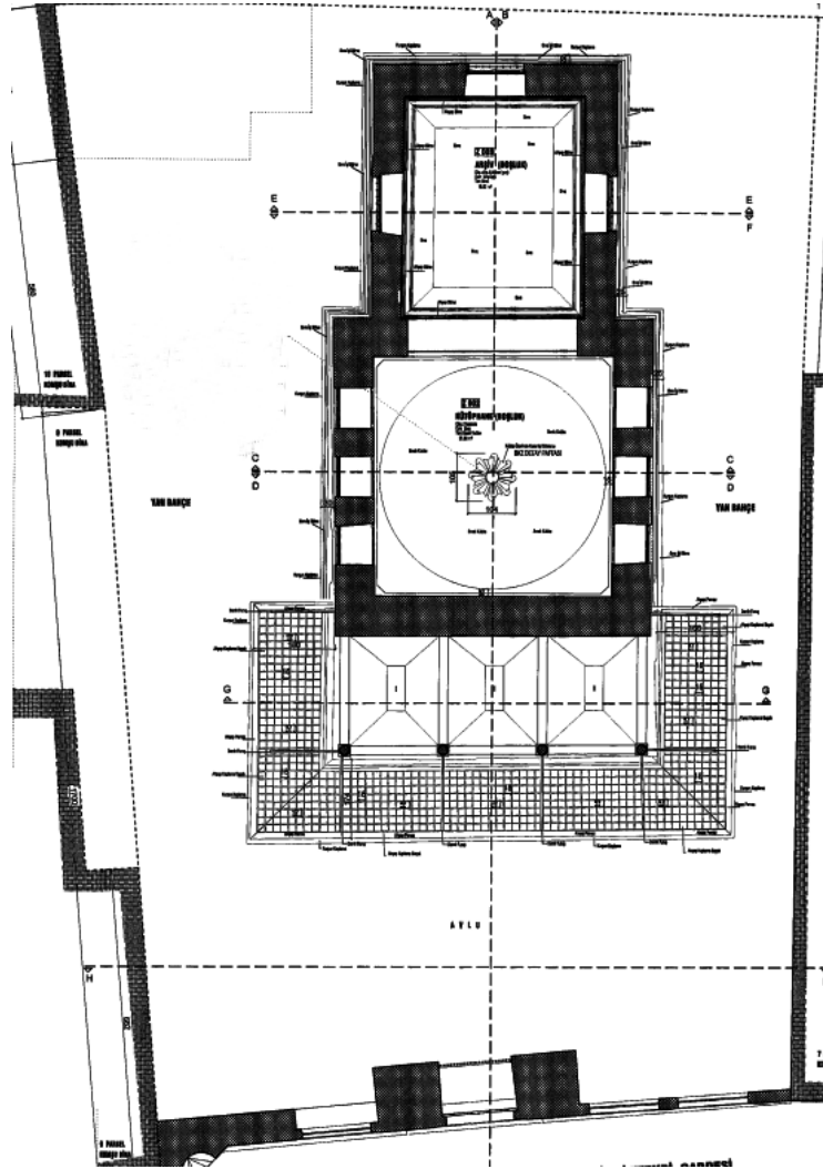
Şekil 4.105: Hacı Selim Ağa Kütüphanesi tavan örtü planı (KTVKK İstanbul 6 numaralı Bölge Müdürlüğü).
