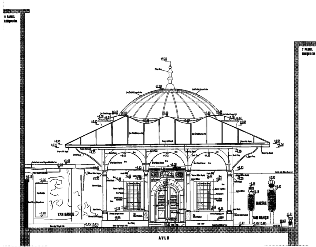
Şekil 4.107: Hacı Selim Ağa Kütüphanesi giriş cephesi (KTVKK İstanbul 6 numaralı Bölge Müdürlüğü).
