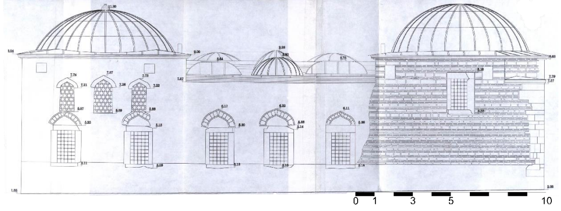
Şekil 4.30: Feyzullah Efendi Kütüphanesi Macarlar Caddesi cephesi ( Atatürk Kitaplığı ).
