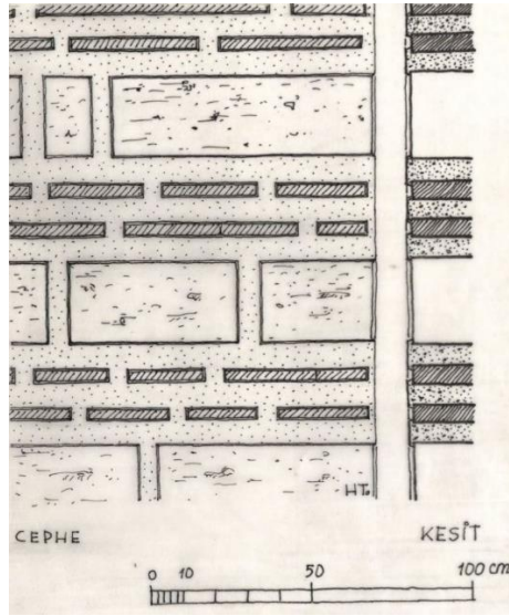
řekil 4.22: Feyzullah Efendi-Millet Kütüphanesi almařık düzen duvar detayı (Atatürk Kitaplıđı).
