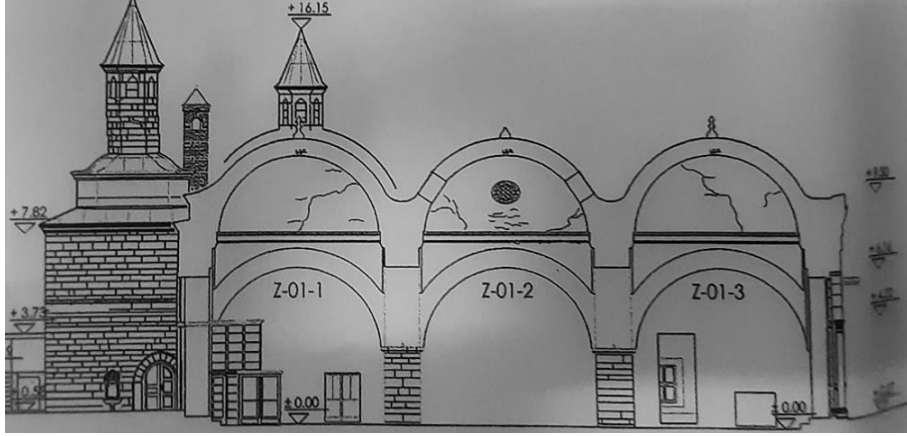
Şekil 4.114: Beyazıt Umumi Kütüphanesi kesiti (VGM İstanbul 1. Bölge Arşivi).
