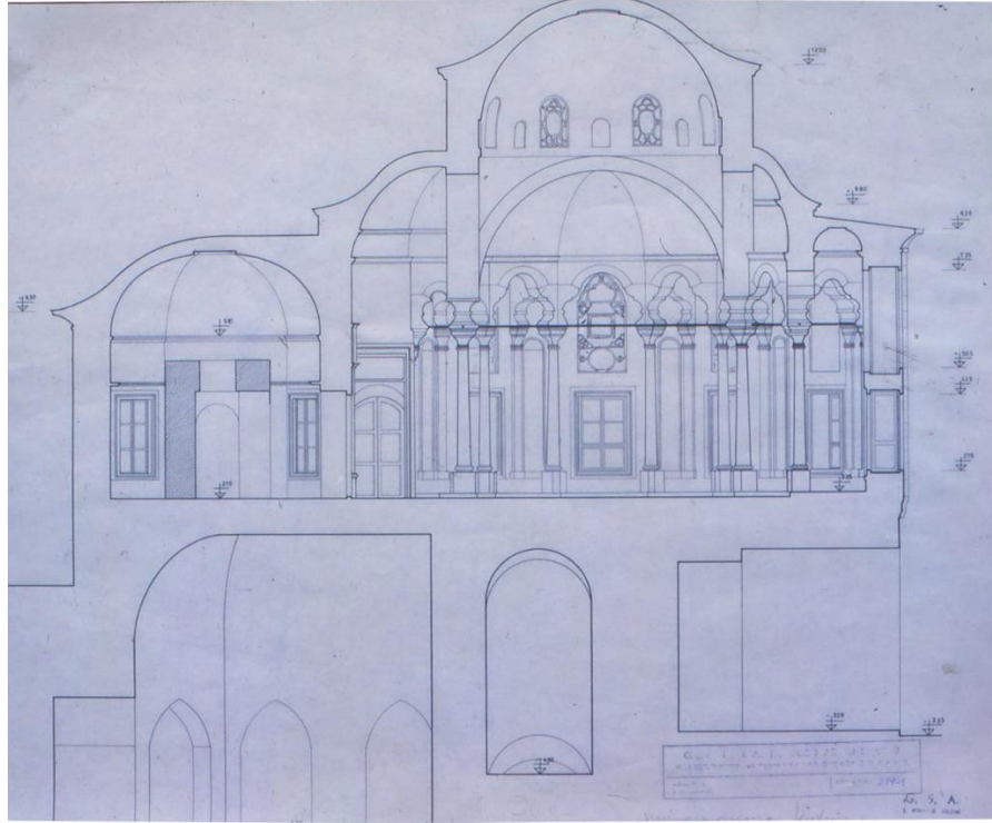
Şekil 4.80: Nuruosmaniye Kütüphanesi kesiti (Atatürk Kitaplığı).
