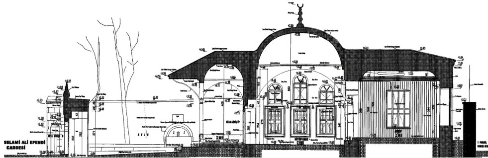
Şekil 4.98: Hacı Selim Ağa Kütüphanesi kesiti (KTVKK İstanbul 6 numaralı Bölge Müdürlüğü).
