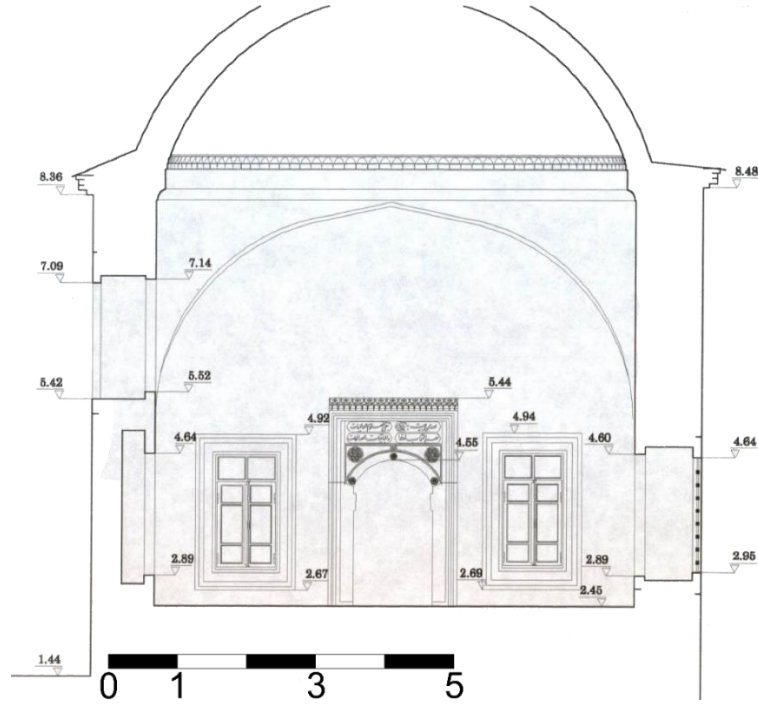
Şekil 4.44: Feyzullah Efendi Kütüphanesi kesiti (Atatürk Kitaplığı).
