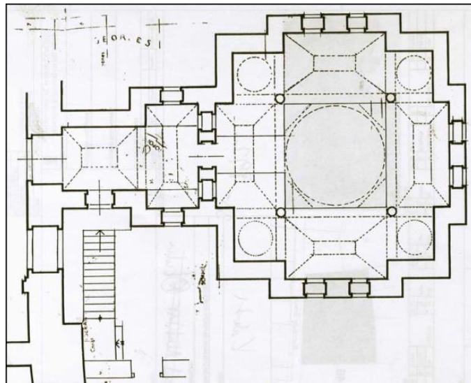
Şekil 4.72: Fatih Kütüphanesi planı (Asuman Budak, 2006).
