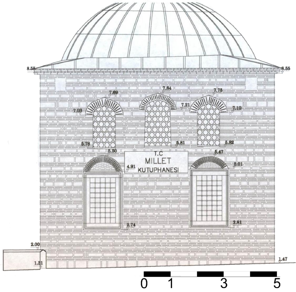
Şekil 4.35: Feyzullah Efendi Külliyesi dersane/mescit cephesi (Atatürk Kitaplığı).
