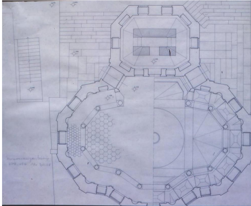
Şekil 4.79: Nuruosmaniye Kütüphanesi planı (Atatürk Kitaplığı).
