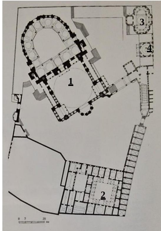
Şekil 4.78: Nuruosmaniye Külliyesi vaziyet planı (Kuban, 1998). 1-Nuruosmaniye Camii, 2-Medrese, 3- Kütüphane, 4- Türbe.
