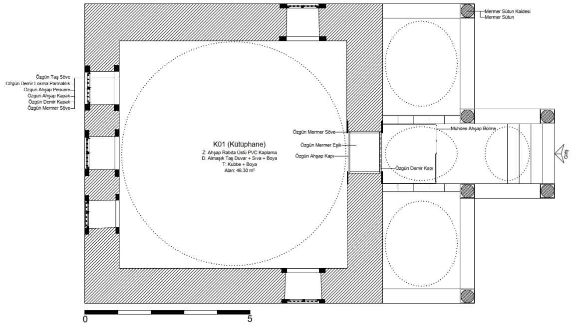
Şekil 4.6: Köprülü Kütüphanesi planı (VGM Arşiv’inden işlenerek).
