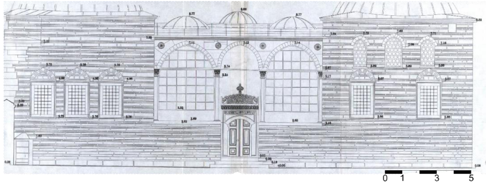
Şekil 4.37: Feyzullah Efendi Kütüphanesi avlu cephesi (Atatürk Kitaplığı).
