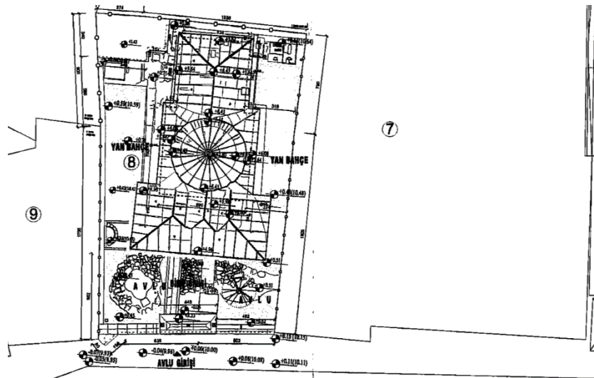
Şekil 4.96: Hacı Selim Ağa Kütüphanesi vaziyet planı (KTVKK İstanbul 6 numaralı Bölge Müdürlüğü).
