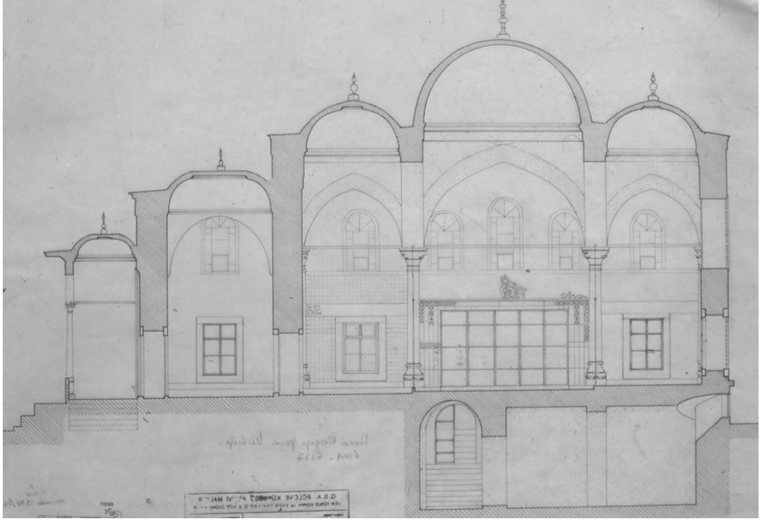
Şekil 4.88: Ragıp Paşa Kütüphanesi kesiti (Atatürk Kitaplığı).
