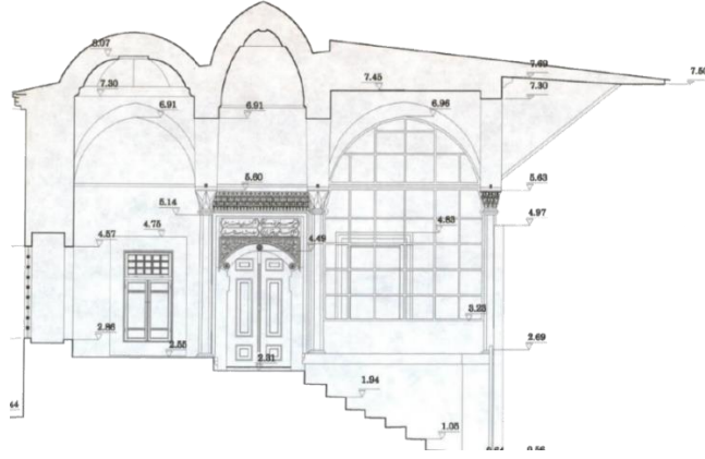
Şekil 4.41: Feyzullah Efendi kütüphane ve dersane/mescit yapısı ara mekân kesiti (Atatürk Kitaplığı).
