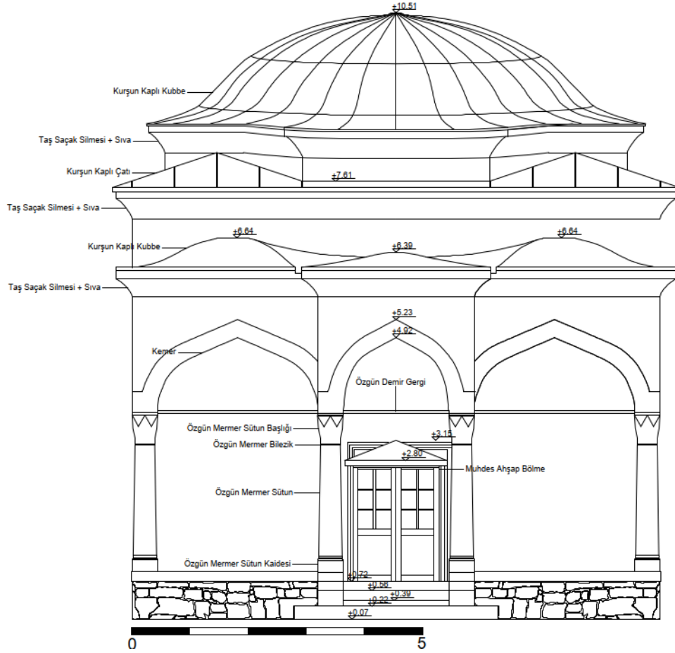
Şekil 4.9: Köprülü Kütüphanesi giriş cephesi (VGM Arşivi'nden işlenerek).
