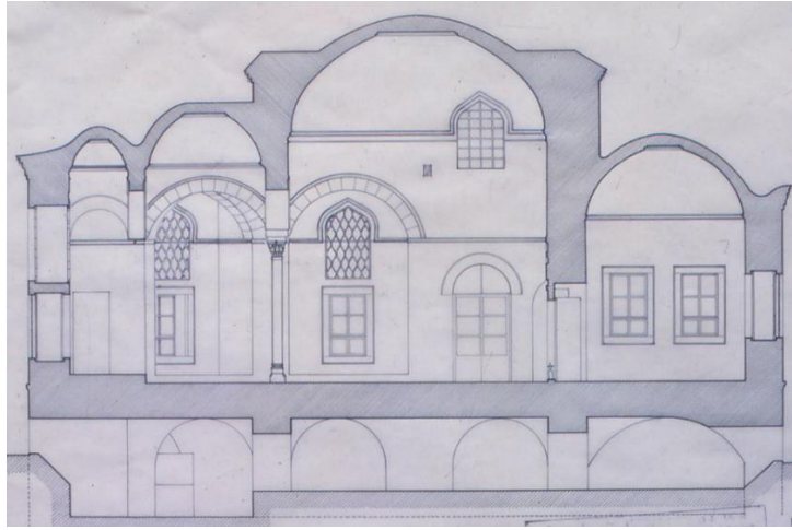
Şekil 4.55: Atıf Efendi Kütüphanesi kesiti ( Atatürk Kitaplığı ).
