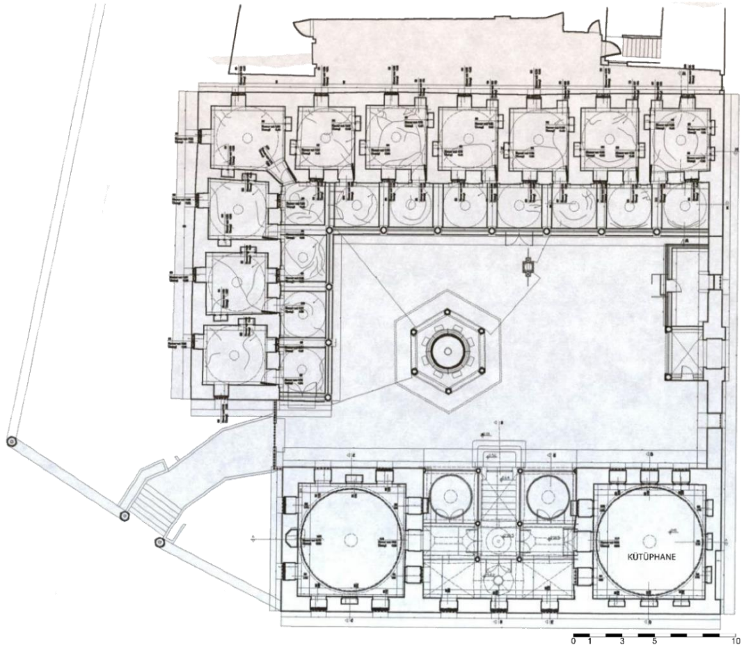
Şekil 4.16: Feyzullah Efendi -Millet Kütüphanesi planı (Atatürk Kitaplığı).
