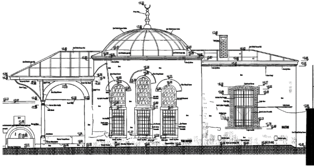
Şekil 4.109: Hacı Selim Ağa Kütüphanesi yan cephesi (KTVKK İstanbul 6 numaralı Bölge Müdürlüğü).
