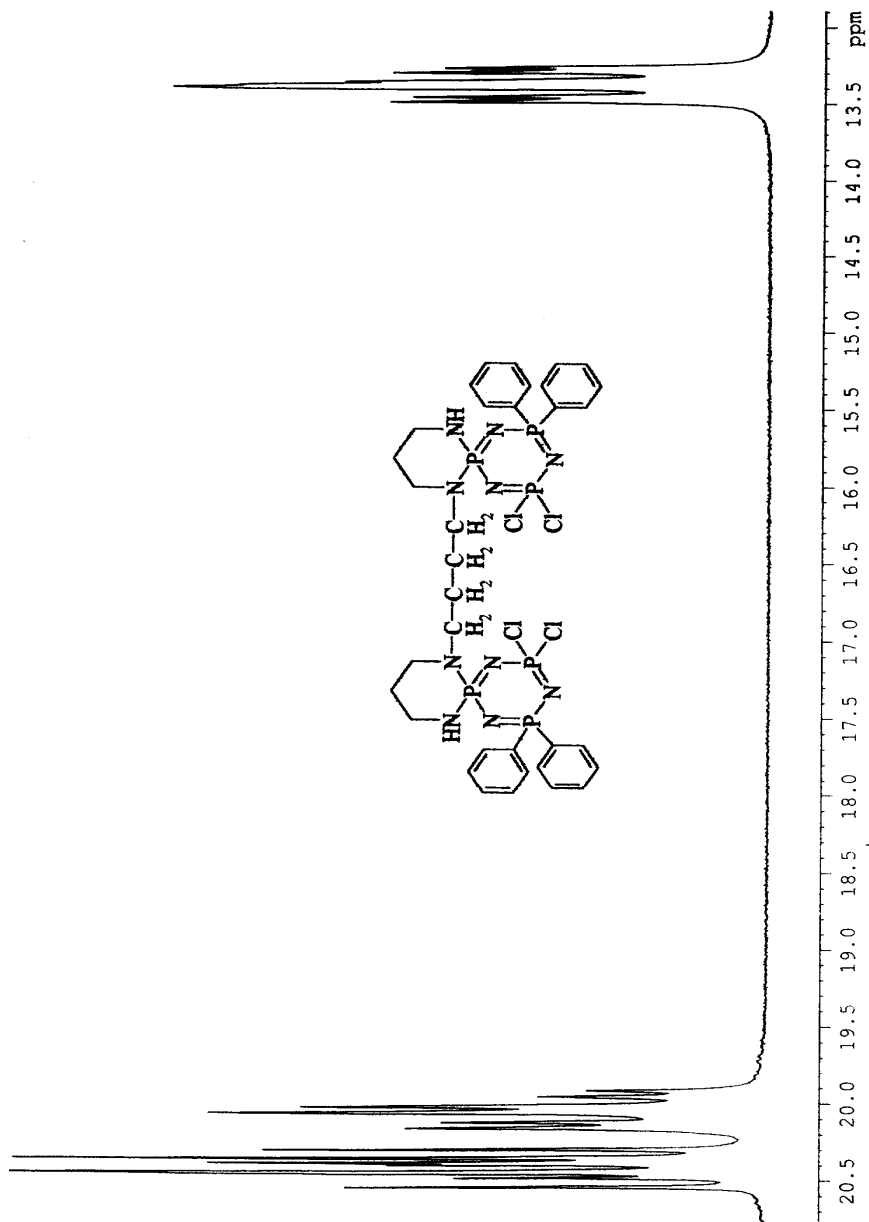
Spektrum 6.12 : III Numaralı Bileşiğin Proton ile Eşleşmiş ^{31}\text{P} NMR Spektrumu
