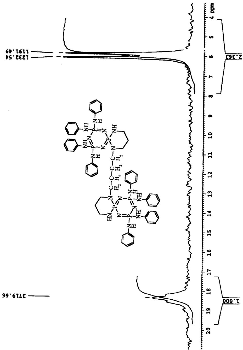
Spektrum 6.39: VIII Numaralı Bileşiğin Proton ile Eyleşenmiş ^{31}\text{P} NMR Spektrumu
