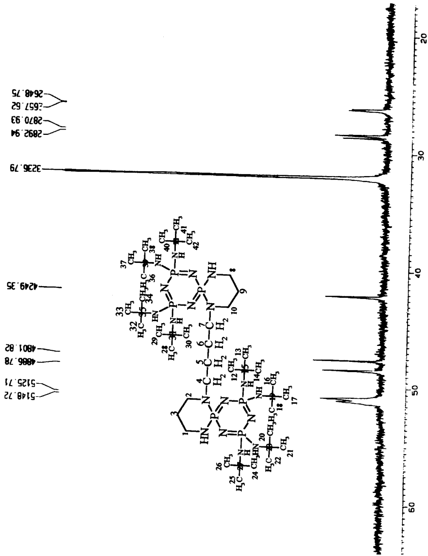
Spektrum 6.36 : VII Numaralı Bileşiğin Proton ile Eşleşmiş 13 C NMR Spektrumu
