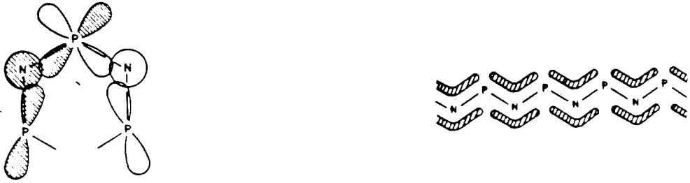
Şekil 2.6. Hekzaklorosiklotrifosfazatrien (Trimer)'deki fosforun d_{xz} ve d_{yz} orbitallerinin azotun p_z orbitali ile örtüşmesi
