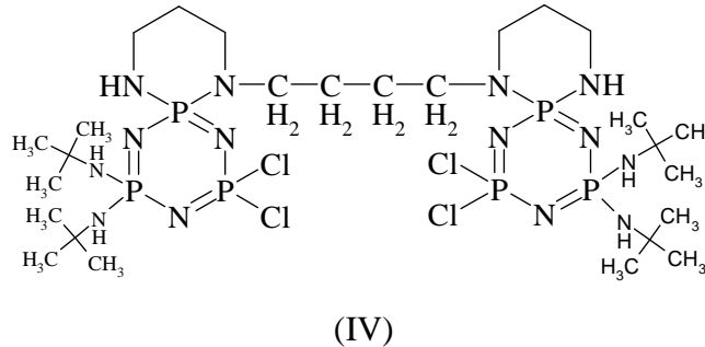
Şekil 6.6. Trimerin SperminTürevi (I) ile t -Butilaminin Reaksiyonu Sonucu Oluşan Ürün
