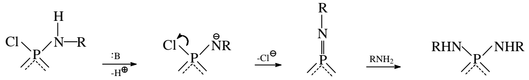
Şekil 2.22. t -butilaminin geminal sübstütüsüonu.
