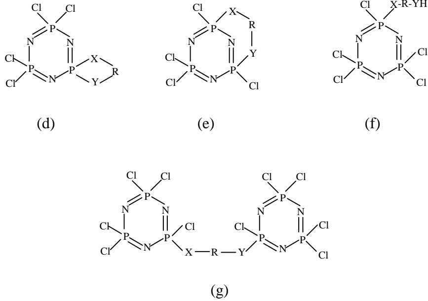
Şekil 2.13. Hekzaklorosiklotrifosfazatrienin (Trimer)'in difonksiyonlu reaktifler ile meydana getirdikleri ürünler
