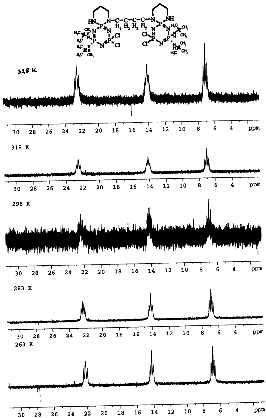
Spektrum 6.24 : IV/1 Numaralı Bileşiğin Değişik Sıcaklıklardaki Proton ile Eşleşmemiş ^{31}\text{P} NMR Spektrumu
