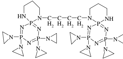
Şekil.2.34. Tetrakis(aziridino)siklotrifosfazatrien Bileşiğinin Spermin Türevi
