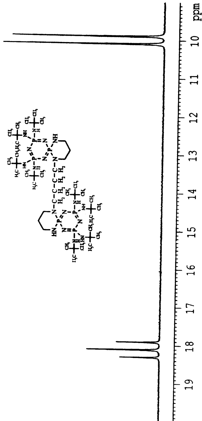
Spektrum 6.35 : VI Numaralı Bileşiğin Proton ile Eşleşmemiş ^{31}\text{P} NMR Spektrumu
