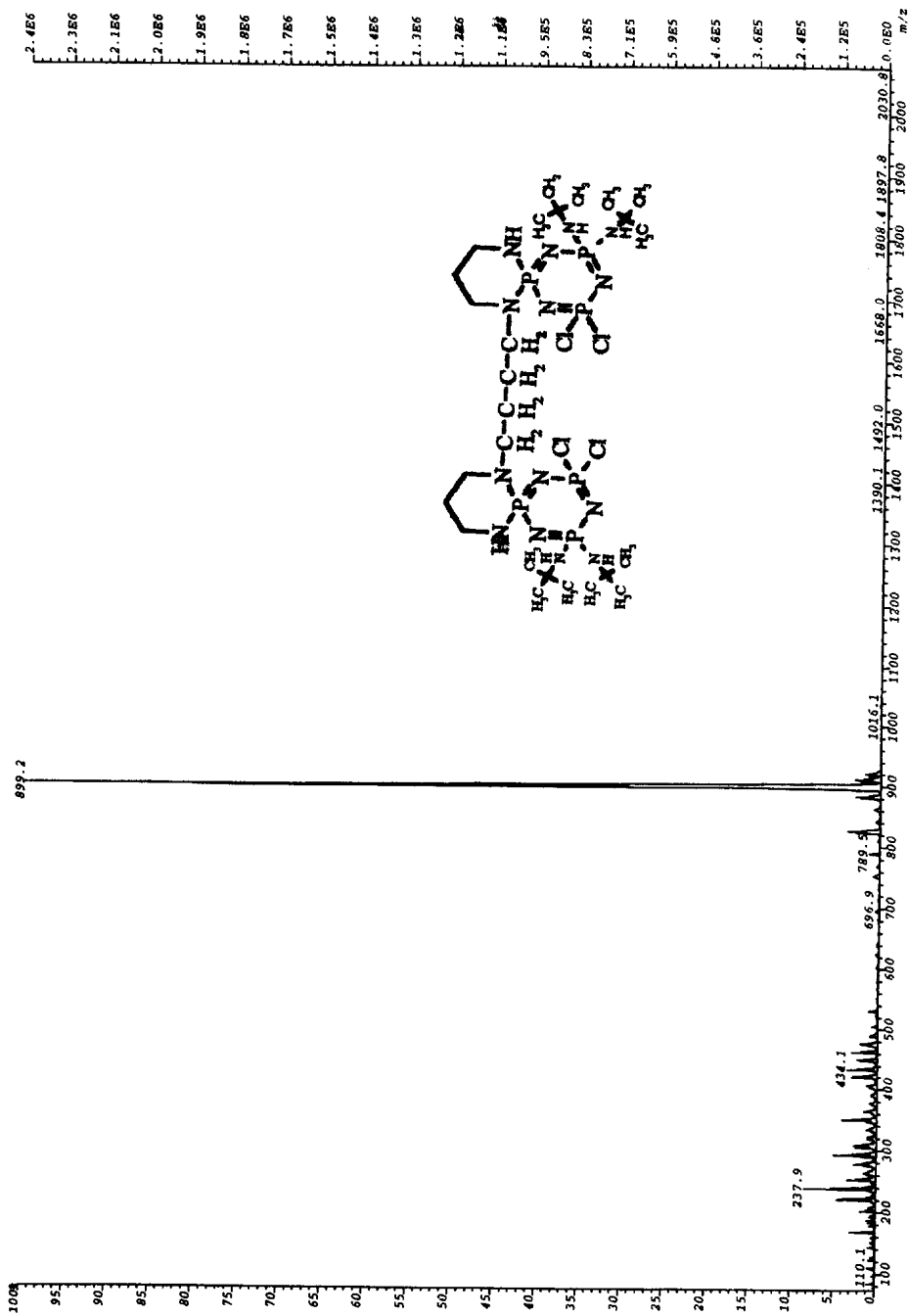
Spektrum 6.19 : IV Numaralı Bileşiğin Kütle Spektrumu
