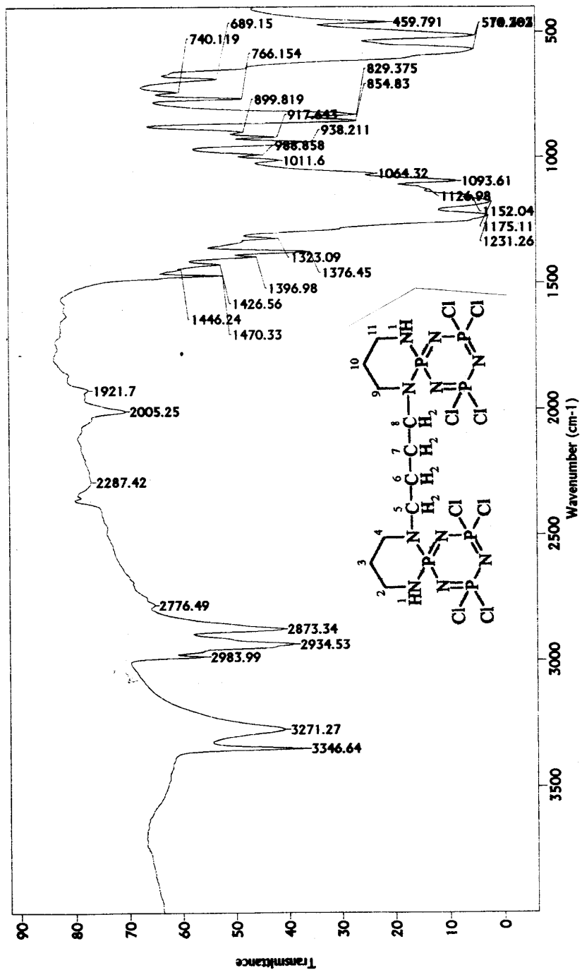
Spektrum 6.1 : I Numaralı Bileşiğin FT-IR Spektrumu
