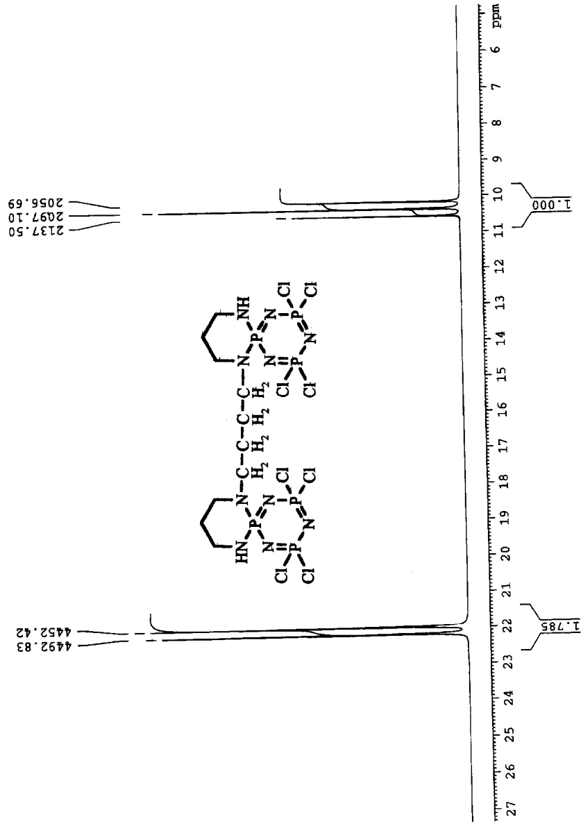
Spektrum 6.3 : I Numaralı Bileşğin Proton ile Eşleşmemiş ^{31}\text{P} NMR Spektrumu
