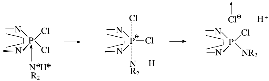
Şekil 2.20. S_N^2 bimoleküler reaksiyon tipi.
