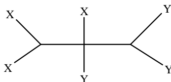
Şekil 2.15. Hekzaklorosiklotrifosfazatrien (Trimer)’in Geminal Trisübstitüe Bileşikleri
