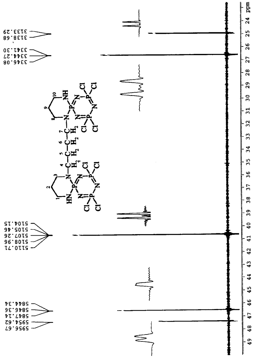
Spektrum 6.6 : I Numaralı Bileşimin Proton ile Eşleşmemiş Fosfor ile Eşleşmiş ^{13}\text{C} NMR Spektrumu
