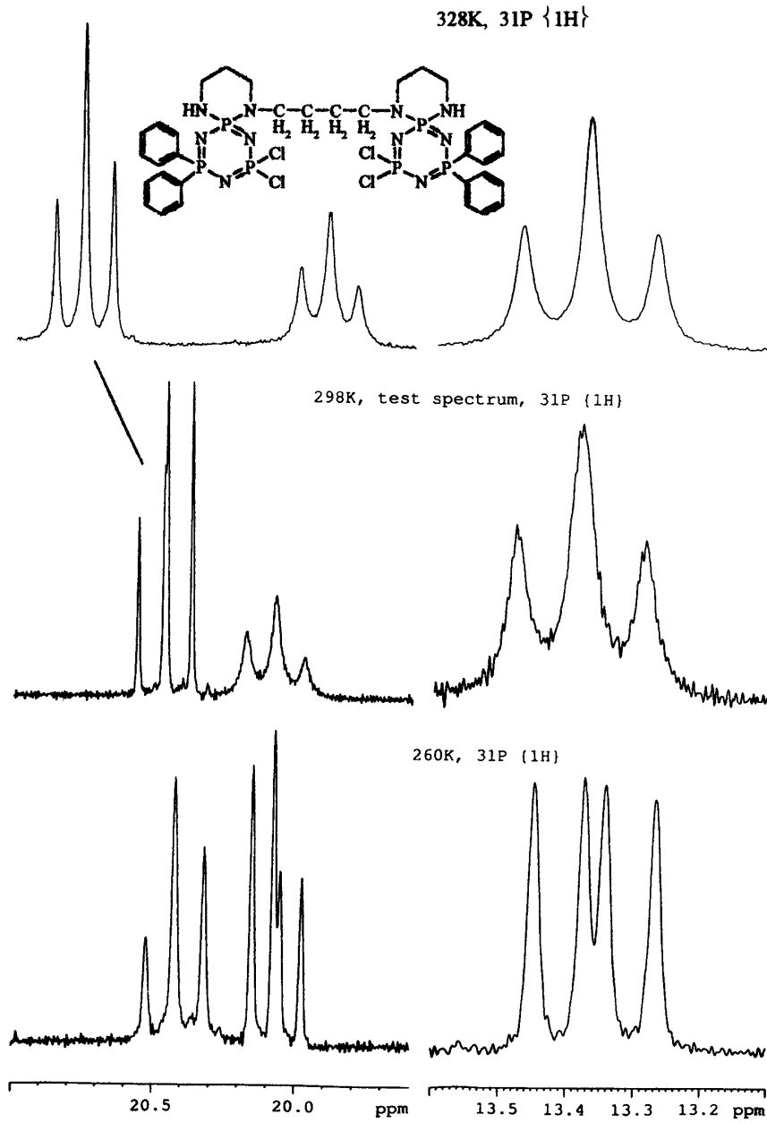
Spektrum 6.16 : III/1 Numaralı Bileşimin Değişik Sıcaklıklardaki Proton ile Eşleşmiş ^{31}\text{P} NMR Spektrumu
