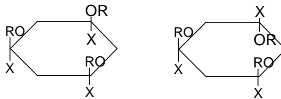
Şekil 2.25. Hekzaklorosiklotrifosfazatriende non-geminal sübtitüsyonla cis - ve trans izomerlerin oluşumu.
