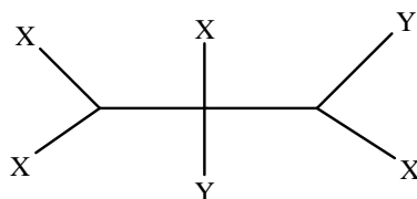
Şekil 2.16. Geminal olmayan trans-di ve tetra sübstitüe türevleri
