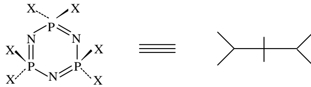
Şekil 2.8. Trimerin genel olarak gösterilişi.
