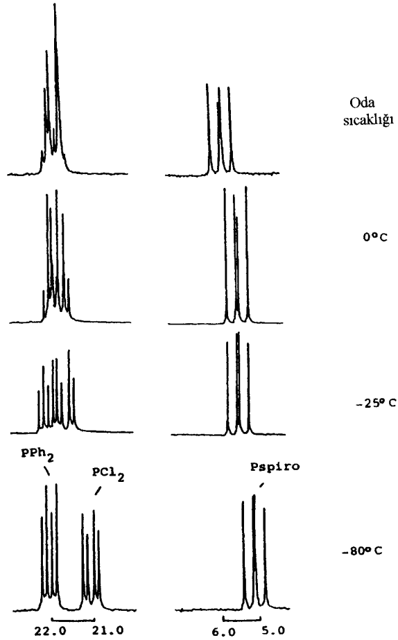
Şekil 3.3. \text{N}_3\text{P}_3\text{Ph}_2[\text{O}(\text{CH}_2)_3\text{O}]\text{Cl}_2 bileşiğinin değişik sıcaklıklardaki ^{31}\text{P} NMR’ı
