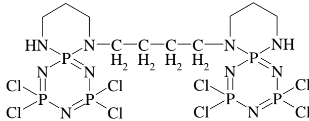
Şekil 6.1. Trimerin spermin türevi (I)
