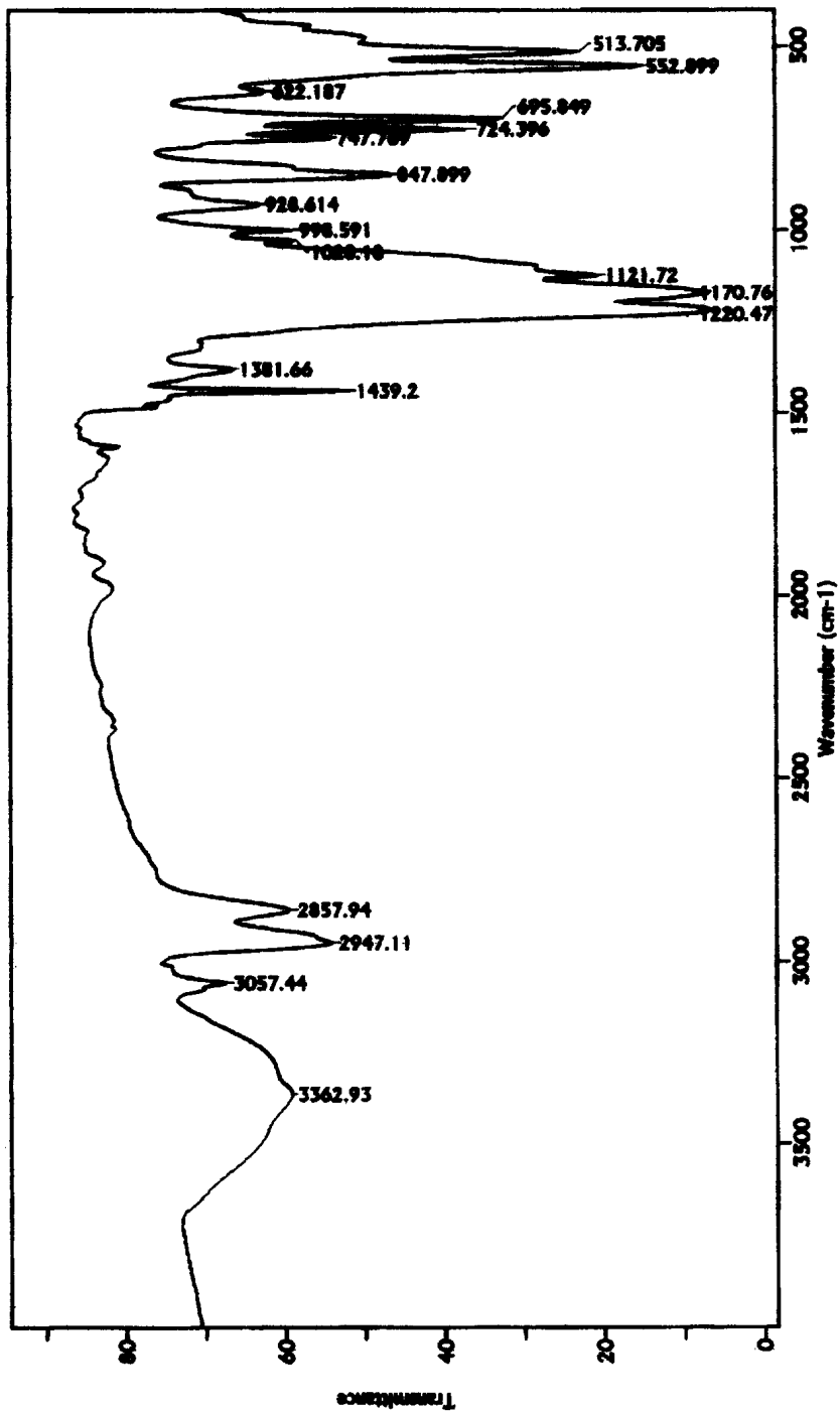
Spektrum 6.9 : III Numaralı Bileşğin FT-IR Spektrumu
