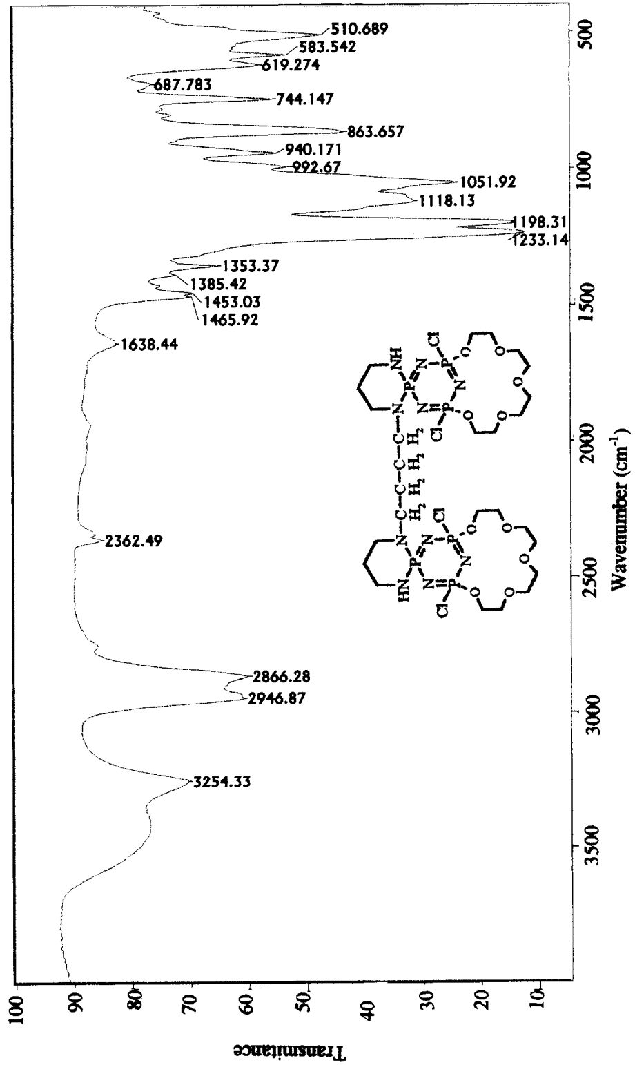
Spektrum 6.26: V Numaralı Bileşiğin FT-IR Spektrumu
