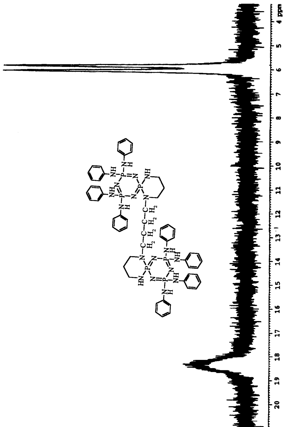
Spektrum 6.40 : VIII Numaralı Bileşiğin Proton ile Eylemiş ^{31}\text{P} NMR Spektrumu
