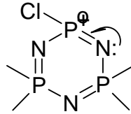
Şekil 2.30. Azotun çiftlenmemiş elektronlarının etkisi
