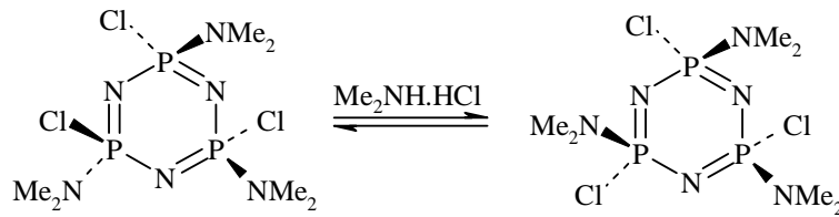
Şekil 2.14. Geminal olmayan N_3P_3Cl_3(NMe_2)_3 bileşiğinin cis -, trans - izomerliği
