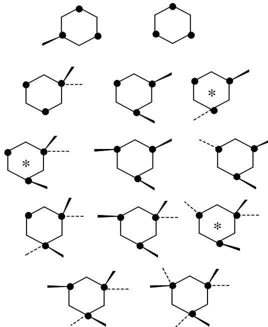
Şekil 2.10. Hekzaklorosiklotrifosfazatrienin (Trimer) Stereokimyası
