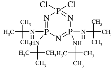
Şekil 6.10. Trimer ile t-bütilamin Reaksiyonu Sonucu Oluşan Ürün
