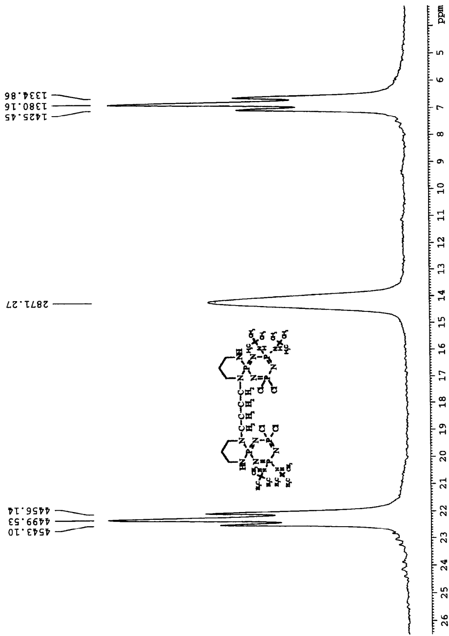
Spektrum 6.21 : IV/1 Numaralı Bileşimin Proton ile Eşleşmiş ^{31}\text{P} NMR Spektrumu
