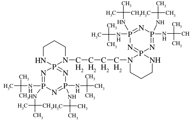
Şekil 6.11. Spermin ile 2,2-dikloro-4,4,6,6-tetra-t-butilaminosiklotrifosfazatrien Reaksiyonu Sonucu Oluşan Ürün
