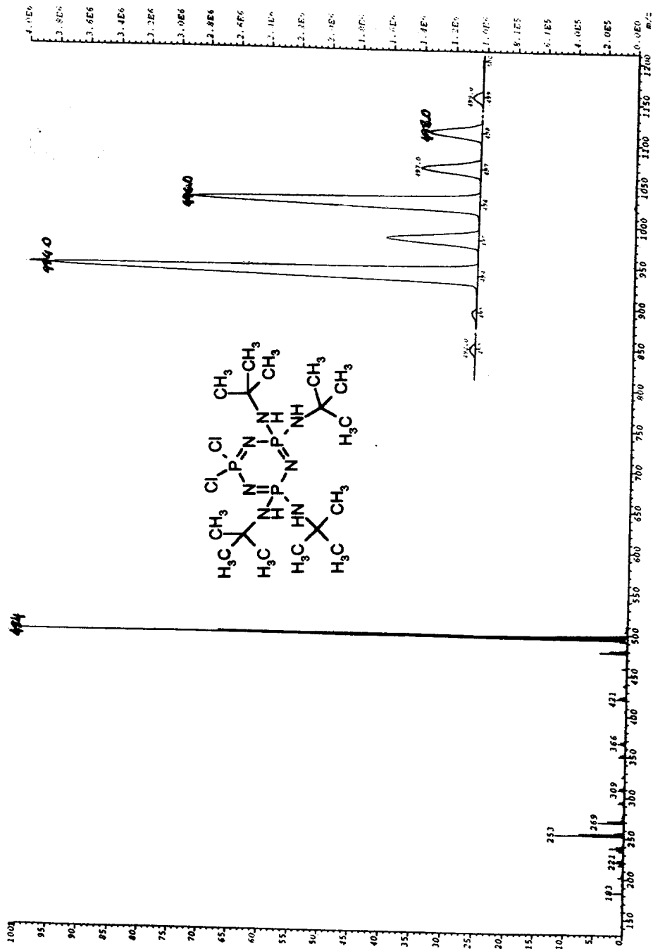
Spektrum 6.32 : VI Numaralı Bileşiğin Kütle Spektrumu
