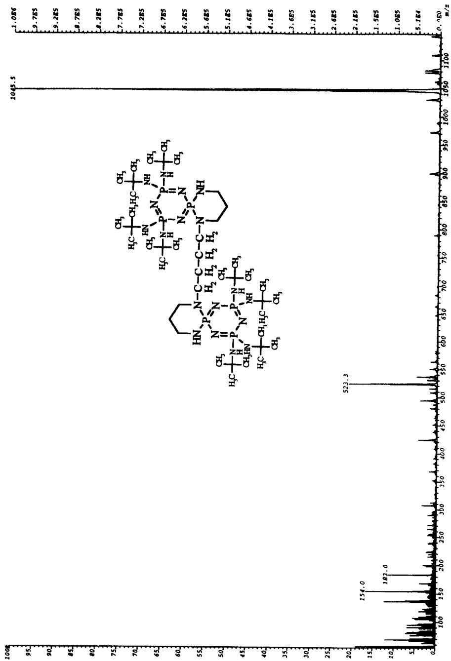
Spektrum 6.34 : VII Numaralı Bileşimin Kütle Spektrumu
