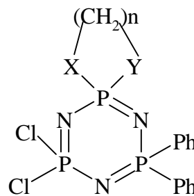
Şekil. 3.2. gem- \text{N}_3\text{P}_3\text{Ph}_2\text{Cl}_4 bileşiğinin monospiro türevleri
