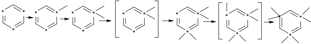
Şekil 3.1. t-butilaminosiklotrifosfazatrienler için reaksiyon şeması
