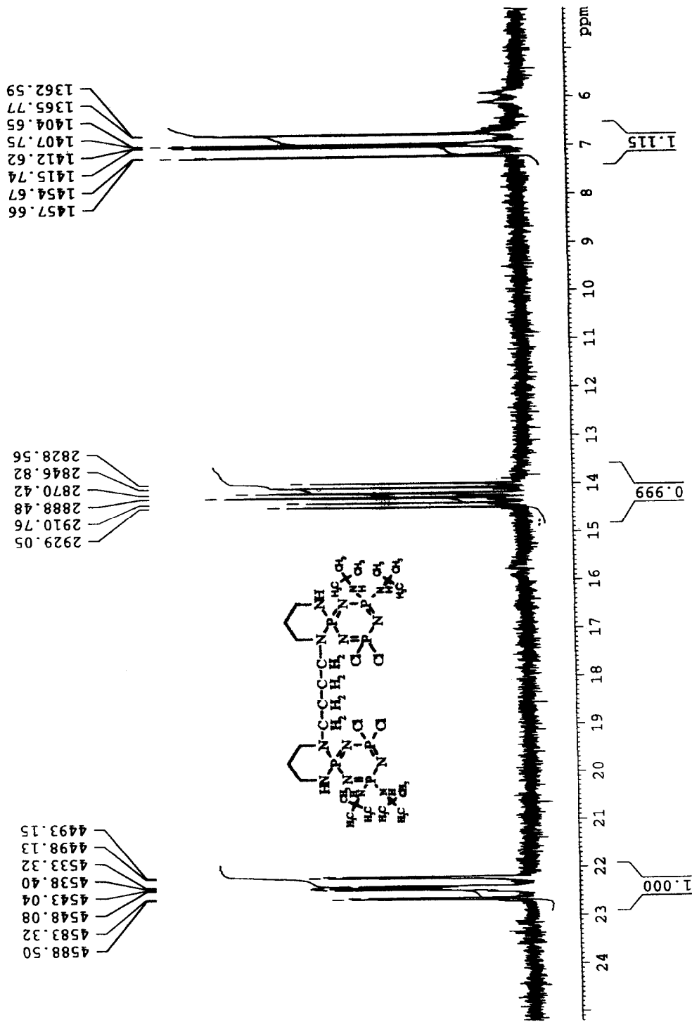
Spektrum 6.17 : IV Numaralı Bileşğin Reaksiyon Karışımının Proton ile Eşleşmemiş ^{31}\text{P} NMR Spektrumu
