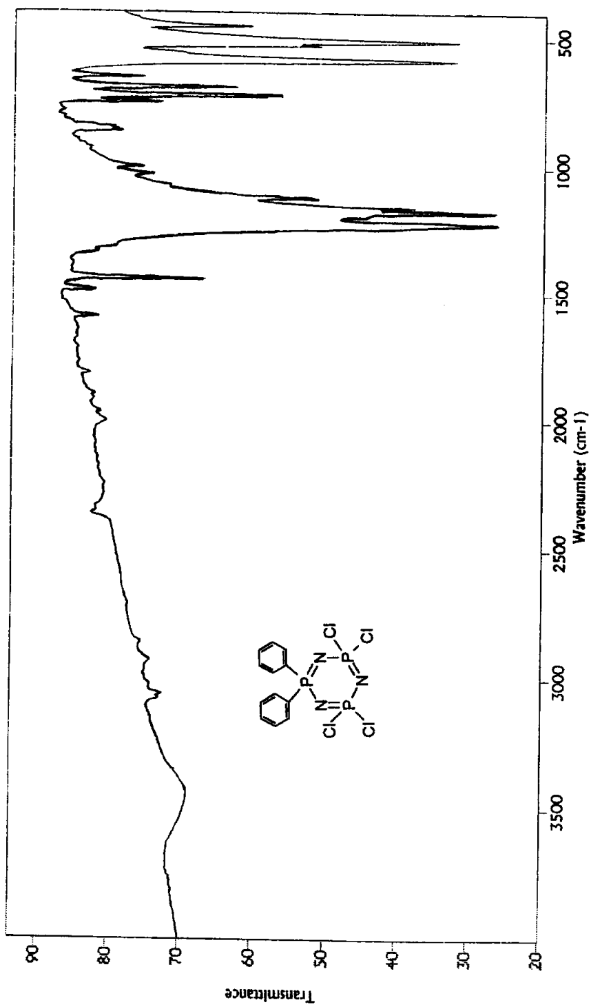
Spektrum 6.8 : II Numaralı Bileşiğin FT-IR Spektrumu
