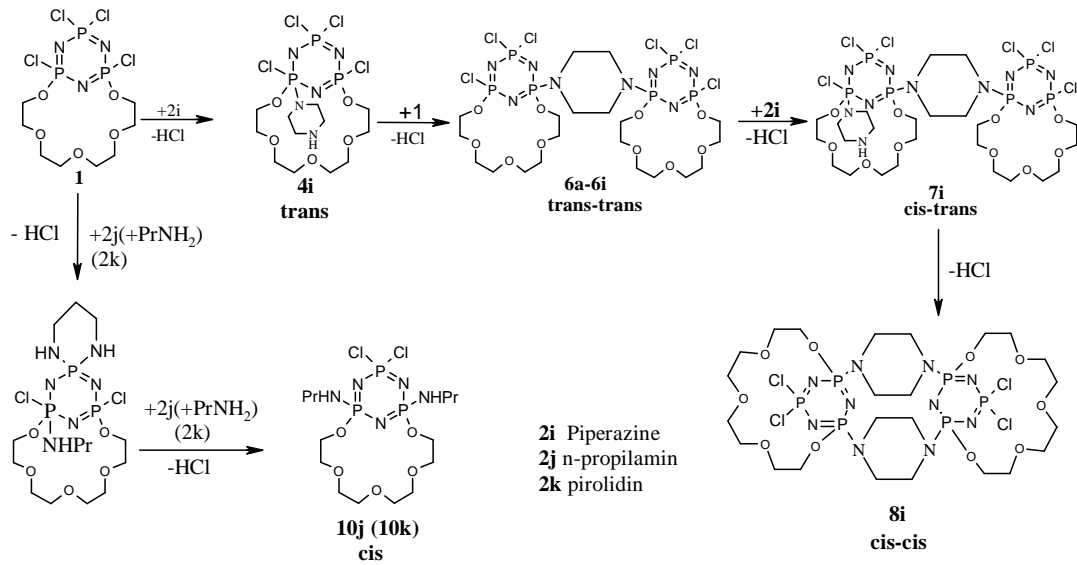
Şekil 2.18. Piperazin türevi makrosiklik fosfazen bileşikleri
