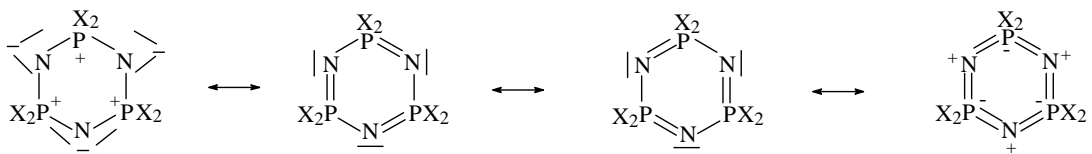
Şekil 2.9. Trimerin rezonans yapılarının toplamı
