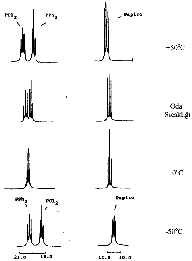
Şekil 3.4. N_3P_3Ph_2[HN(CH_2)_3NH]Cl_2 bileşiginin değişik sıcaklıklardaki ^{31}P NMR'ı
