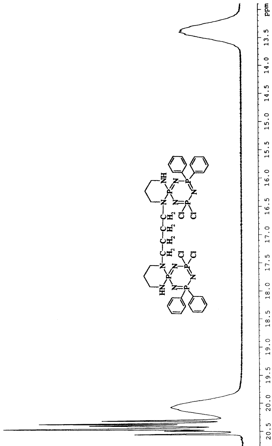
Spektrum 6.13 : III Numaralı Bileşimin Proton ile Eşleşmiş ^{31}\text{P} NMR Spektrumu
