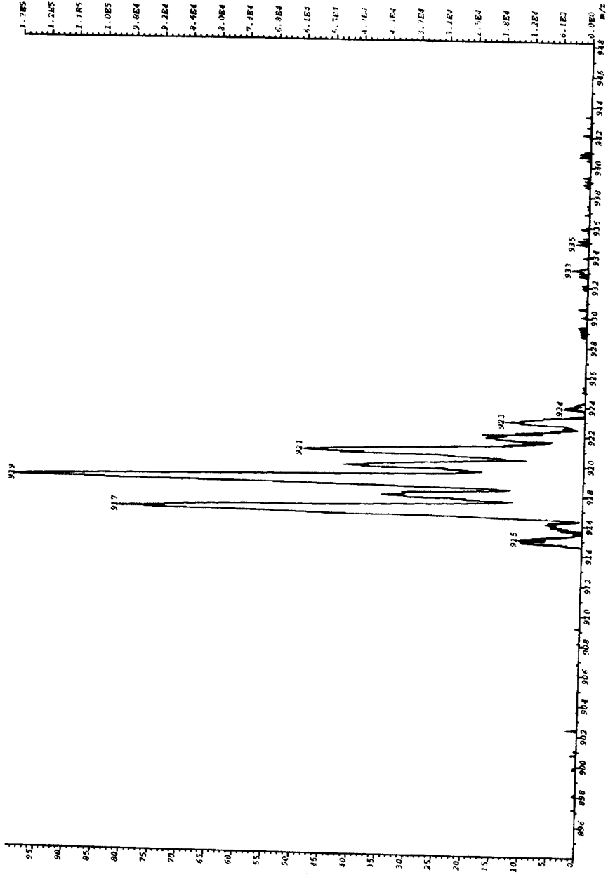
Spektrum 6.11: III Numaralı Bileşğin Mol Pikinin Genişletilmiş Hali
