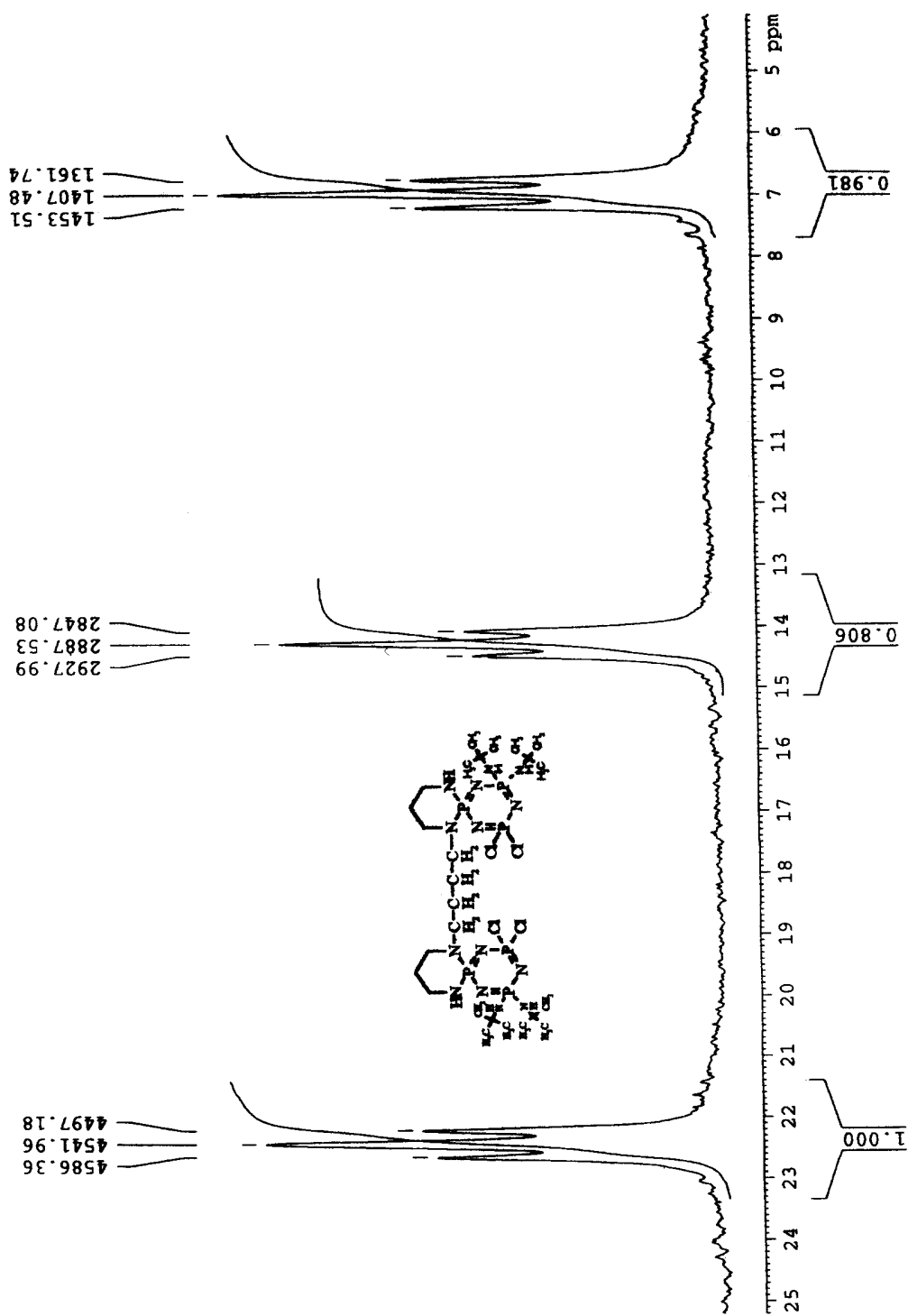
Spektrum 6.25 : IV/2 Numaralı Bileşiğin Proton ile Eşleşmemiş ^{31}\text{P} NMR Spektrumu
