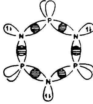
Şekil 2.3. Hekzaklorosiklotrifosfazatrien (Trimer)'in \delta -bağı iskelet yapısı
