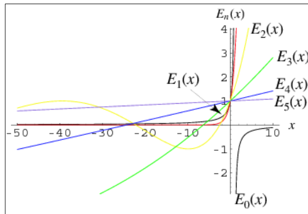
Şekil 2.2: Mittag-Leffler Fonksiyonu.
