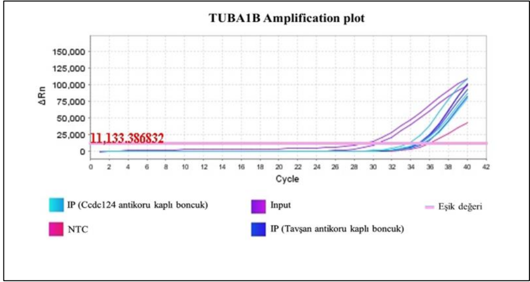
Şekil 5.16: Ccdc124 proteininin olası bir RNA hedefi olarak TUBA1B'ye ait amplifikasyon grafiği.
