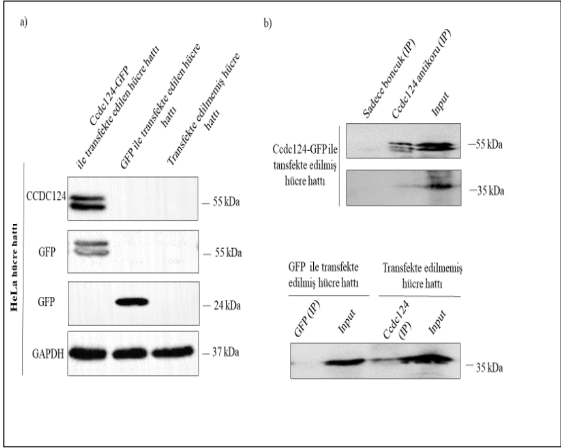
Şekil 5.6: Sekanslama öncesinde yapılan kontrollere ait western blot sonuçları. a) Transfekte edilmemiş, GFP plazmidıyla ve Cdc124 ile transfekte edilmiş hücre hatalarına ait western blot sonuçları. b) RNA ile çöktürme deneyi sırasında kullanılan boncukların Cdc124 bağlama kapasitelerinin kontrolüne ait western sonuçları.
