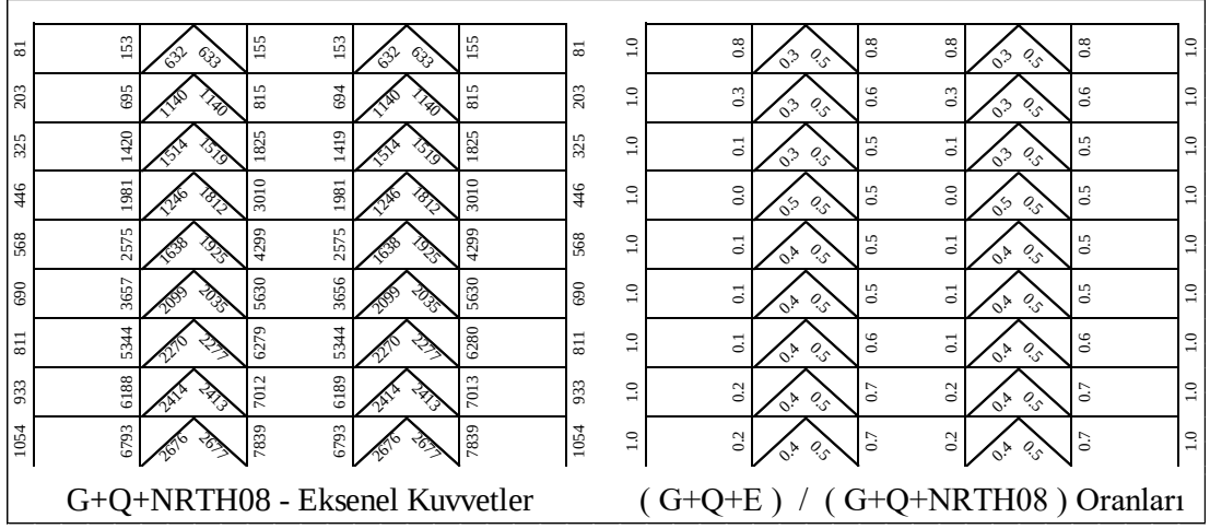
Şekil 5.135 : 9 Katlı Çerçevenin G+Q+E /G+Q+NRTH (SF=0.8) Oranları.
