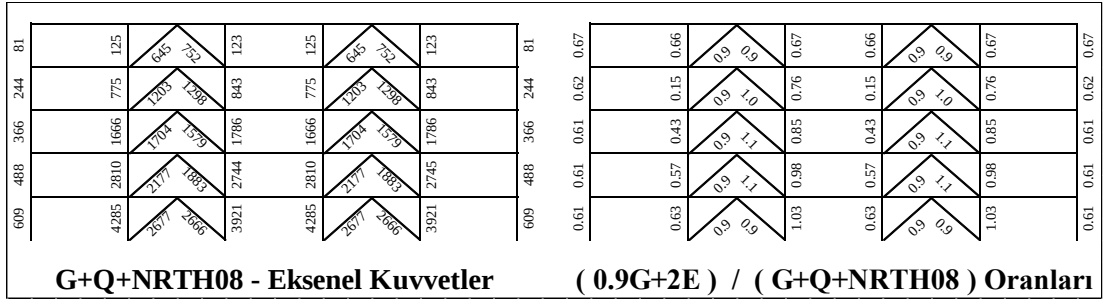
Şekil 5.84 : 5 Katlı Çerçevenin 0.9G+2E /G+Q+NRTH (SF=0.8) Oranları.
