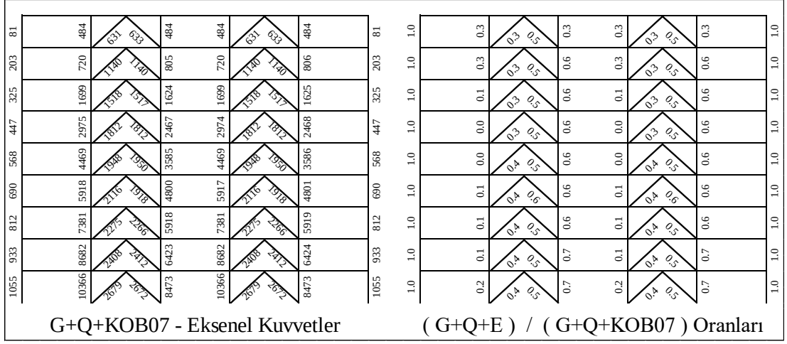
Şekil 5.126 : 9 Katlı Çerçevenin G+Q+E /G+Q+KOB (SF=0.7) Oranları.
