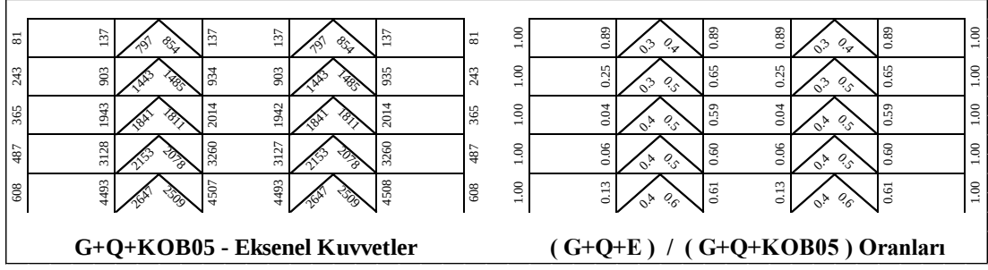
Şekil 5.50 : 5 Katlı Çerçevenin G+Q+E /G+Q+KOB (SF=0.5) Oranları.
