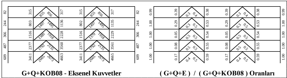
Şekil 5.52 : 5 Katlı Çerçevenin G+Q+E /G+Q+KOB (SF=0.8) Oranları.
