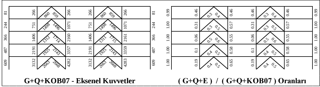
Şekil 5.51 : 5 Katlı Çerçevenin G+Q+E /G+Q+KOB (SF=0.7) Oranları.
