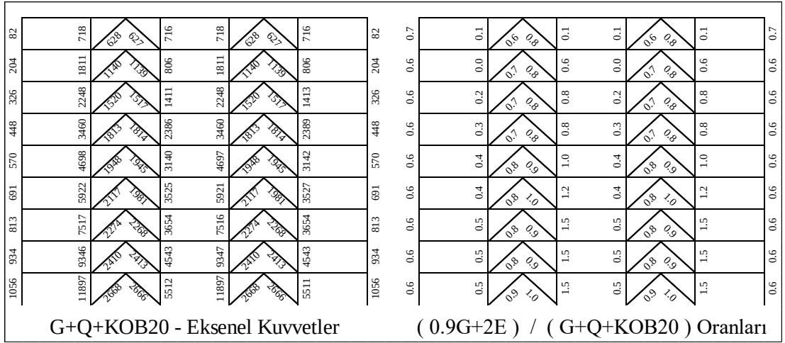
Şekil 5.154 : 9 Katlı Çerçevenin 0.9G+2E /G+Q+KOB (SF=2.0) Oranları.
