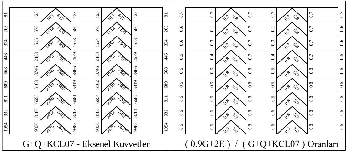
Şekil 5.142 : 9 Katlı Çerçevenin 0.9G+2E /G+Q+KCL (SF=0.7) Oranları.
