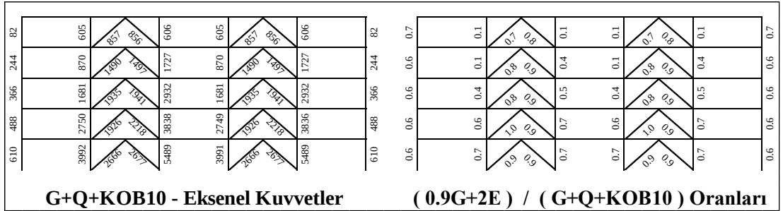
Şekil 5.77 : 5 Katlı Çerçevenin 0.9G+2E /G+Q+KOB (SF=1.0) Oranları.
