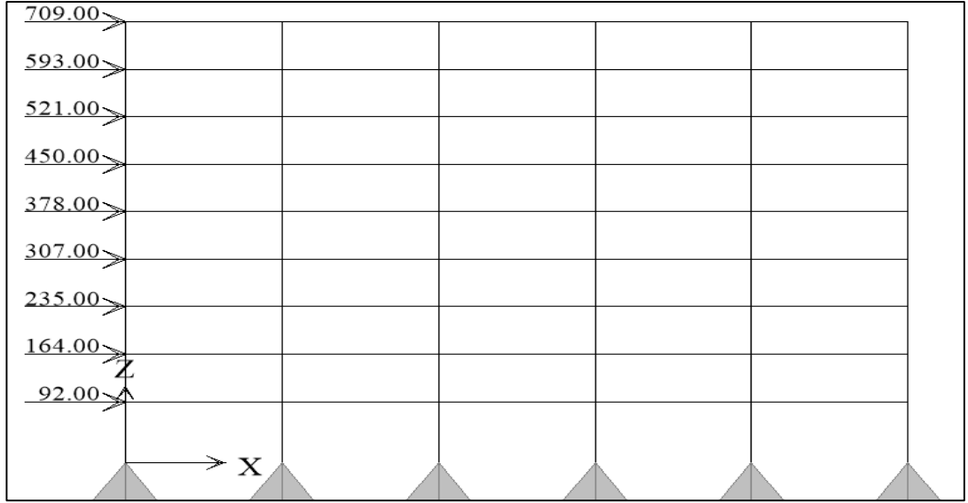
Şekil 5.7 : 9 Katlı Çerçeve İçin SAP2000 Deprem Yükleme.
