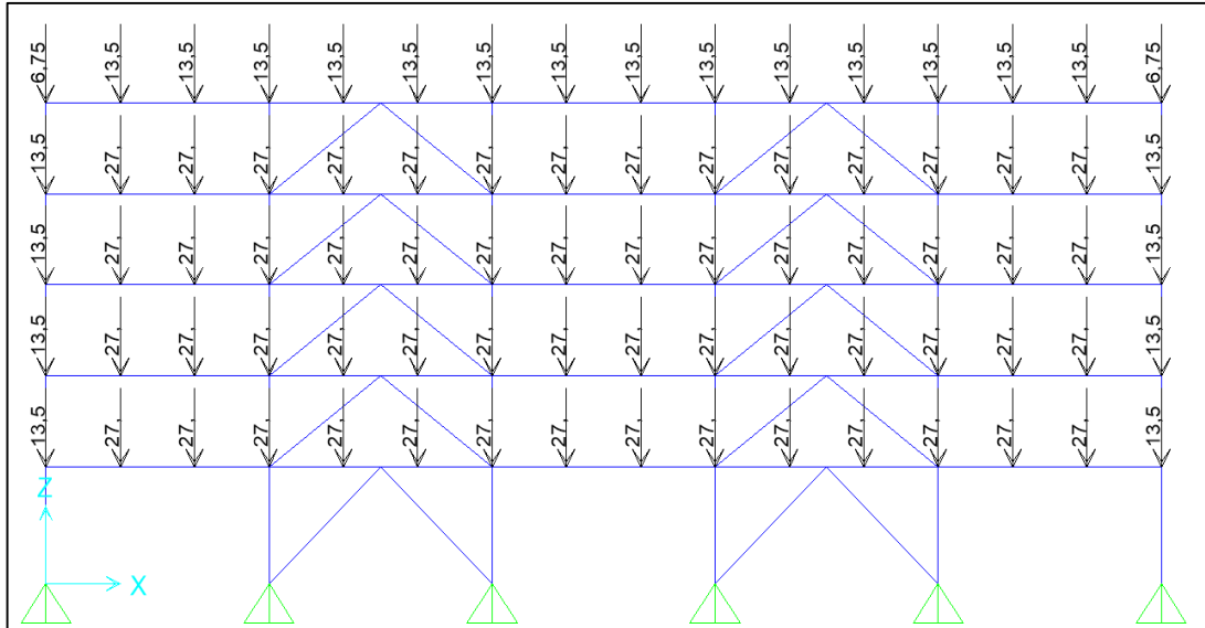
Şekil 5.4 : 5 Katlı Çerçeve LL Yükleme.
