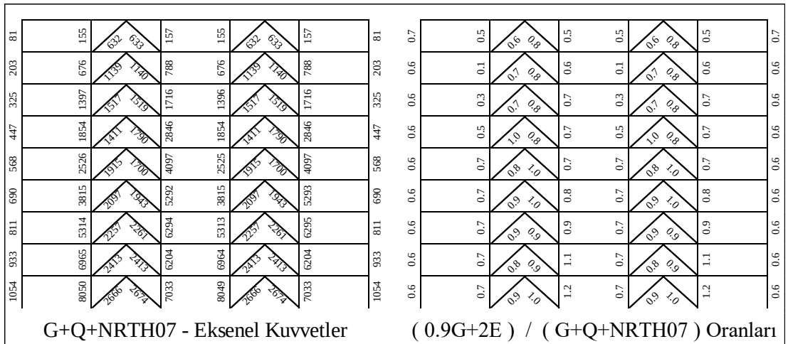
Şekil 5.158 : 9 Katlı Çerçevenin 0.9G+2E /G+Q+NRTH (SF=0.7) Oranları.
