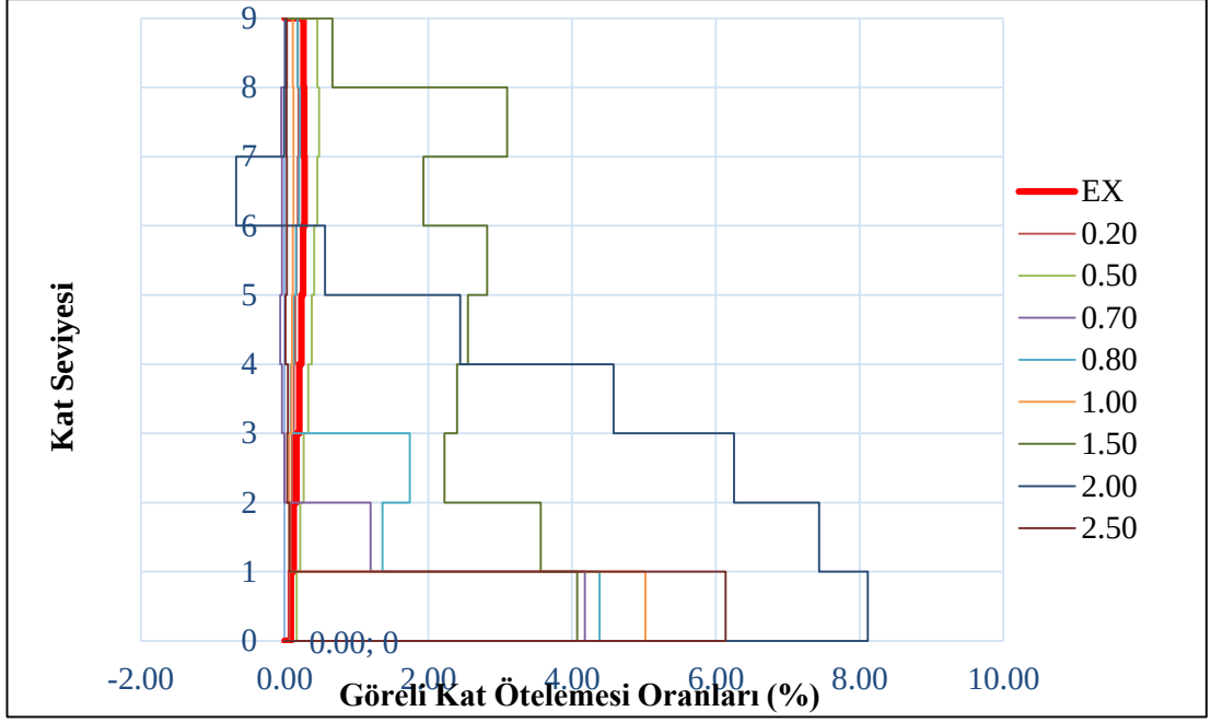
Şekil 5.23 : 9 Katlı Bina için Kocaeli Depremi Görel Kat Öteleme Oranları.
