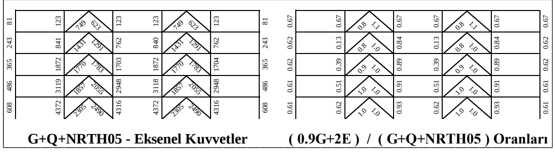
Şekil 5.82 : 5 Katlı Çerçevenin 0.9G+2E /G+Q+NRTH (SF=0.5) Oranları.
