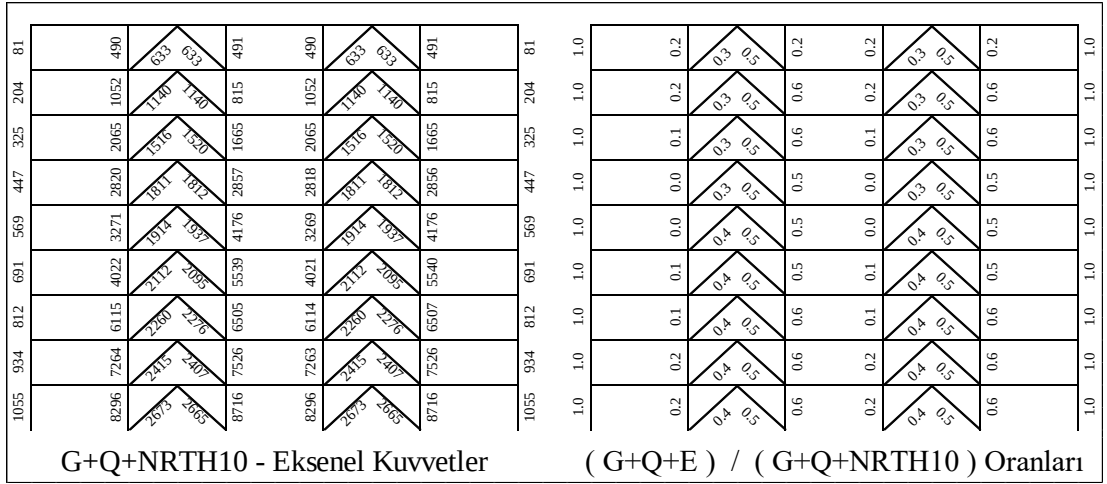
Şekil 5.136 : 9 Katlı Çerçevenin G+Q+E /G+Q+NRTH (SF=1.0) Oranları.
