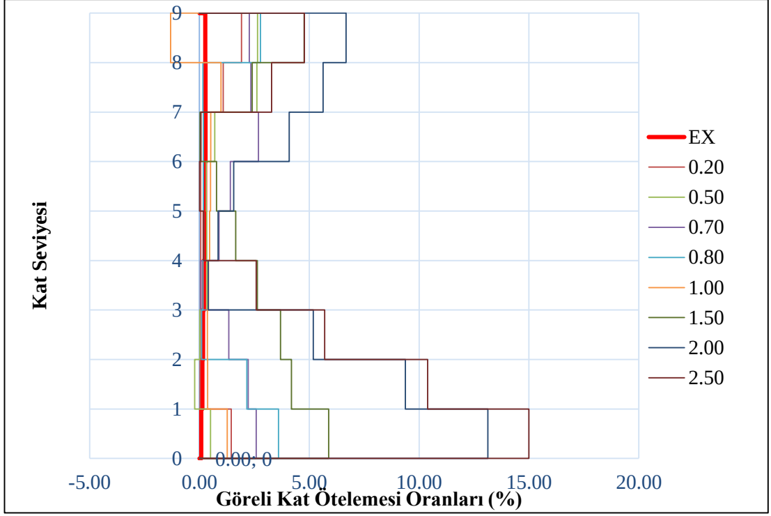
Şekil 5.25 : 9 Katlı Bina için Kobe Depremi Görel Kat Öteleme Oranları.
