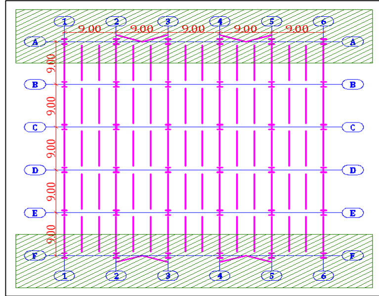
Şekil 5.1 : Çaprazlı Çerçevelerde Ana Kirişlere Gelen Düşey Yük Alanları.
