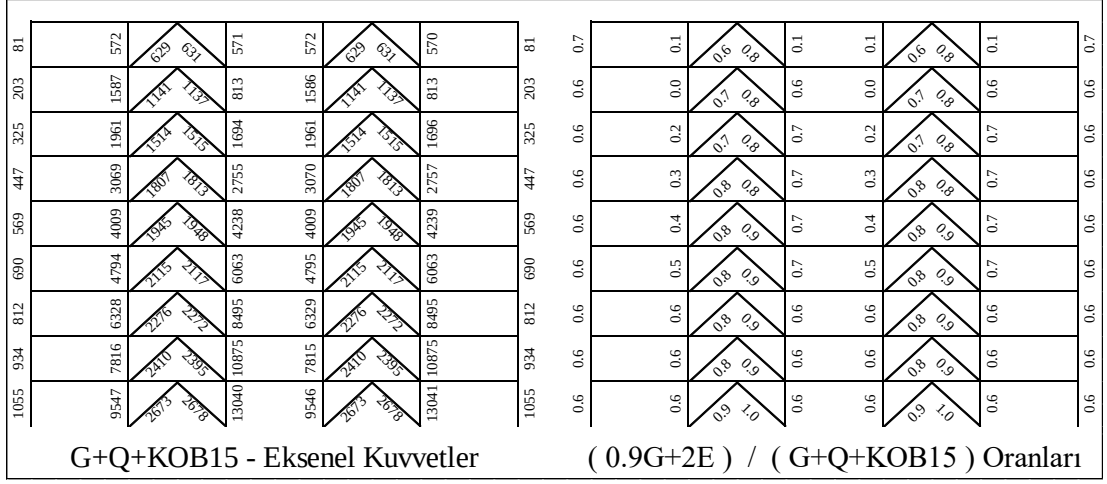
Şekil 5.153 : 9 Katlı Çerçevenin 0.9G+2E /G+Q+KOB (SF=1.5) Oranları.
