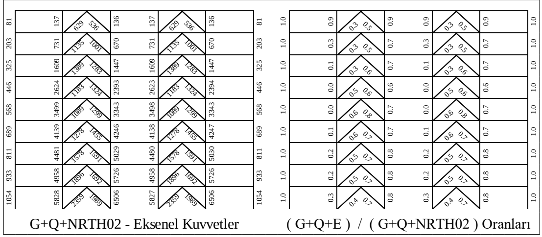
Şekil 5.132 : 9 Katlı Çerçevenin G+Q+E /G+Q+NRTH (SF=0.2) Oranları.
