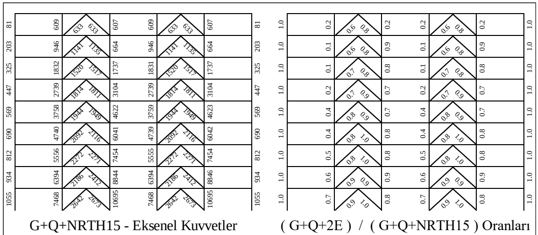
Şekil 5.185 : 9 Katlı Çerçevenin G+Q+2E /G+Q+NRTH (SF=1.5) Oranları.
