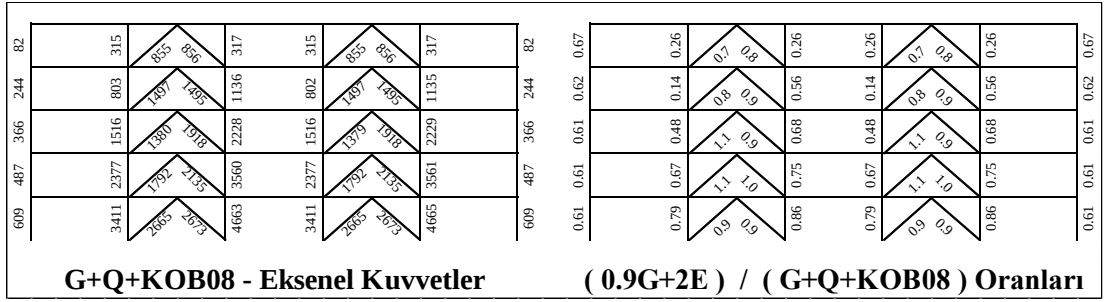
Şekil 5.76 : 5 Katlı Çerçevenin 0.9G+2E /G+Q+KOB (SF=0.8) Oranları.
