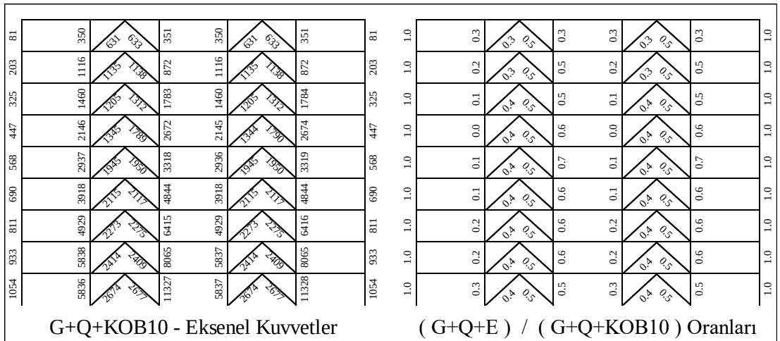
Şekil 5.128 : 9 Katlı Çerçevenin G+Q+E /G+Q+KOB (SF=1.0) Oranları.
