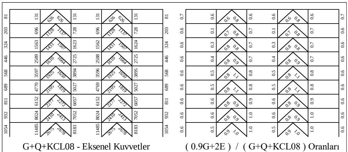
Şekil 5.143 : 9 Katlı Çerçevenin 0.9G+2E /G+Q+KCL (SF=0.8) Oranları.
