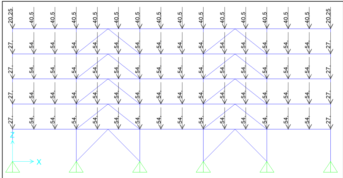
Şekil 5.2 : 5 Katlı Çerçeve DL Yükleme.
