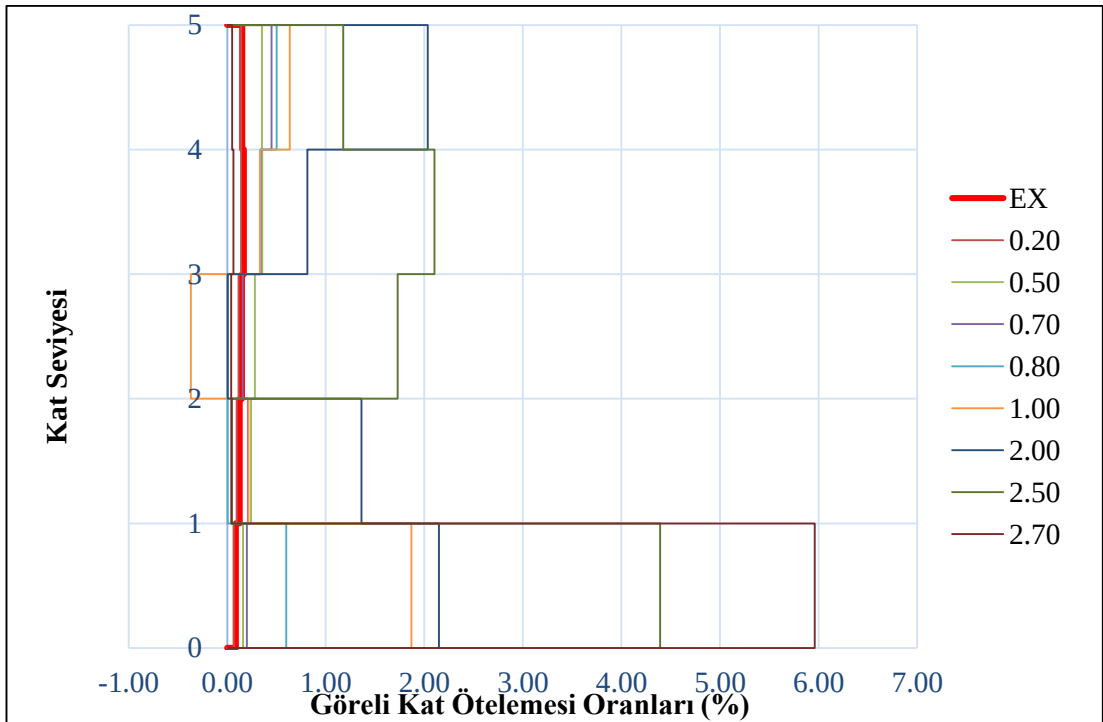
Şekil 5.22 : 5 Katlı Bina için Kobe Depremi Görelî Kat Öteleme Oranları.
