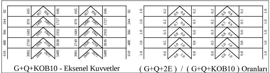
Şekil 5.101 : 5 Katlı Çerçevenin G+Q+2E /G+Q+KOB (SF=1.0) Oranları.
