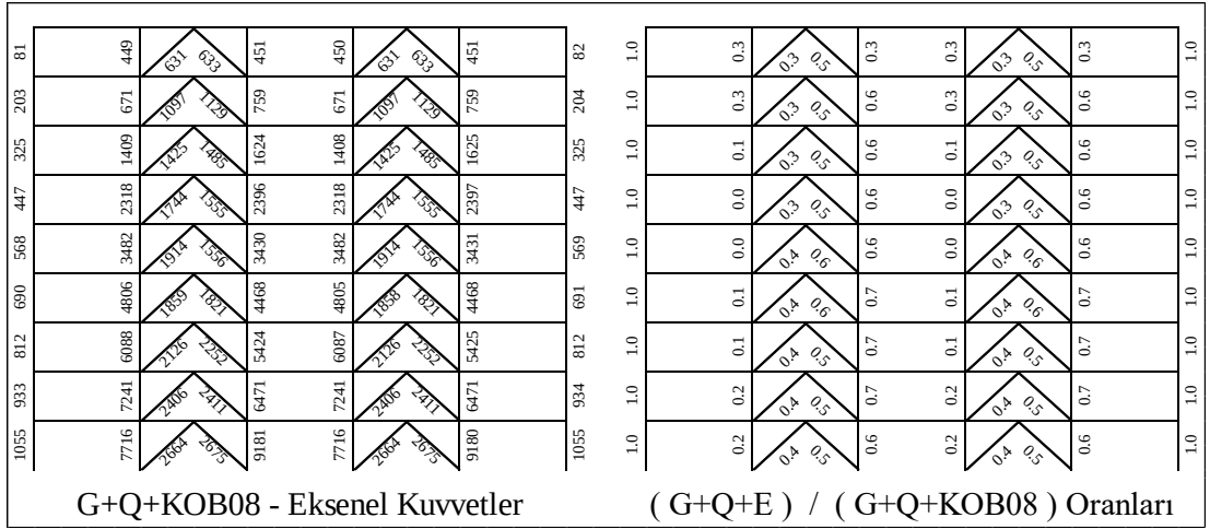
Şekil 5.127 : 9 Katlı Çerçevenin G+Q+E /G+Q+KOB (SF=0.8) Oranları.
