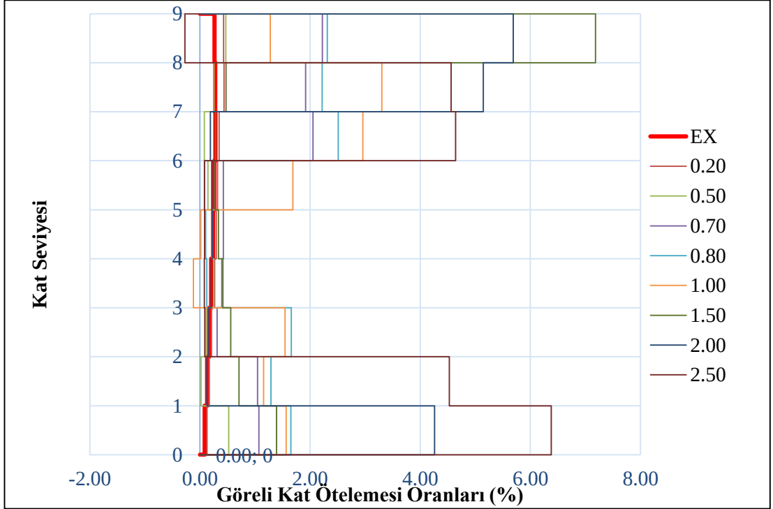
Şekil 5.24 : 9 Katlı Bina için Northridge Depremi Görel Kat Öteleme Oranları.
