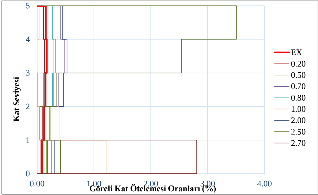
Şekil 5.21 : 5 Katlı Bina için Northridge Depremi Görelî Kat Öteleme Oranları.
