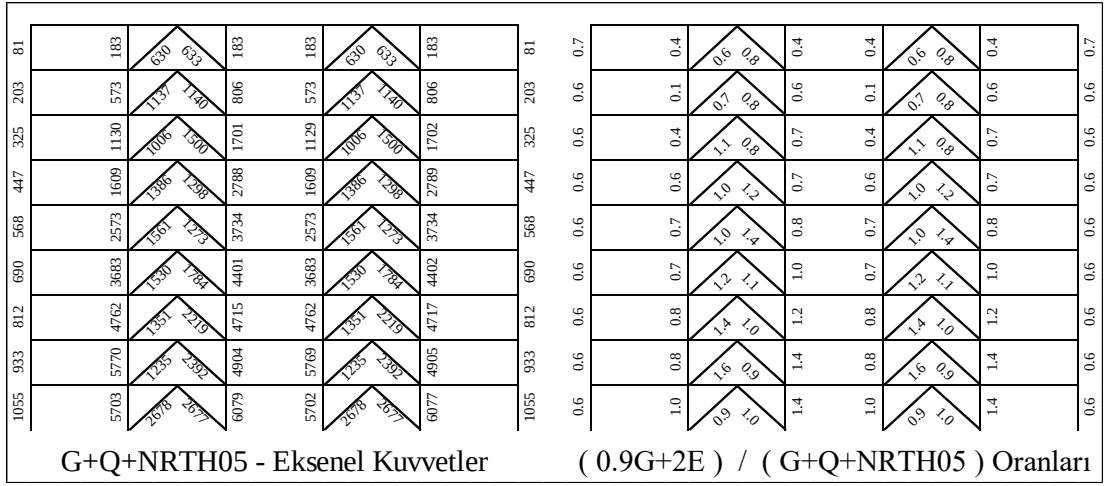
Şekil 5.157 : 9 Katlı Çerçevenin 0.9G+2E /G+Q+NRTH (SF=0.5) Oranları.
