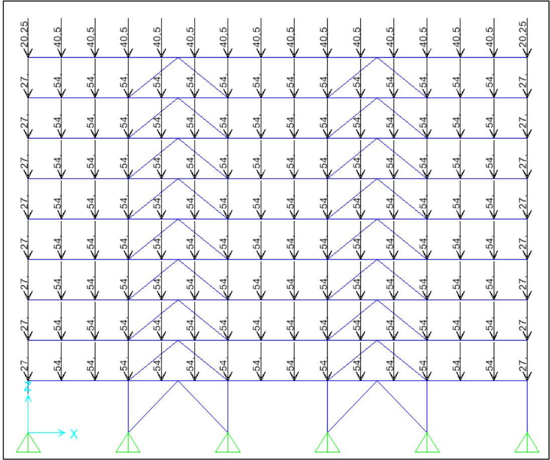
Şekil 5.3 : 9 Katlı Çerçeve DL Yükleme.
