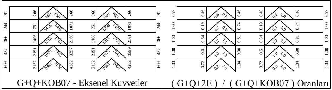
Şekil 5.99 : 5 Katlı Çerçevenin G+Q+2E /G+Q+KOB (SF=0.7) Oranları.
