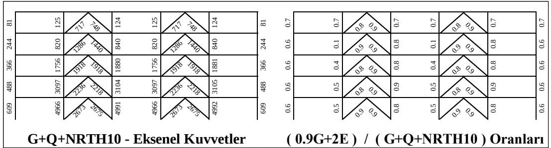
Şekil 5.85 : 5 Katlı Çerçevenin 0.9G+2E /G+Q+NRTH (SF=1.0) Oranları.
