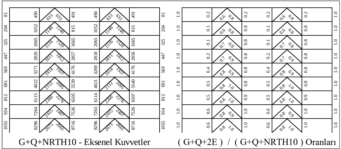
Şekil 5.184 : 9 Katlı Çerçevenin G+Q+2E /G+Q+NRTH (SF=1.0) Oranları.
