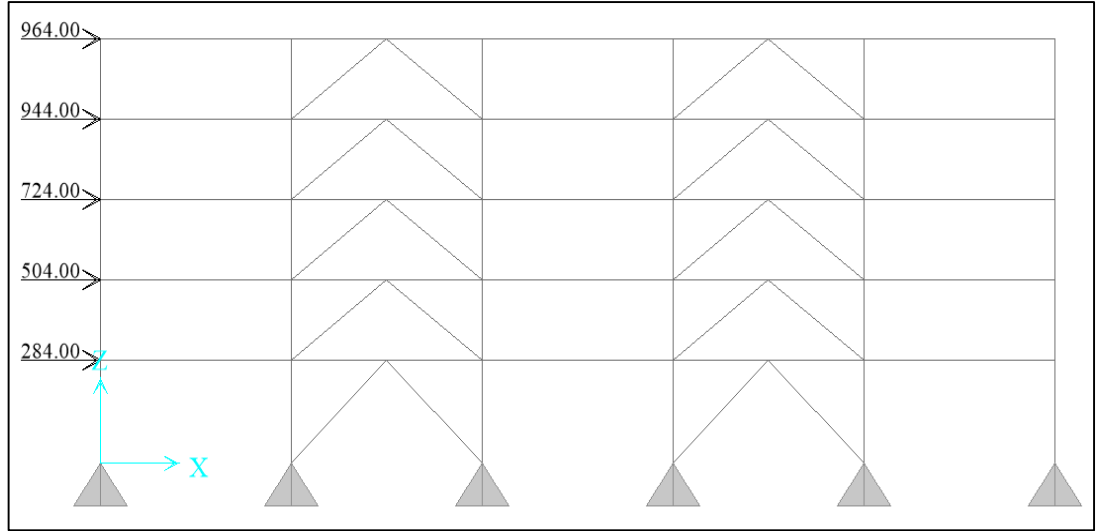
Şekil 5.6 : 5 Katlı Çerçeve İçin SAP2000 Deprem Yükleme.
