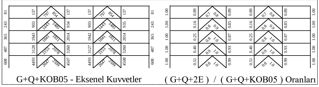
Şekil 5.98 : 5 Katlı Çerçevenin G+Q+2E /G+Q+KOB (SF=0.5) Oranları.
