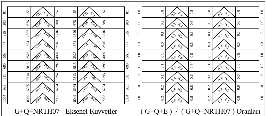
Şekil 5.134 : 9 Katlı Çerçevenin G+Q+E /G+Q+NRTH (SF=0.7) Oranları.
