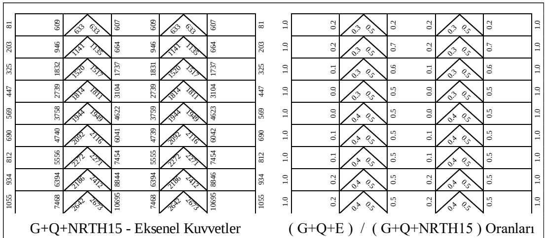
Şekil 5.137 : 9 Katlı Çerçevenin G+Q+E /G+Q+NRTH (SF=1.5) Oranları.
