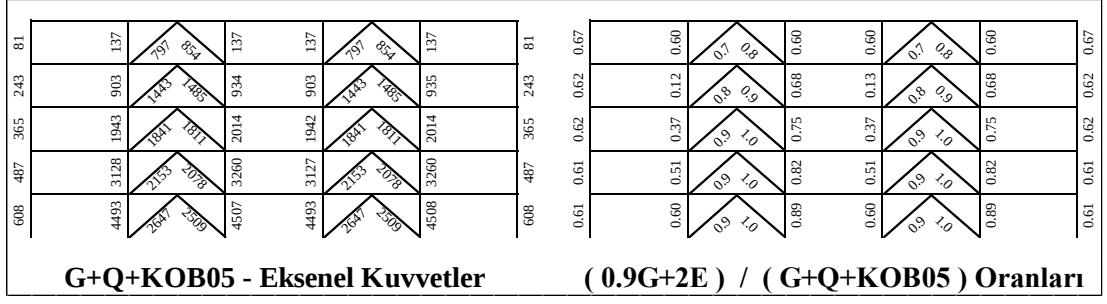
Şekil 5.74 : 5 Katlı Çerçevenin 0.9G+2E /G+Q+KOB (SF=0.5) Oranları.
