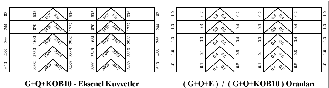
Şekil 5.53 : 5 Katlı Çerçevenin G+Q+E /G+Q+KOB (SF=1.0) Oranları.
