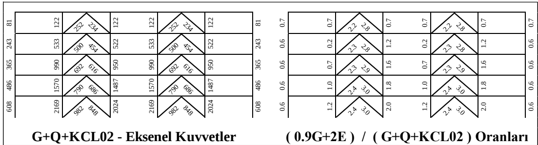
Şekil 5.65 : 5 Katlı Çerçevenin 0.9G+2E /G+Q+KCL (SF=0.2) Oranları.
