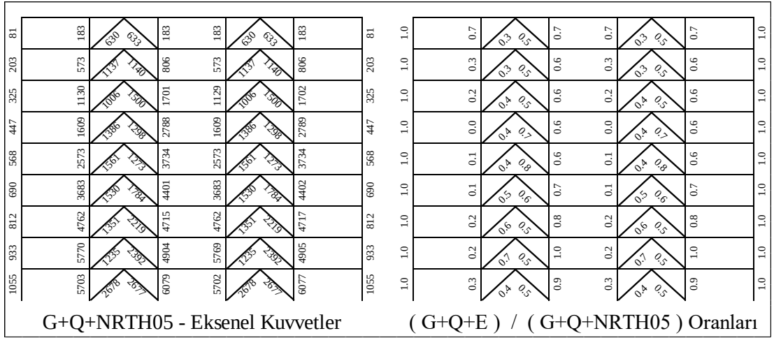
Şekil 5.133 : 9 Katlı Çerçevenin G+Q+E /G+Q+NRTH (SF=0.5) Oranları.
