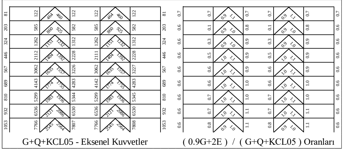
Şekil 5.141 : 9 Katlı Çerçevenin 0.9G+2E /G+Q+KCL (SF=0.5) Oranları.
