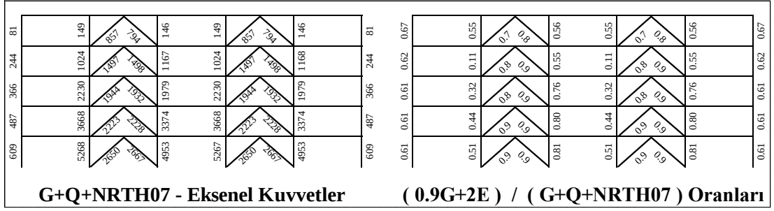
Şekil 5.83 : 5 Katlı Çerçevenin 0.9G+2E /G+Q+NRTH (SF=0.7) Oranları.
