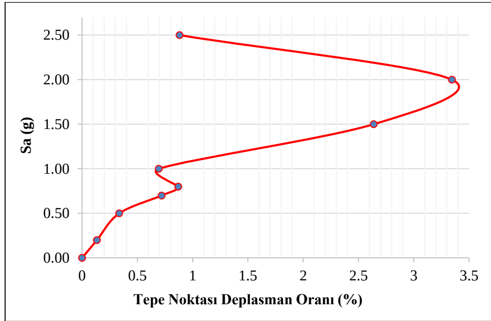
Şekil 5.32 : 9 Katlı Bina için Kocaeli Depremi Tepe Noktası Deplasman Oranı (min).
