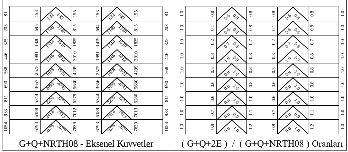
Şekil 5.183 : 9 Katlı Çerçevenin G+Q+2E /G+Q+NRTH (SF=0.8) Oranları.
