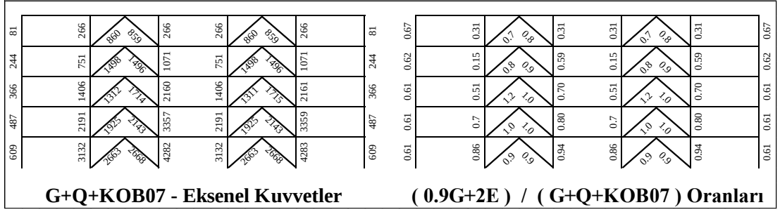
Şekil 5.75 : 5 Katlı Çerçevenin 0.9G+2E /G+Q+KOB (SF=0.7) Oranları.
