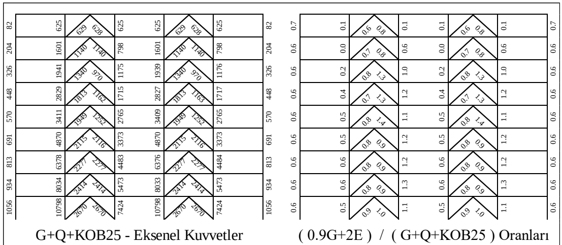
Şekil 5.155 : 9 Katlı Çerçevenin 0.9G+2E /G+Q+KOB (SF=2.5) Oranları.
