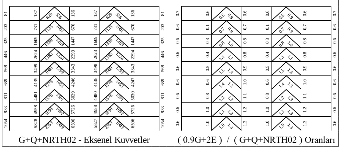
Şekil 5.156 : 9 Katlı Çerçevenin 0.9G+2E /G+Q+NRTH (SF=0.2) Oranları.
