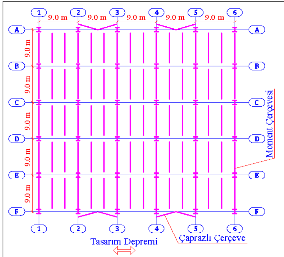
Şekil 4.1 : 5 Katlı Yapının Planı.
