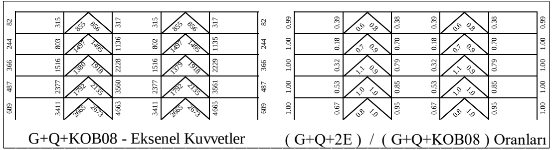
Şekil 5.100 : 5 Katlı Çerçevenin G+Q+2E /G+Q+KOB (SF=0.8) Oranları.
