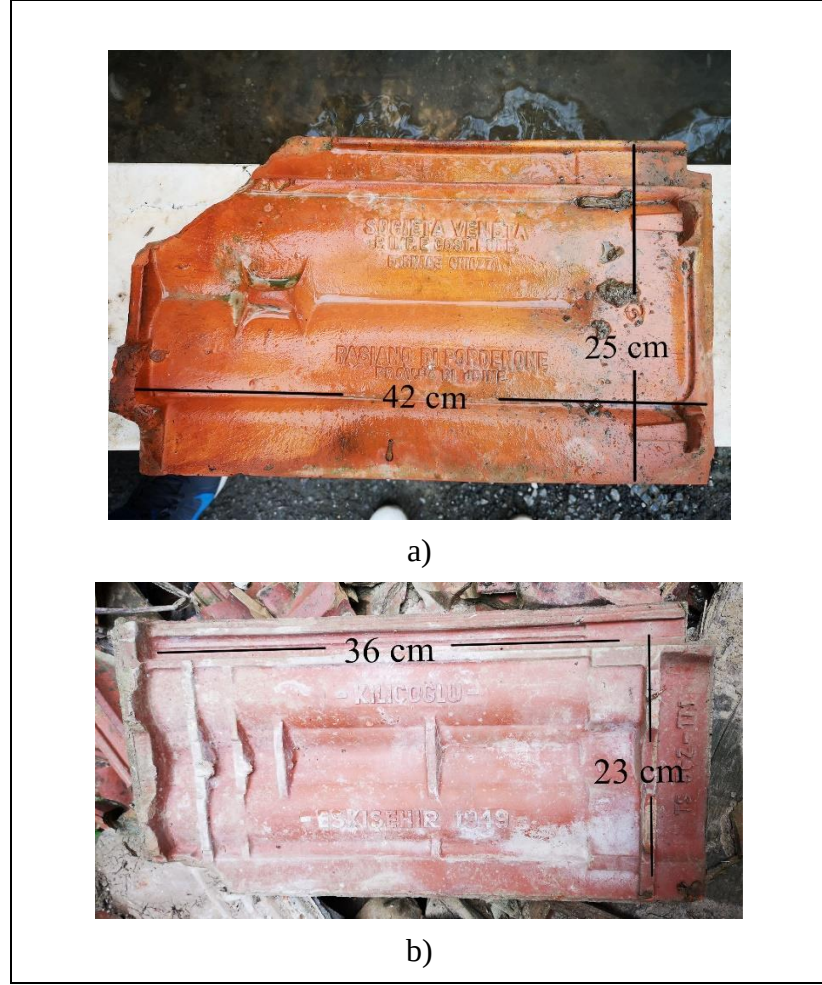
Şekil 4.48: a) İtalya'dan gelen özgün kiremit numunesi, b) Eskişehir'den gelen kiremit numunesi.
