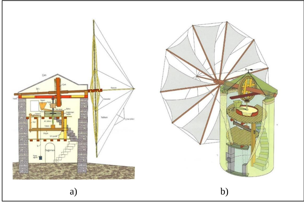
Şekil 3.29: a) Batı türü bir Akdeniz yel değirmeninin kesiti, b) Akdeniz yel değirmeninin perspektif kesiti.
