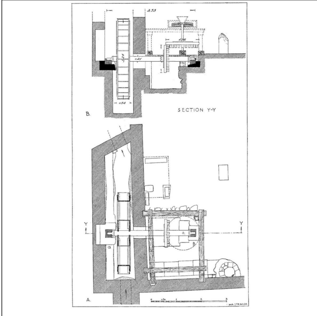
Şekil 3.26: Değirmen plan ve kesit restitüsyon önerisi.
