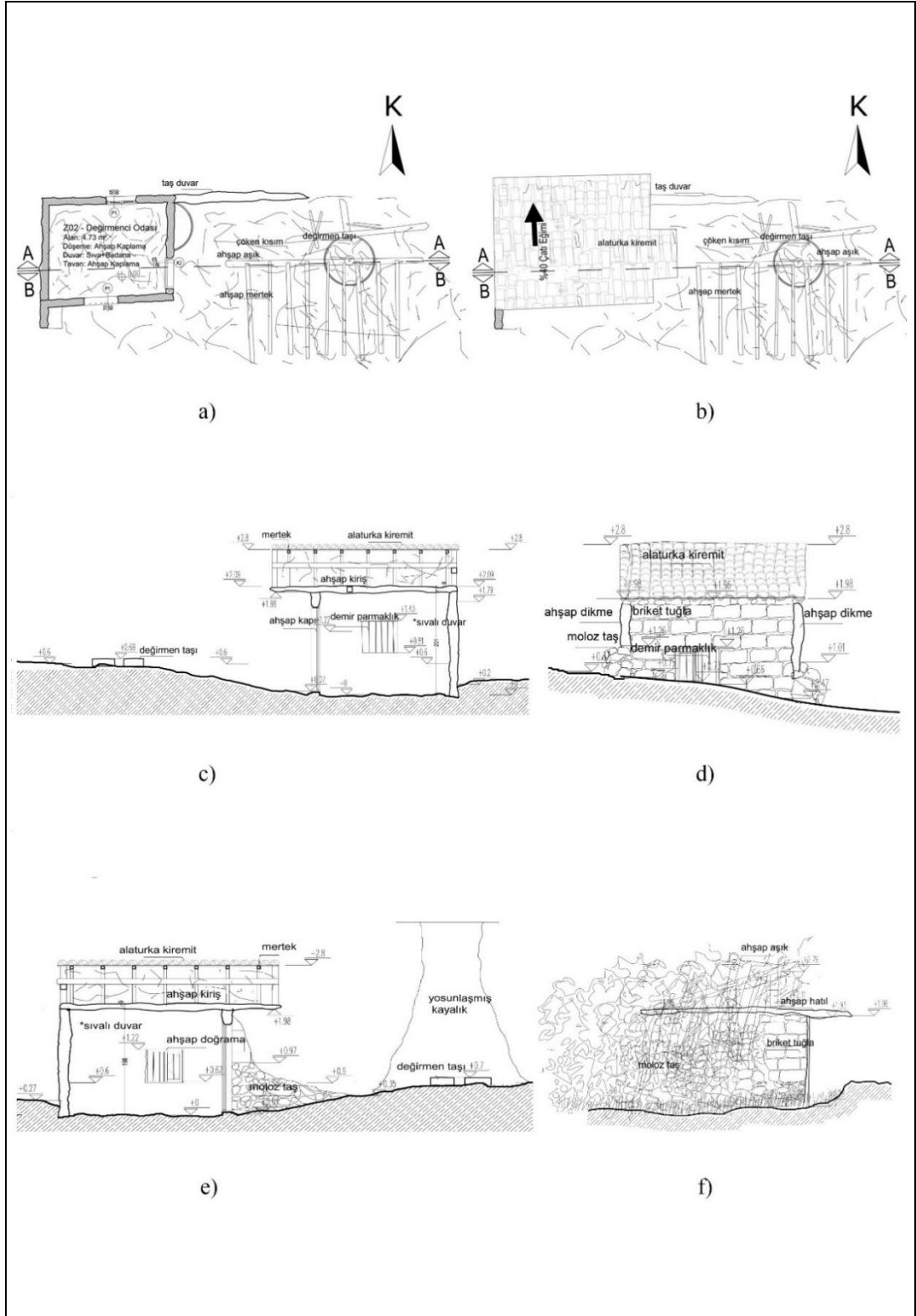
Şekil 5.10: a) Zemin kat planı, b) Çatı planı, c) B-B Kesiti, d) Kuzey cephesi, e) A-A kesiti, f) Batı cephesi (Mecidiye Değirmeni rölöve çizimleri- Mimar E. Arısal KKTVBK arşivi).
