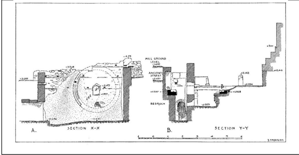
Şekil 3.25: Atina Agorası Değirmeni rölöve çizimleri.
