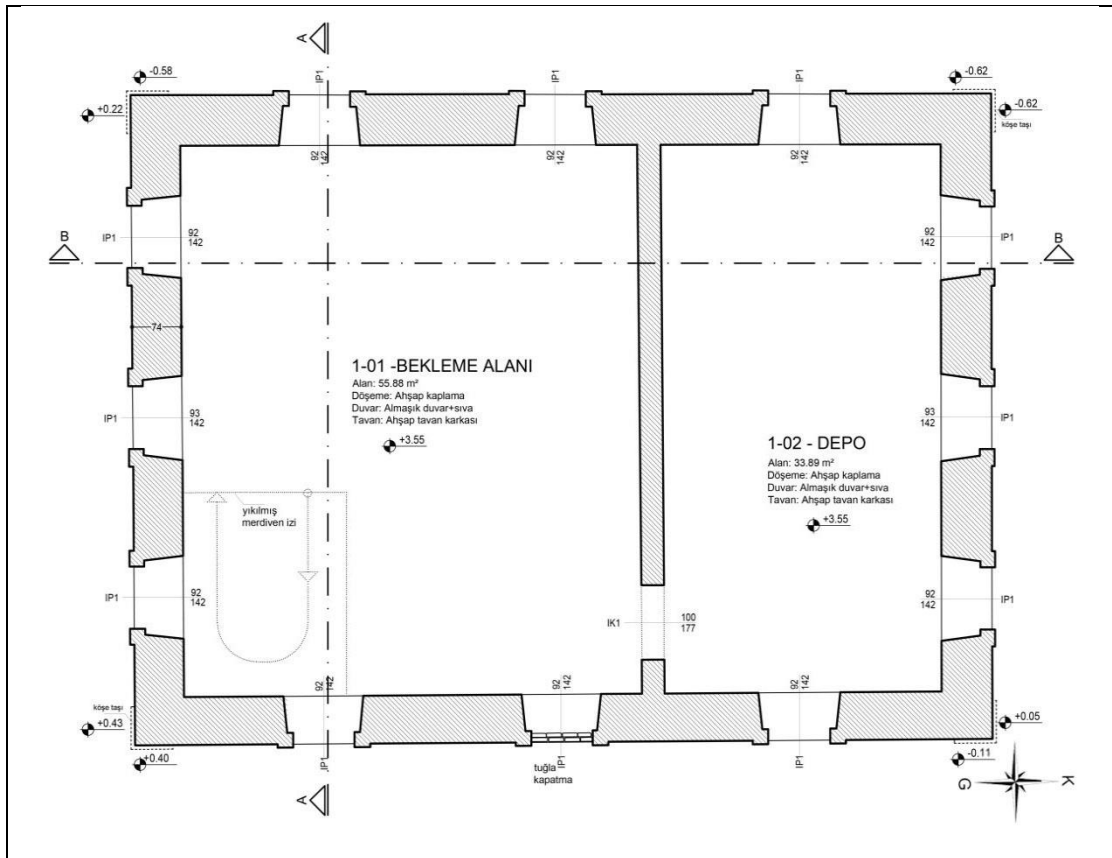
Şekil 4.15: Birinci kat rölöve çizimi.
