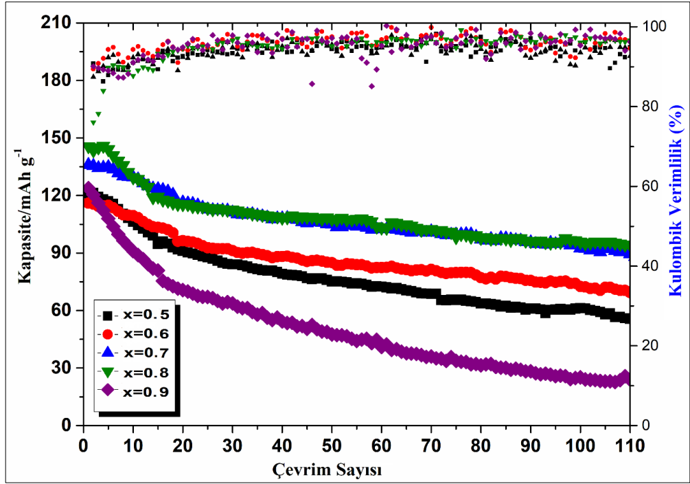
Şekil 4.44: 1.5-4.0 V gerilim aralığında 0.05C deşarj hızında \text{Na}_x(\text{Fe}_{0.35}\text{Mn}_{0.35}\text{Co}_{0.3})\text{O}_2 ( x = 0.5, 0.6, 0.7, 0.8, 0.9 ) malzemelerinin çevrim performansı.
