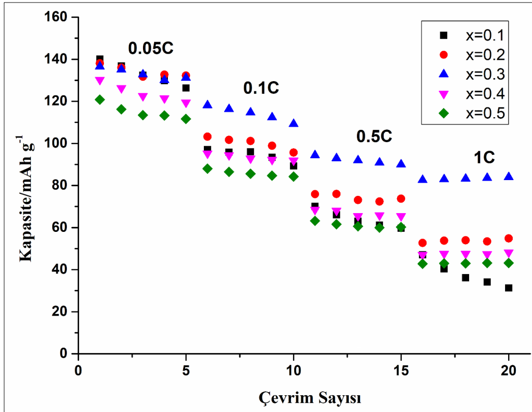
Şekil 4.25: Sol jel yöntemi ile sentezlenen \text{Na}_{0.7}(\text{Mn}_{0.5}\text{Fe}_{0.5})_{1-x}\text{Co}_x\text{O}_2 ( x = 0.1, 0.2, 0.3, 0.4, 0.5 ) katot aktif malzemelerin farklı C hızlarında hız kapasiteleri.
