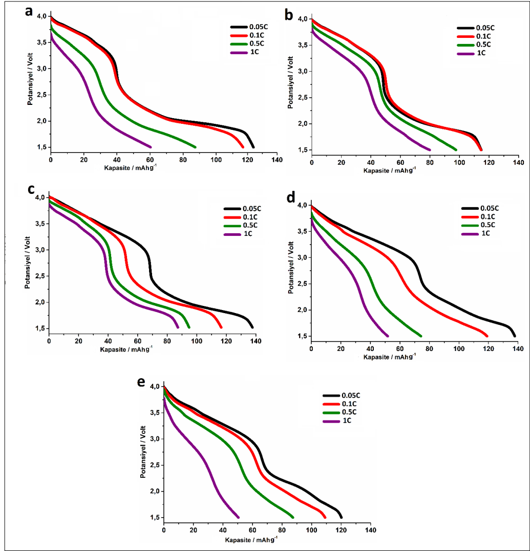
Şekil 4.41: a. \text{Na}_{0.5}(\text{Fe}_{0.35}\text{Mn}_{0.35}\text{Co}_{0.3})\text{O}_2 b. \text{Na}_{0.6}(\text{Fe}_{0.35}\text{Mn}_{0.35}\text{Co}_{0.3})\text{O}_2 c. \text{Na}_{0.7}(\text{Fe}_{0.35}\text{Mn}_{0.35}\text{Co}_{0.3})\text{O}_2 d. \text{Na}_{0.8}(\text{Fe}_{0.35}\text{Mn}_{0.35}\text{Co}_{0.3})\text{O}_2 e. \text{Na}_{0.9}(\text{Fe}_{0.35}\text{Mn}_{0.35}\text{Co}_{0.3})\text{O}_2 numunelerine ait 1.5-4 V potansiyel aralığında 0.05C ile 1C akım yoğunluğunda ki deşarj eğrileri.
