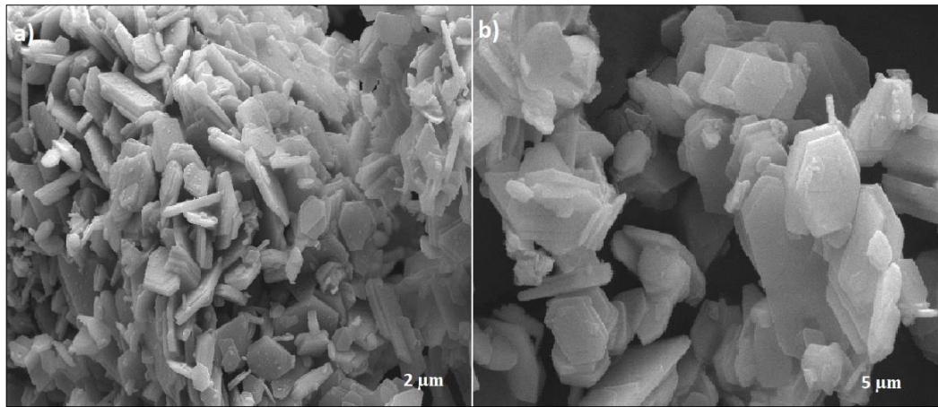
Şekil 4.13: Sol jel yöntemi ile sentezlenen \text{Na}_{0.7}\text{Mn}_{0.45}\text{Fe}_{0.45}\text{Co}_{0.1}\text{O}_2 bileşiğine ait a) 2 \mu\text{m} ve b) 5 \mu\text{m} SEM görüntüleri.
