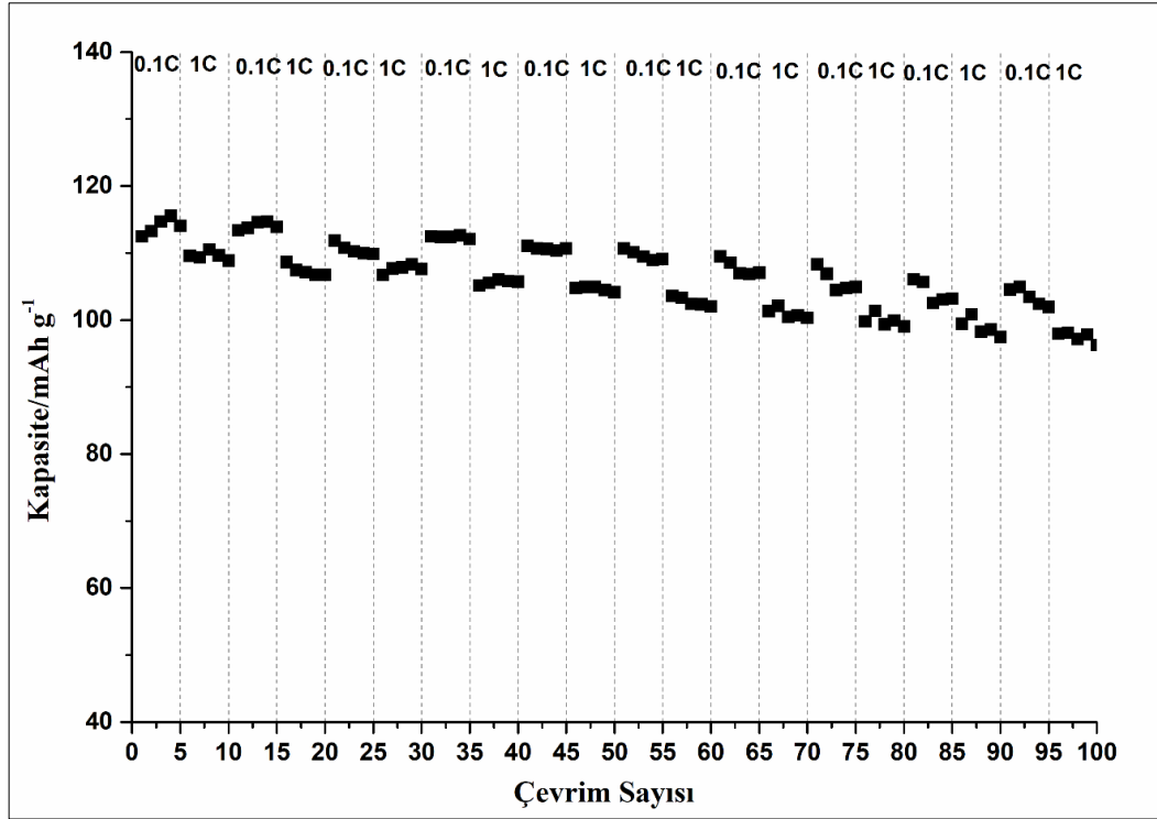
Şekil 4.4: Katı hal yöntemi ile sentezlenen \text{Na}_{0.7}\text{CoO}_2 maddesinin deşarj kapasitesinin akım yoğunluğu ile değişimi.
