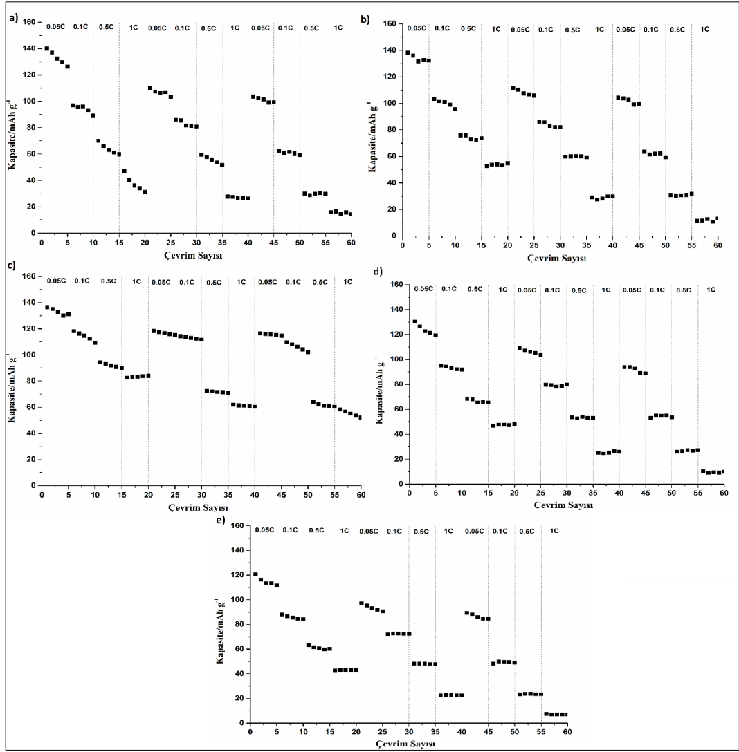
Şekil 4.26: Sol jel yöntemi ile sentezlenen a) Na 0.7 Mn 0.45 Fe 0.45 Co 0.1 O 2 b) Na 0.7 Mn 0.4 Fe 0.4 Co 0.2 O 2 c) Na 0.7 Mn 0.35 Fe 0.35 Co 0.3 O 2 d) Na 0.7 Mn 0.3 Fe 0.3 Co 0.4 O 2 e) Na 0.7 Mn 0.25 Fe 0.25 Co 0.5 O 2 numunelerine ait deşarj kapasitesinin akım yoğunluğu ile değişimi.
