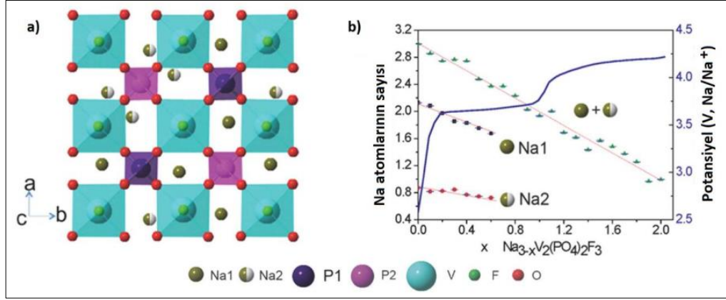
Şekil 2.13: \text{Na}_3\text{V}_2(\text{PO}_4)_2\text{F}_3 maddesinin a) Kristal yapısı ve b) Şarj/deşarj eğrisi.
