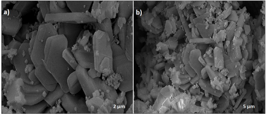
Şekil 4.32: Sol jel yöntemi ile sentezlenen \text{Na}_{0.6}\text{Mn}_{0.35}\text{Fe}_{0.35}\text{Co}_{0.3}\text{O}_2 bileşiğine ait a) 2 μm ve b) 5 μm SEM görüntüleri.
