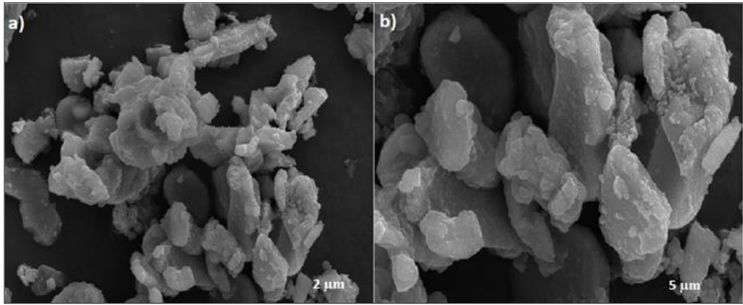
Şekil 4.7: Katı hal yöntemi ile sentezlenen \text{Na}_{0.7}\text{Fe}_{0.5}\text{Mn}_{0.5}\text{O}_2 bileşiğine ait a) 2 \mu\text{m} ve b) 5 \mu\text{m} SEM görüntüleri.
