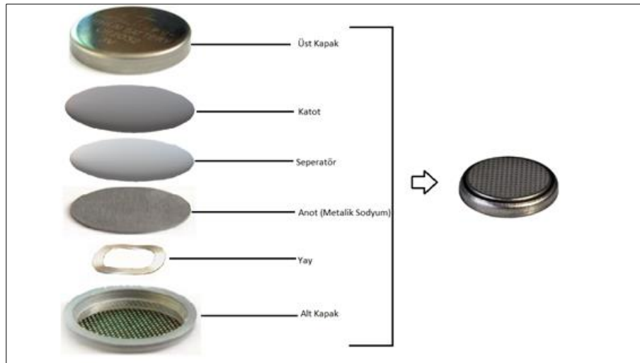
Şekil 3.2. Düğme tipi pillerin şematik olarak görünümü.
