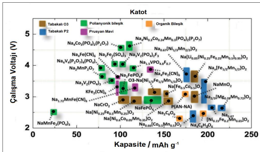
Şekil 2.8: Sodyum iyon pillerde kullanılan bazı katot aktif maddelerin spesifik kapasitesine karşı çalışma voltajı.
