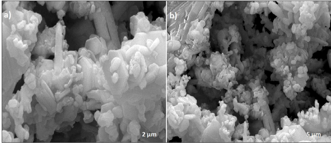
Şekil 4.55: Sol jel yöntemi ile sentezlenen \text{K}_{0.005}\text{Na}_{0.595}\text{Mn}_{0.35}\text{Fe}_{0.35}\text{Co}_{0.3}\text{O}_2 bileşiğine ait a) 2 \mu\text{m} ve b) 5 \mu\text{m} taramalı elektron mikroskobu (SEM) görüntüleri.
