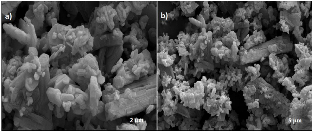
Şekil 4.18: Katı hal yöntemi ile sentezlenen \text{Na}_{0.7}\text{Mn}_{0.45}\text{Fe}_{0.45}\text{Co}_{0.1}\text{O}_2 bileşiğine ait a) 2 μm ve b) 5 μm SEM görüntüleri.
