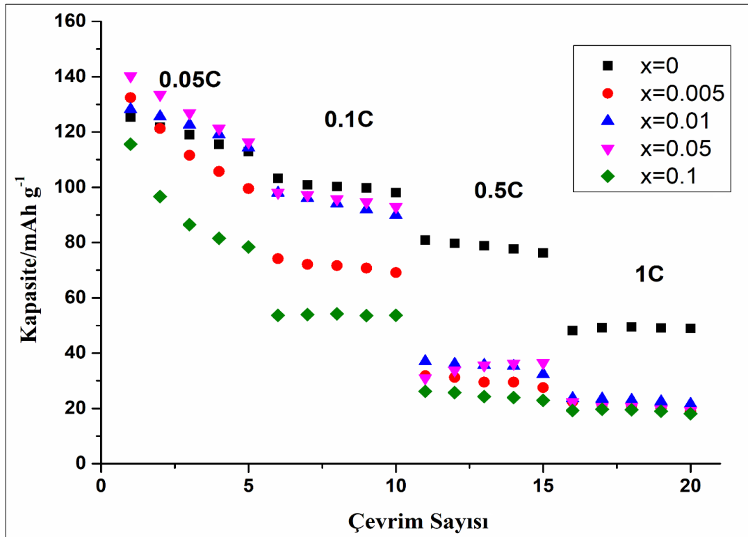
Şekil 4.78: Katı hal yöntemi ile sentezlenen 1.5-4.0 V gerilim aralığında \text{K}_x\text{Na}_{0.9-x}\text{Mn}_{0.35}\text{Fe}_{0.35}\text{Co}_{0.3}\text{O}_2 ( x= 0, 0.005, 0.01, 0.05, 0.1 ) katot aktif malzemelerin farklı C hızlarında hız kapasiteleri.
