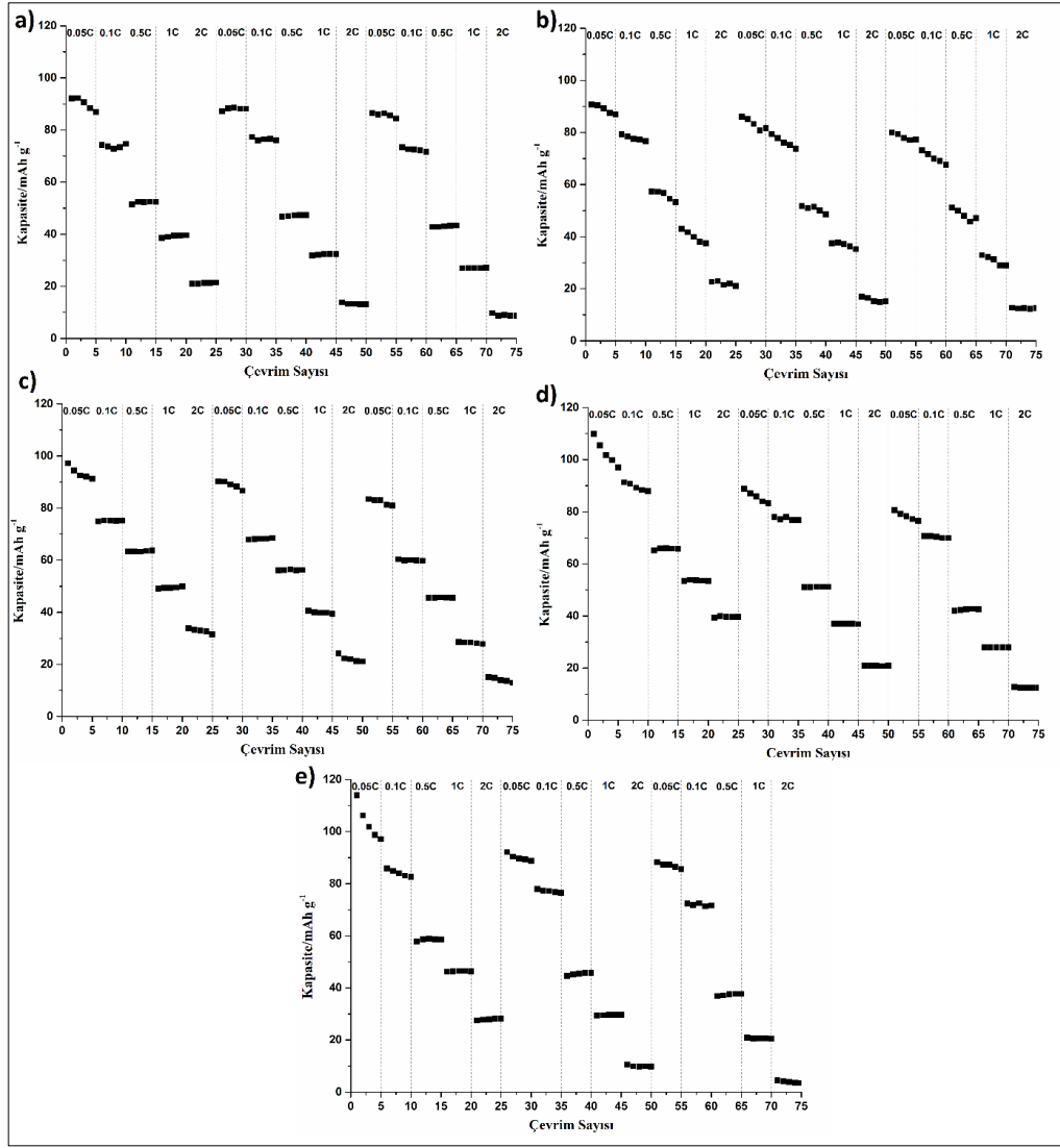
Şekil 4.50: Katı hal yöntemi ile sentezlenen 2.0-4.0 V voltaj aralığında a) \text{Na}_{0.5}\text{Mn}_{0.35}\text{Fe}_{0.35}\text{Co}_{0.3}\text{O}_2 b) \text{Na}_{0.6}\text{Mn}_{0.35}\text{Fe}_{0.35}\text{Co}_{0.3}\text{O}_2 c) \text{Na}_{0.7}\text{Mn}_{0.35}\text{Fe}_{0.35}\text{Co}_{0.3}\text{O}_2 d) \text{Na}_{0.8}\text{Fe}_{0.35}\text{Mn}_{0.35}\text{Co}_{0.3}\text{O}_2 e) \text{Na}_{0.9}\text{Fe}_{0.35}\text{Mn}_{0.35}\text{Co}_{0.3}\text{O}_2 numunelerine ait deşarj kapasitesinin akım yoğunluğu ile değişimi.
