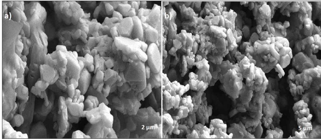
Şekil 4.70: Katı hal yöntemi ile sentezlenen K_{0.1}Na_{0.8}Mn_{0.35}Fe_{0.35}Co_{0.3}O_2 bileşiğine ait a) 2 \mu m ve b) 5 \mu m taramalı elektron mikroskobu (SEM) görüntüleri.
