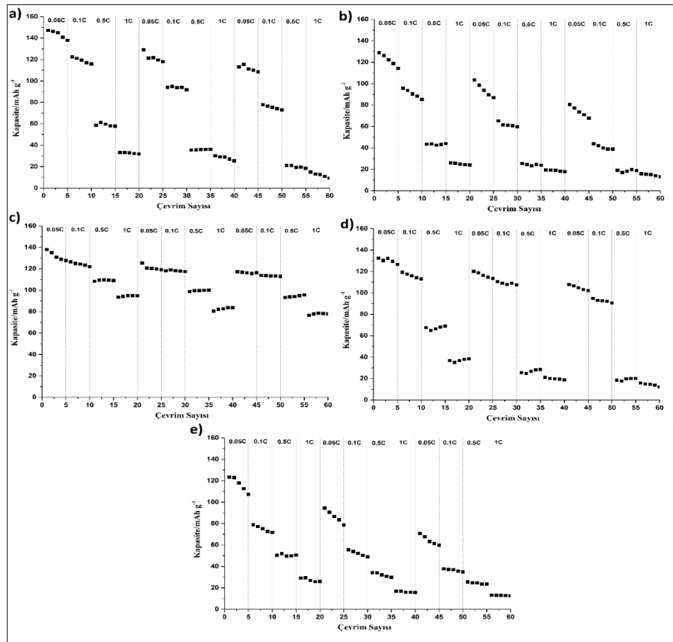
Şekil 4.75: Katı hal yöntemi ile sentezlenen 1.5-4.0 V voltaj aralığında a) Na_{0.6}Mn_{0.35}Fe_{0.35}Co_{0.3}O_2 b) K_{0.005}Na_{0.595}Mn_{0.35}Fe_{0.35}Co_{0.3}O_2 c) K_{0.01}Na_{0.59}Mn_{0.35}Fe_{0.35}Co_{0.3}O_2 d) K_{0.05}Na_{0.55}Mn_{0.35}Fe_{0.35}Co_{0.3}O_2 e) K_{0.1}Na_{0.5}Mn_{0.35}Fe_{0.35}Co_{0.3}O_2 numunelerine ait deşarj kapasitesinin akım yoğunluğu ile değişimi.
