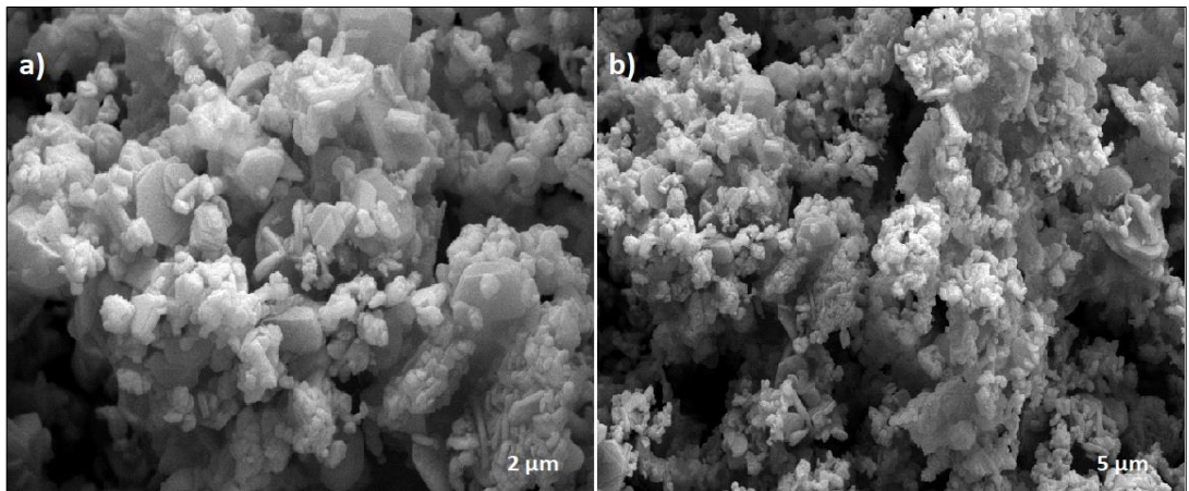
Şekil 4.22: Katı hal yöntemi ile sentezlenen \text{Na}_{0.7}\text{Mn}_{0.25}\text{Fe}_{0.25}\text{Co}_{0.5}\text{O}_2 bileşiğine ait a) 2 \mu\text{m} ve b) 5 \mu\text{m} SEM görüntüleri.
