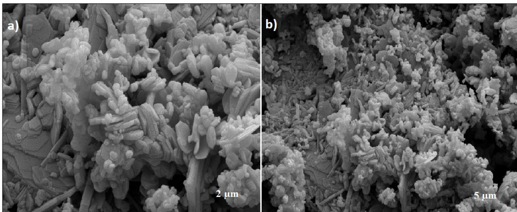
Şekil 4.19: Katı hal yöntemi ile sentezlenen \text{Na}_{0.7}\text{Mn}_{0.4}\text{Fe}_{0.4}\text{Co}_{0.2}\text{O}_2 bileşiğine ait a) 2 μm ve b) 5 μm SEM görüntüleri.
