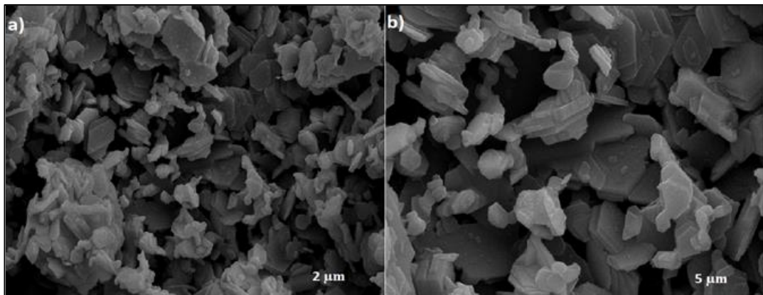
Şekil 4.8: Sol jel yöntemi ile sentezlenen \text{Na}_{0.7}\text{Fe}_{0.5}\text{Mn}_{0.5}\text{O}_2 bileşiğine ait a) 2 \mu\text{m} ve b) 5 \mu\text{m} SEM görüntüleri.
