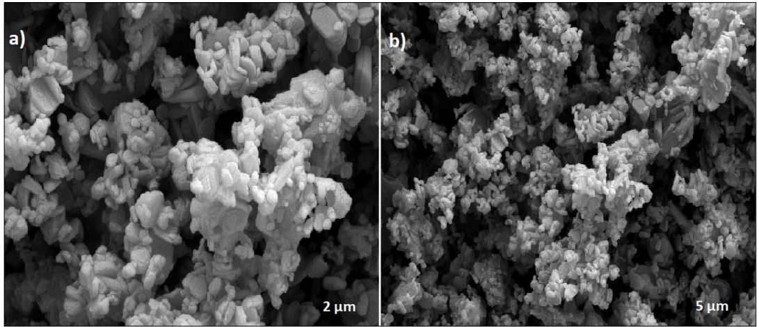
Şekil 4.21: Katı hal yöntemi ile sentezlenen \text{Na}_{0.7}\text{Mn}_{0.3}\text{Fe}_{0.3}\text{Co}_{0.4}\text{O}_2 bileşiğine ait a) 2 \mu\text{m} ve b) 5 \mu\text{m} SEM görüntüleri.
