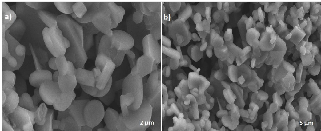
Şekil 4.66: Sol jel yöntemi ile sentezlenen K_{0.1}Na_{0.8}Mn_{0.35}Fe_{0.35}Co_{0.3}O_2 bileşiğine ait a) 2 \mu m ve b) 5 \mu m taramalı elektron mikroskobu (SEM) görüntüleri.
