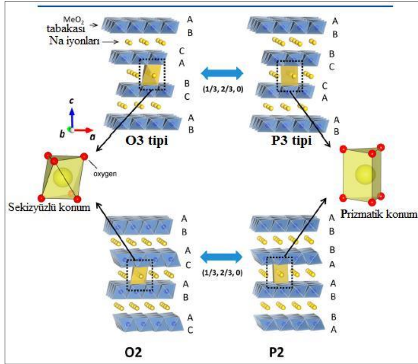
Şekil 2.10: Tabakalı \text{NaMO}_2 maddelerin yapıları ve faz dönüşümleri.
