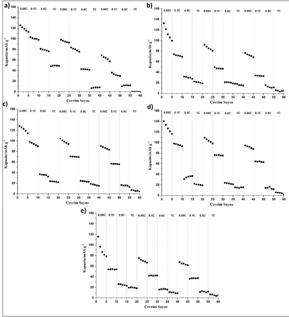
Şekil 4.79: Katı hal yöntemi ile sentezlenen 1.5-4.0 V voltaj aralığında a) \text{Na}_{0.9}\text{Mn}_{0.35}\text{Fe}_{0.35}\text{Co}_{0.3}\text{O}_2 b) \text{K}_{0.005}\text{Na}_{0.895}\text{Mn}_{0.35}\text{Fe}_{0.35}\text{Co}_{0.3}\text{O}_2 c) \text{K}_{0.01}\text{Na}_{0.89}\text{Mn}_{0.35}\text{Fe}_{0.35}\text{Co}_{0.3}\text{O}_2 d) \text{K}_{0.05}\text{Na}_{0.85}\text{Mn}_{0.35}\text{Fe}_{0.35}\text{Co}_{0.3}\text{O}_2 e) \text{K}_{0.1}\text{Na}_{0.8}\text{Mn}_{0.35}\text{Fe}_{0.35}\text{Co}_{0.3}\text{O}_2 numunelerine ait deşarj kapasitesinin akım yoğunluğu ile değişimi.
