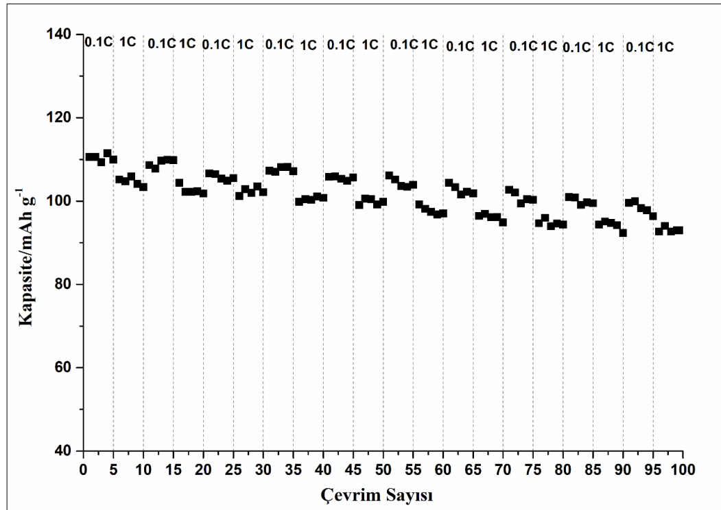
Şekil 4.5: Sol jel yöntemi ile sentezlenen \text{Na}_{0.7}\text{CoO}_2 maddesinin deşarj kapasitesinin akım yoğunluğu ile değişimi.
