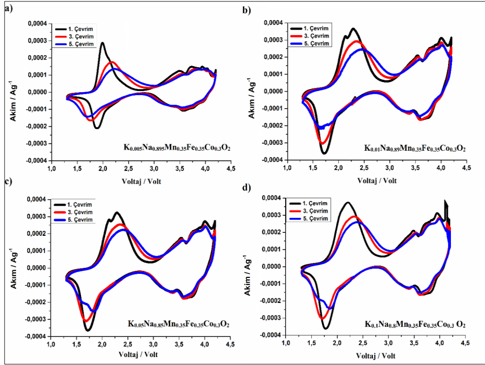
Şekil 4.72: 0.1 mVs -1 tarama hızında a) K 0.005 Na 0.895 Mn 0.35 Fe 0.35 Co 0.3 O 2 b) K 0.01 Na 0.89 Mn 0.35 Fe 0.35 Co 0.3 O 2 c) K 0.05 Na 0.85 Mn 0.35 Fe 0.35 Co 0.3 O 2 d) K 0.1 Na 0.8 Mn 0.35 Fe 0.35 Co 0.3 O 2 numunelerine ait CV eğrileri.
