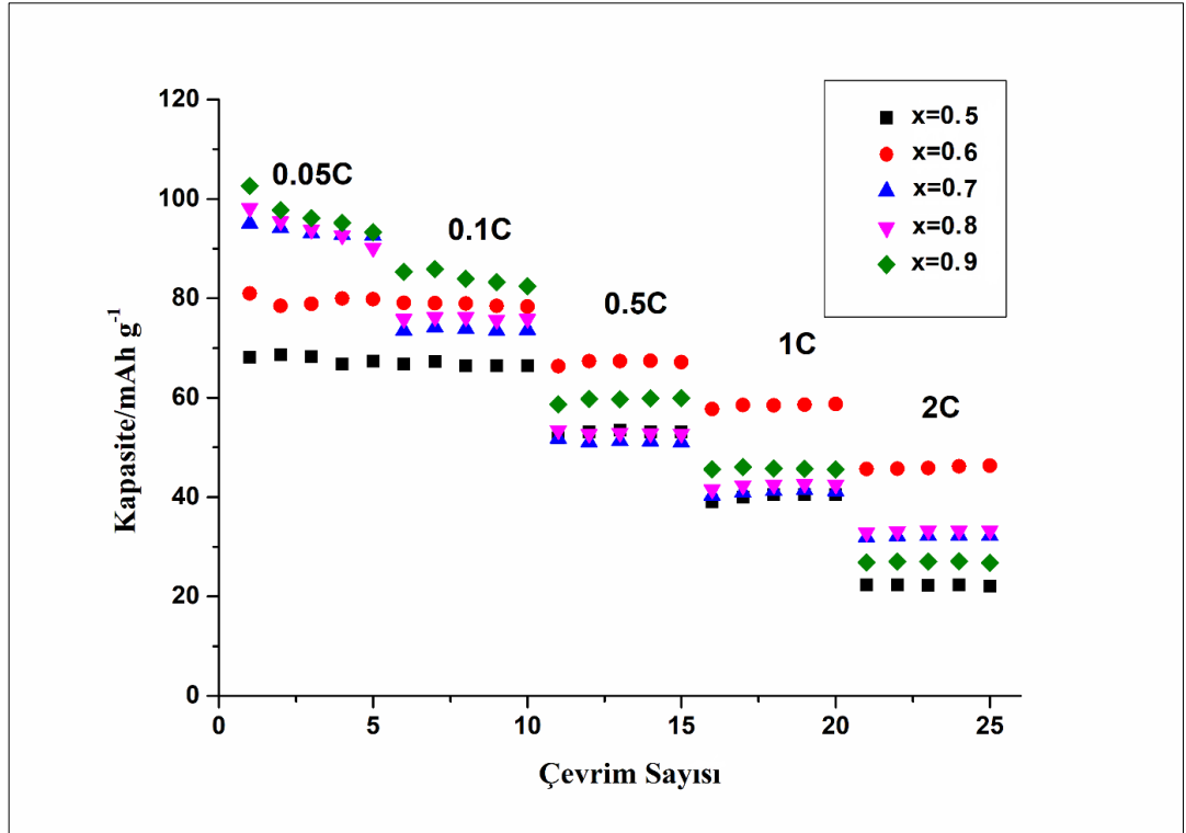
Şekil 4.45: Sol jel yöntemi ile sentezlenen 2-4.0 V gerilim aralığında Na x (Fe 0.35 Mn 0.35 Co 0.3 )O 2 (x = 0.5, 0.6, 0.7, 0.8, 0.9) katot aktif malzemelerin farklı C hızlarında hız kapasiteleri.
