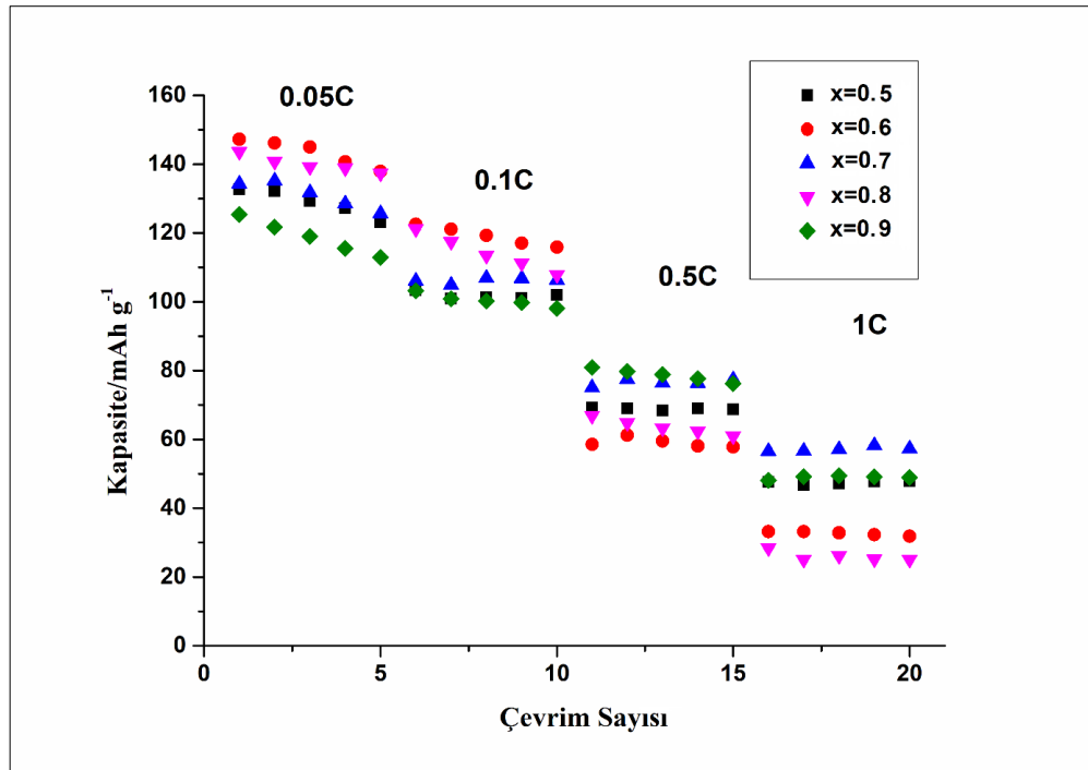
Şekil 4.47: Katı hal yöntemi ile sentezlenen 1.5-4.0 V gerilim aralığında \text{Na}_x(\text{Fe}_{0.35}\text{Mn}_{0.35}\text{Co}_{0.3})\text{O}_2 ( x = 0.5, 0.6, 0.7, 0.8, 0.9 ) katot aktif malzemelerin farklı C hızlarında hız kapasiteleri.
