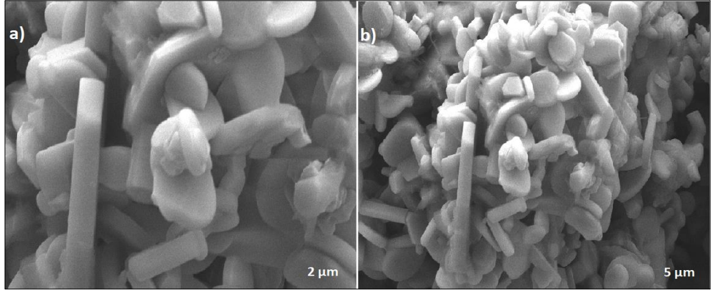
Şekil 4.64: Sol jel yöntemi ile sentezlenen K_{0.01}Na_{0.89}Mn_{0.35}Fe_{0.35}Co_{0.3}O_2 bileşiğine ait a) 2 \mu m ve b) 5 \mu m taramalı elektron mikroskobu (SEM) görüntüleri.
