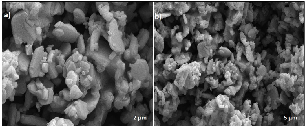
Şekil 4.69: Katı hal yöntemi ile sentezlenen K_{0.05}Na_{0.85}Mn_{0.35}Fe_{0.35}Co_{0.3}O_2 bileşiğine ait a) 2 \mu m ve b) 5 \mu m taramalı elektron mikroskobu (SEM) görüntüleri.
