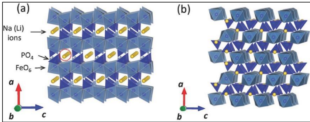
Şekil 2.14: Demir içeren fosfat temelli bileşiklerin kristal yapısı: a) Tripilit tipi \text{NaFePO}_4 , b) Marisit tipi \text{NaFePO}_4 .
