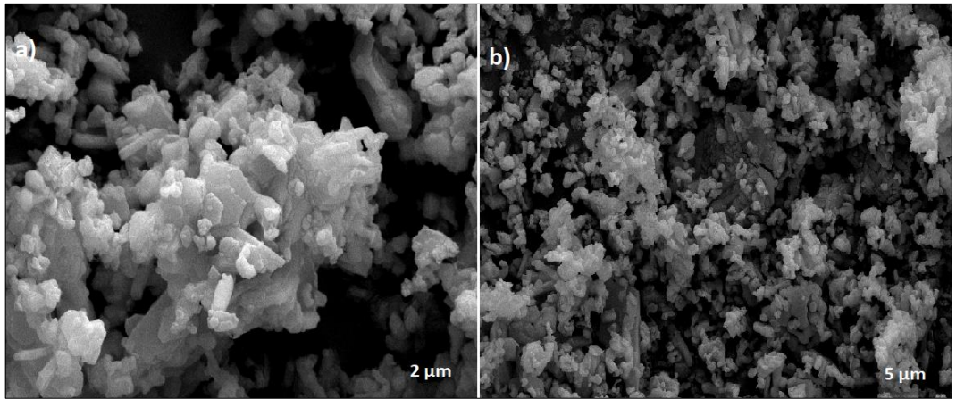
Şekil 4.35: Katı hal yöntemi ile sentezlenen P2 tipi \text{Na}_{0.5}\text{Mn}_{0.35}\text{Fe}_{0.35}\text{Co}_{0.3}\text{O}_2 bileşiğine ait a) 2 μm ve b) 5 μm taramalı elektron mikroskobu (SEM) görüntüleri.
