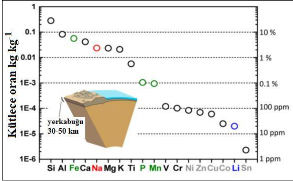
Şekil 2.9: Yer kabuğunda bulunan elementlerin bolluğu.
