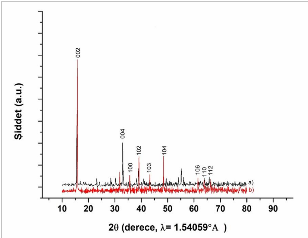
Şekil 4.6: a) Katı hal yöntemi ile sentezlenen ve b) Sol-jel yöntemi ile sentezlenen P2- \text{Na}_{0.7}\text{Fe}_{0.5}\text{Mn}_{0.5}\text{O}_2 maddesinin XRD toz desenleri.
