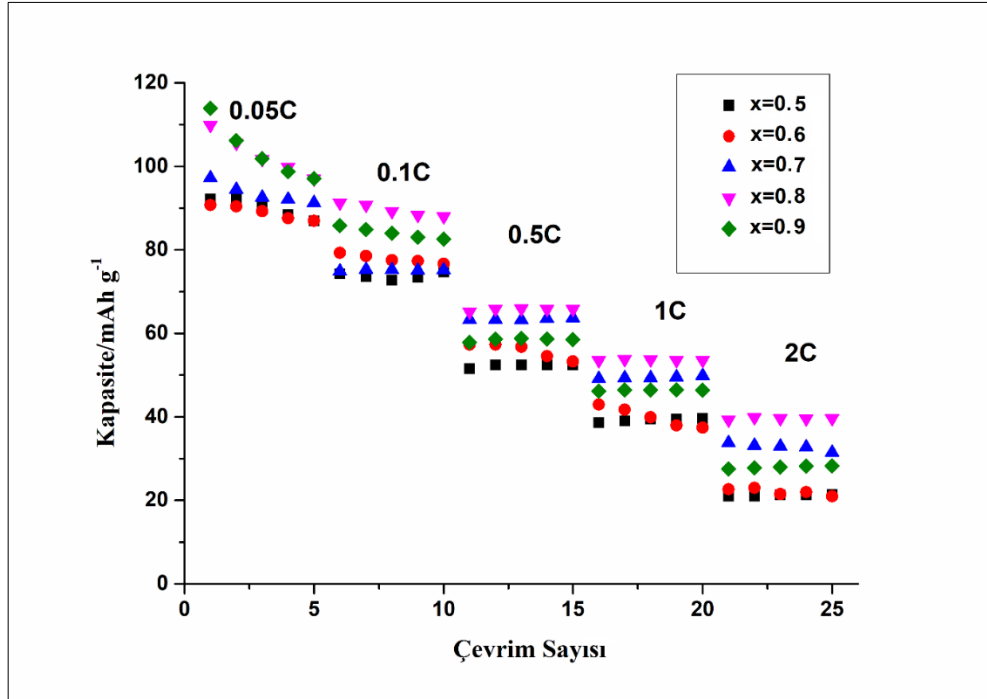
Şekil 4.49: Katı hal yöntemi ile sentezlenen 2-4.0 V gerilim aralığında \text{Na}_x(\text{Fe}_{0.35}\text{Mn}_{0.35}\text{Co}_{0.3})\text{O}_2 ( x = 0.5, 0.6, 0.7, 0.8, 0.9 ) katot aktif malzemelerin farklı C hızlarında hız kapasiteleri.
