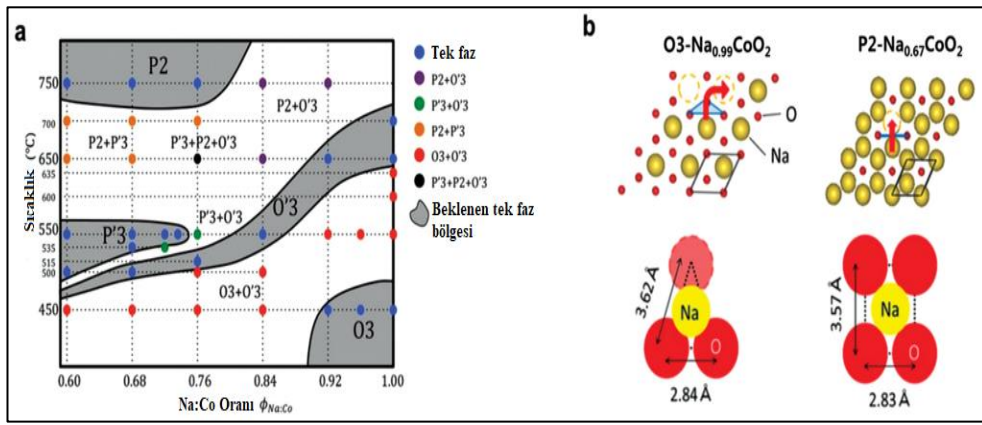
Şekil 2.11: a) Na:Co oranı ve sinterleme sıcaklığının bir fonksiyonu olarak \text{Na}_x\text{CoO}_2 sentez faz diyagramı. b) O3 tipi \text{Na}_{0.99}\text{CoO}_2 ve P2 tipi \text{Na}_{0.67}\text{CoO}_2 nin Na iyonu difüzyon yolu. Kırmızı oklar ve mavi işaretler sırasıyla Na iyon difüzyon yolunu ve oksijen penceresini temsil eder.
