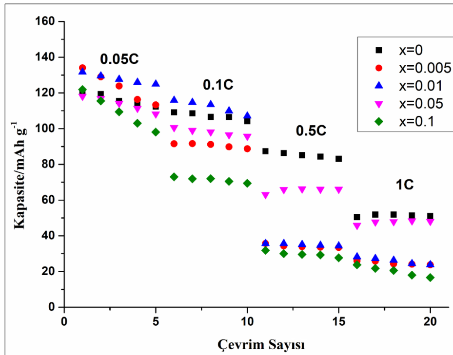
Şekil 4.80: Sol jel yöntemi ile sentezlenen 1.5-4.0 V gerilim aralığında \text{K}_x\text{Na}_{0.9-x}\text{Mn}_{0.35}\text{Fe}_{0.35}\text{Co}_{0.3}\text{O}_2 ( x= 0, 0.005, 0.01, 0.05, 0.1 ) katot aktif malzemelerin farklı C hızlarında hız kapasiteleri.
