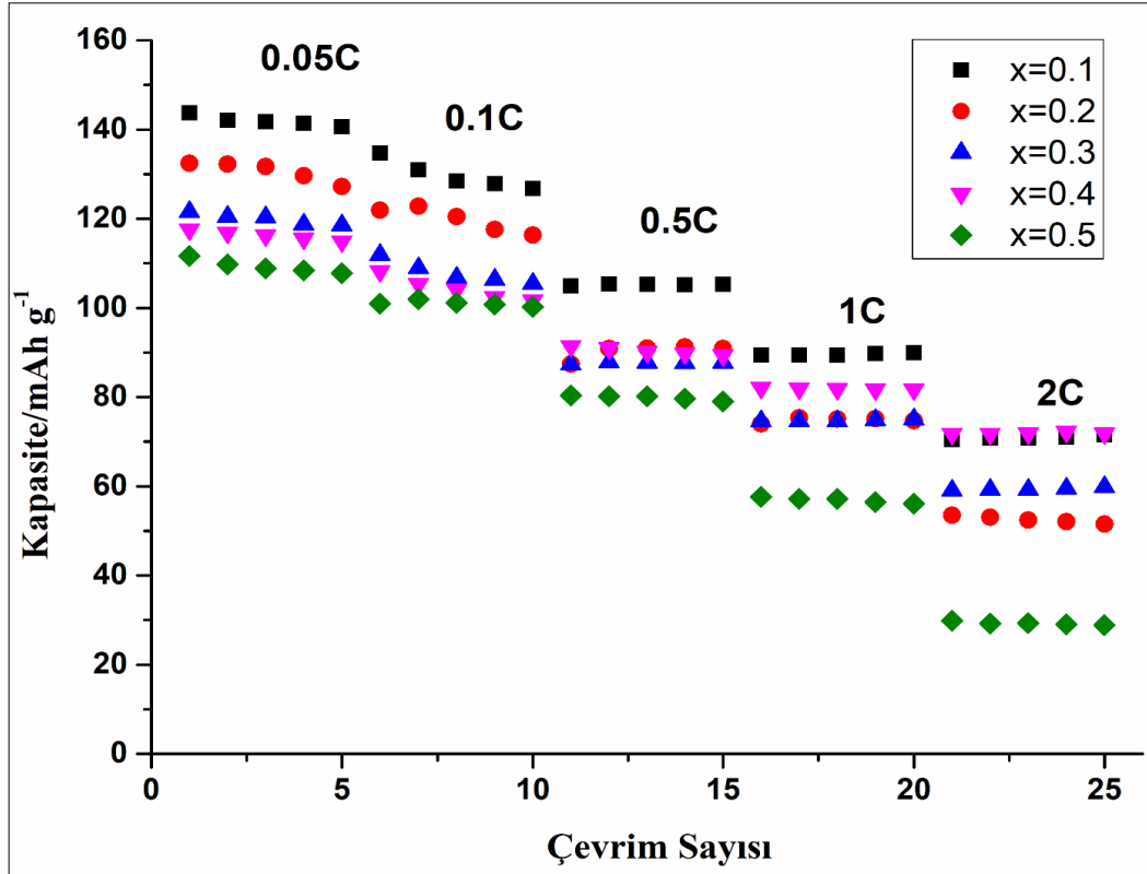
Şekil 4.27: Katı hal yöntemi ile sentezlenen \text{Na}_{0.7}(\text{Mn}_{0.5}\text{Fe}_{0.5})_{1-x}\text{Co}_x\text{O}_2 ( x = 0.1, 0.2, 0.3, 0.4, 0.5 ) katot aktif malzemelerin farklı C hızlarında hız kapasiteleri.
