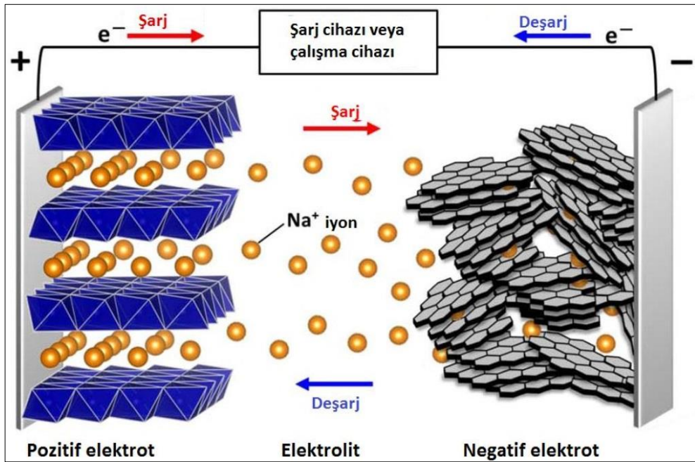
Şekil 2.7: Bir sodyum iyon pilin çalışma prensibi.
