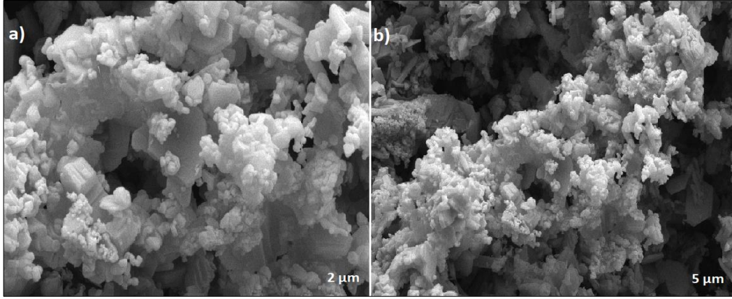
Şekil 4.60: Katı hal yöntemi ile sentezlenen K_{0.01}Na_{0.59}Mn_{0.35}Fe_{0.35}Co_{0.3}O_2 bileşiğine ait a) 2 \mu m ve b) 5 \mu m taramalı elektron mikroskobu (SEM) görüntüleri.
