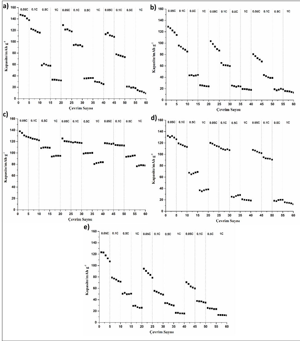
Şekil 4.77: Sol jel yöntemi ile sentezlenen 1.5-4.0 V voltaj aralığında a) \text{Na}_{0.6}\text{Mn}_{0.35}\text{Fe}_{0.35}\text{Co}_{0.3}\text{O}_2 b) \text{K}_{0.005}\text{Na}_{0.595}\text{Mn}_{0.35}\text{Fe}_{0.35}\text{Co}_{0.3}\text{O}_2 c) \text{K}_{0.01}\text{Na}_{0.59}\text{Mn}_{0.35}\text{Fe}_{0.35}\text{Co}_{0.3}\text{O}_2 d) \text{K}_{0.05}\text{Na}_{0.55}\text{Mn}_{0.35}\text{Fe}_{0.35}\text{Co}_{0.3}\text{O}_2 e) \text{K}_{0.1}\text{Na}_{0.5}\text{Mn}_{0.35}\text{Fe}_{0.35}\text{Co}_{0.3}\text{O}_2 numunelerine ait deşarj kapasitesinin akım yoğunluğu ile değişimi.
