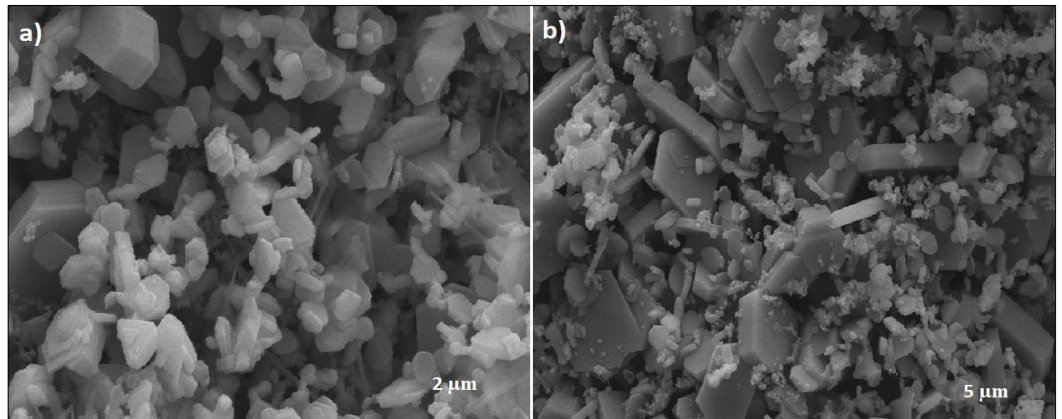
Şekil 4.16: Sol jel yöntemi ile sentezlenen \text{Na}_{0.7}\text{Mn}_{0.3}\text{Fe}_{0.3}\text{Co}_{0.4}\text{O}_2 bileşiğine ait a) 2 μm ve b) 5 μm SEM görüntüleri.
