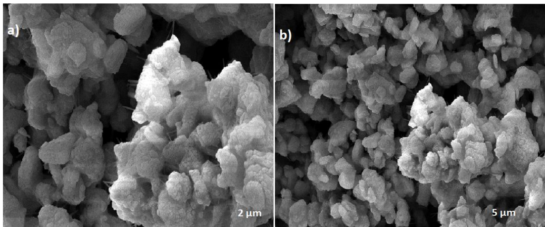
Şekil 4.38: Katı hal yöntemi ile sentezlenen O3 tipi \text{Na}_{0.9}\text{Mn}_{0.35}\text{Fe}_{0.35}\text{Co}_{0.3}\text{O}_2 bileşiğine ait a) 2 μm ve b) 5 μm taramalı elektron mikroskobu (SEM) görüntüleri.
