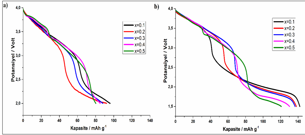
Şekil 4.24: Sol jel yöntemi ile sentezlenen \text{Na}_{0.7}(\text{Mn}_{0.5}\text{Fe}_{0.5})_{1-x}\text{Co}_x\text{O}_2 ( x= 0.1, 0.2, 0.3, 0.4, 0.5 ) numunelerinin a) 2-4.0\text{ V} ve b) 1.5-4\text{ V} potansiyel aralığında 0.05\text{C} akım yoğunluğunda ilk deşarj eğrileri.
