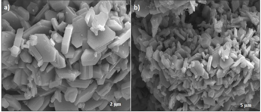
Şekil 4.14: Sol jel yöntemi ile sentezlenen \text{Na}_{0.7}\text{Mn}_{0.4}\text{Fe}_{0.4}\text{Co}_{0.2}\text{O}_2 bileşiğine ait a) 2 μm ve b) 5 μm SEM görüntüleri.
