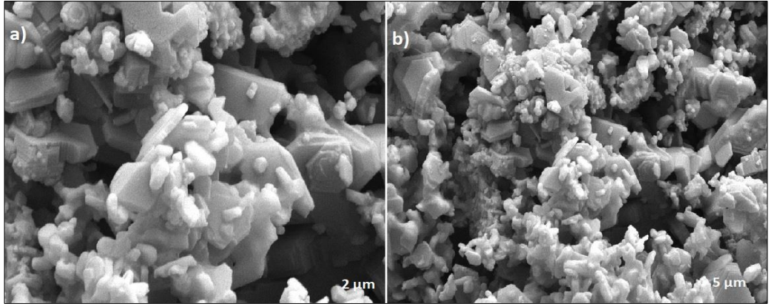
Şekil 4.57: Sol jel yöntemi ile sentezlenen K_{0.05}Na_{0.55}Mn_{0.35}Fe_{0.35}Co_{0.3}O_2 bileşiğine ait a) 2 \mu m ve b) 5 \mu m taramalı elektron mikroskobu (SEM) görüntüleri.
