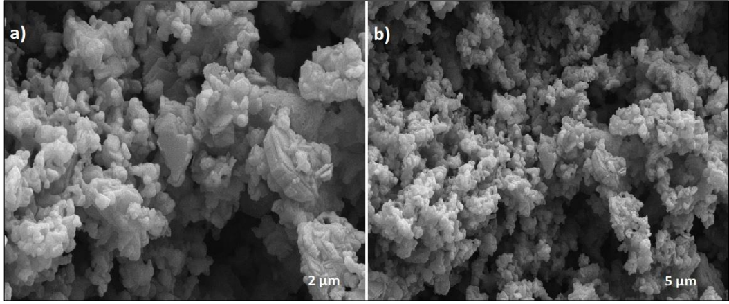
Şekil 4.62: Katı hal yöntemi ile sentezlenen K_{0.1}Na_{0.5}Mn_{0.35}Fe_{0.35}Co_{0.3}O_2 bileşiğine ait a) 2 \mu m ve b) 5 \mu m taramalı elektron mikroskobu (SEM) görüntüleri.
