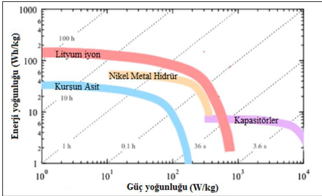
Şekil 2.1: Ragone Grafiği (Enerji yoğunluğu-güç yoğunluğu grafiği).
