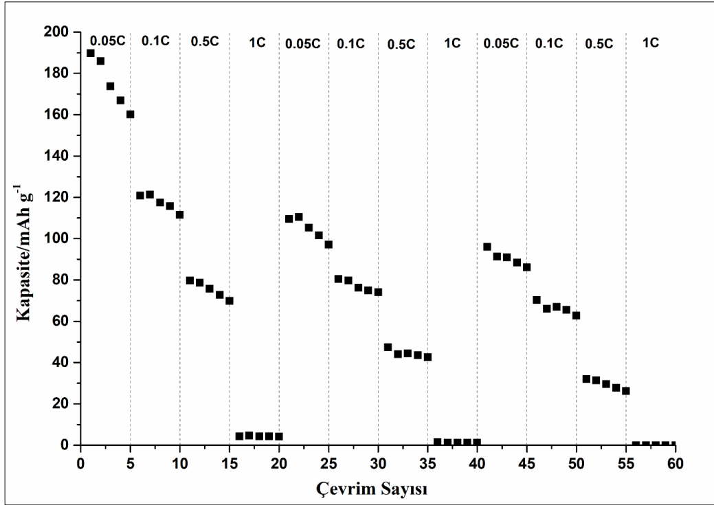
Şekil 4.10: Sol jel yöntemi ile sentezlenen \text{Na}_{0.7}\text{Fe}_{0.5}\text{Mn}_{0.5}\text{O}_2 maddesinin deşarj kapasitesinin akım yoğunluğu ile değişimi.
