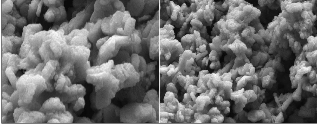
Şekil 4.68: Katı hal yöntemi ile sentezlenen K_{0.01}Na_{0.89}Mn_{0.35}Fe_{0.35}Co_{0.3}O_2 bileşiğine ait a) 2 \mu m ve b) 5 \mu m taramalı elektron mikroskobu (SEM) görüntüleri.
