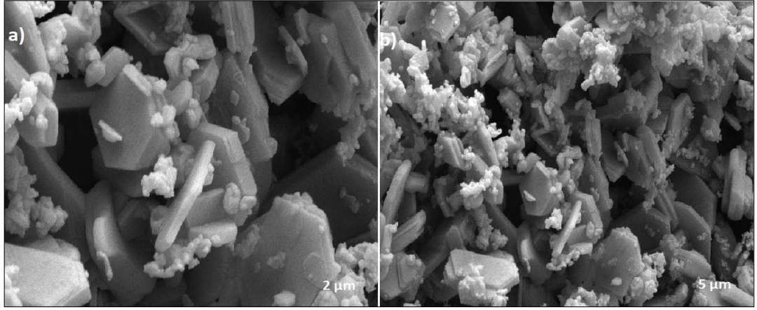
Şekil 4.56: Sol jel yöntemi ile sentezlenen K_{0.01}Na_{0.59}Mn_{0.35}Fe_{0.35}Co_{0.3}O_2 bileşiğine ait a) 2 \mu m ve b) 5 \mu m taramalı elektron mikroskobu (SEM) görüntüleri.
