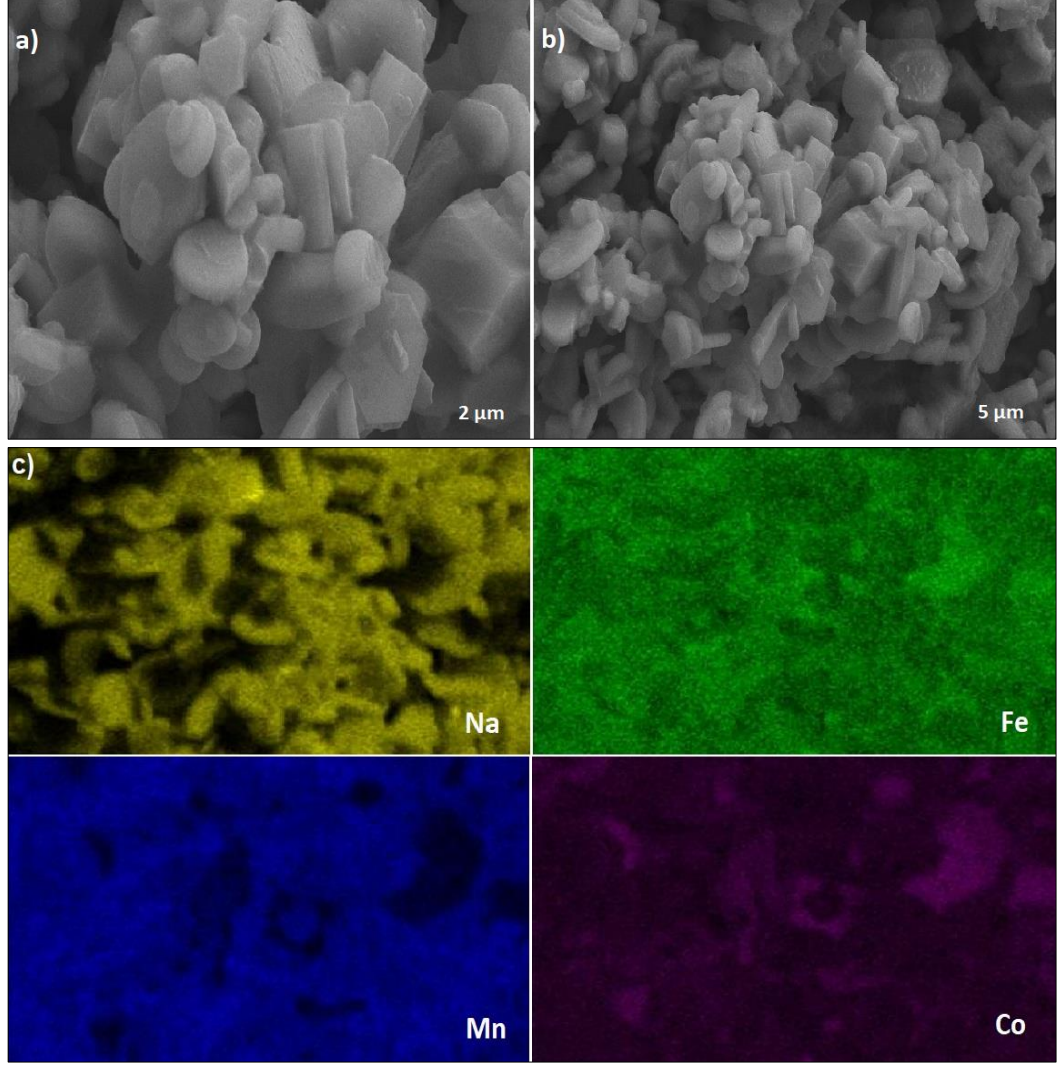
Şekil 4.34: Sol jel yöntemi ile sentezlenen \text{Na}_{0.9}\text{Mn}_{0.35}\text{Fe}_{0.35}\text{Co}_{0.3}\text{O}_2 bileşiğine ait a) 2 μm ve b) 5 μm SEM görüntüleri c) O3 tipi \text{Na}_{0.9}\text{Mn}_{0.35}\text{Fe}_{0.35}\text{Co}_{0.3}\text{O}_2 bileşiğinin EDS Haritalama görüntüleri.
