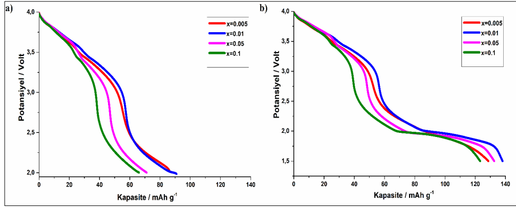
Şekil 4.73: Katı hal yöntemi ile sentezlenen K_xNa_{0.6-x}Mn_{0.35}Fe_{0.35}Co_{0.3}O_2 ( x = 0.005, 0.01, 0.05, 0.1 ) numunelerinin a) 2-4 V ve b) 1.5-4 V potansiyel aralığında 0.05C akım yoğunluğunda ilk deşarj eğrileri.
