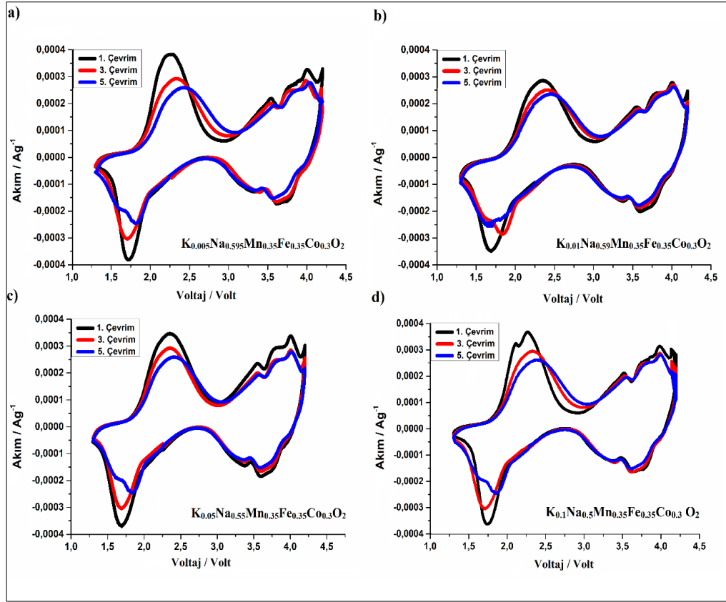
Şekil 4.71: 0.1 \text{ mVs}^{-1} tarama hızında a) K_{0.005}Na_{0.595}Mn_{0.35}Fe_{0.35}Co_{0.3}O_2 b) K_{0.01}Na_{0.59}Mn_{0.35}Fe_{0.35}Co_{0.3}O_2 c) K_{0.05}Na_{0.55}Mn_{0.35}Fe_{0.35}Co_{0.3}O_2 d) K_{0.1}Na_{0.5}Mn_{0.35}Fe_{0.35}Co_{0.3}O_2 O 2 numunelerine ait CV eğrileri.
