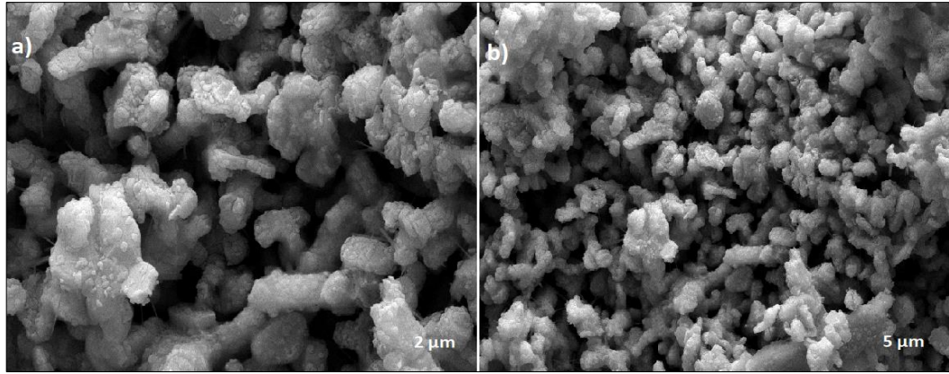
Şekil 4.37: Katı hal yöntemi ile sentezlenen O3 tipi \text{Na}_{0.8}\text{Mn}_{0.35}\text{Fe}_{0.35}\text{Co}_{0.3}\text{O}_2 bileşiğine ait a) 2 μm ve b) 5 μm taramalı elektron mikroskobu (SEM) görüntüleri.
