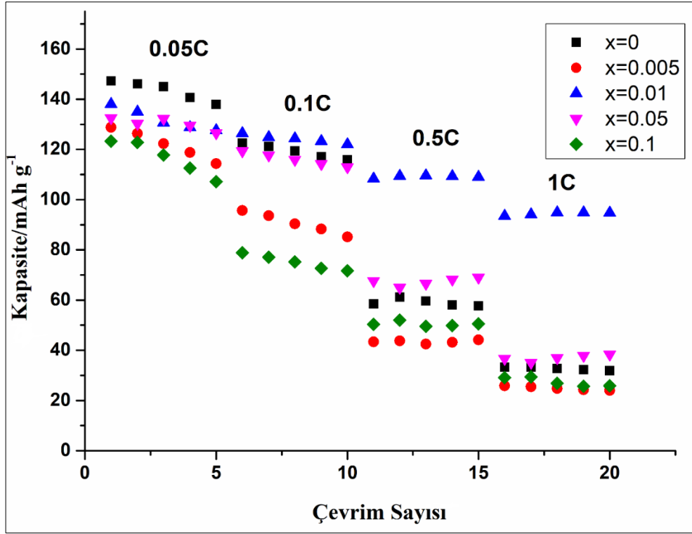
Şekil 4.74: Katı hal yöntemi ile sentezlenen 1.5-4.0 V gerilim aralığında K_xNa_{0.6-x}Mn_{0.35}Fe_{0.35}Co_{0.3}O_2 ( x = 0, 0.005, 0.01, 0.05, 0.1 ) katot aktif malzemelerin farklı C hızlarında hız kapasiteleri.
