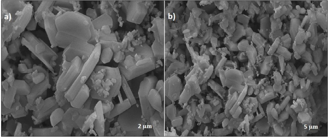
Şekil 4.15: Sol jel yöntemi ile sentezlenen \text{Na}_{0.7}\text{Mn}_{0.35}\text{Fe}_{0.35}\text{Co}_{0.3}\text{O}_2 bileşiğine ait a) 2 μm ve b) 5 μm SEM görüntüleri.
