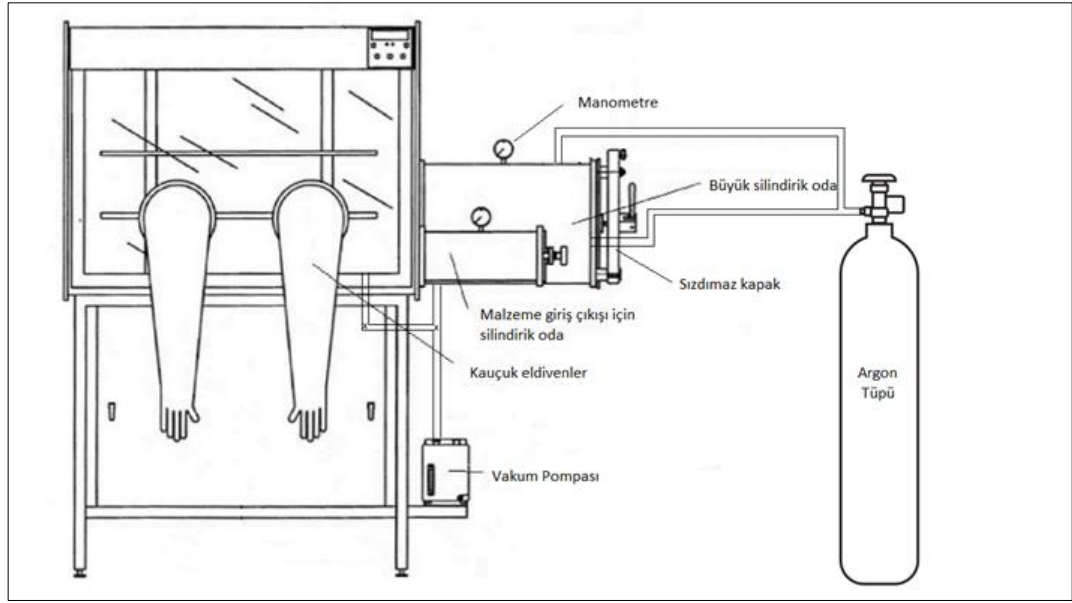
Şekil 3.1. Argon gaz kabini (Glove box).
