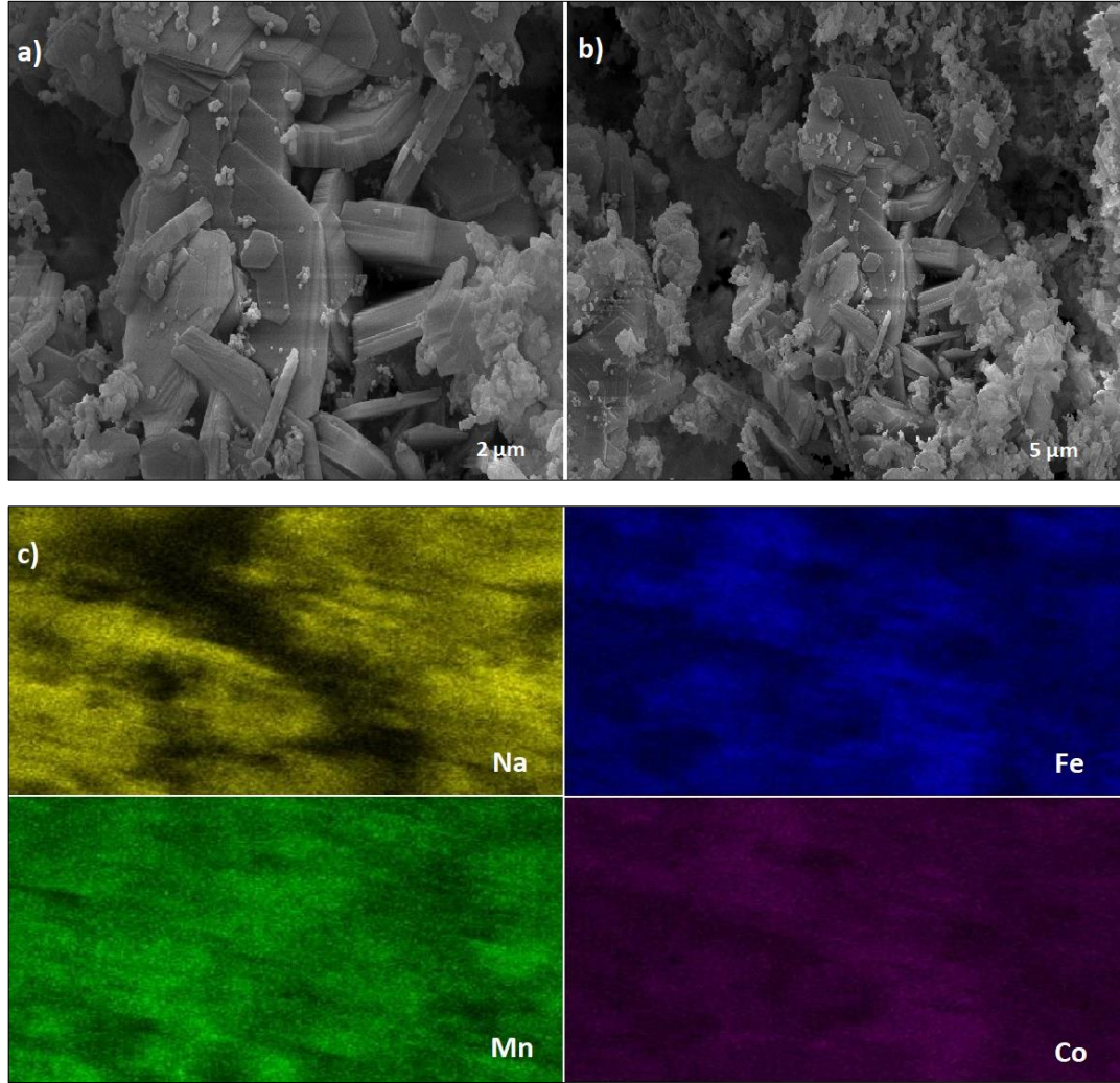
Şekil 4.31: Sol jel yöntemi ile sentezlenen \text{Na}_{0.5}\text{Mn}_{0.35}\text{Fe}_{0.35}\text{Co}_{0.3}\text{O}_2 bileşiğine ait a) 2 µm ve b) 5 µm SEM görüntüleri c) P2 tipi \text{Na}_{0.5}\text{Mn}_{0.35}\text{Fe}_{0.35}\text{Co}_{0.3}\text{O}_2 bileşiğinin EDS Haritalama görüntüleri.
