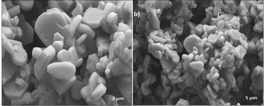
Şekil 4.65: Sol jel yöntemi ile sentezlenen K_{0.05}Na_{0.85}Mn_{0.35}Fe_{0.35}Co_{0.3}O_2 bileşiğine ait a) 2 \mu m ve b) 5 \mu m taramalı elektron mikroskobu (SEM) görüntüleri.
