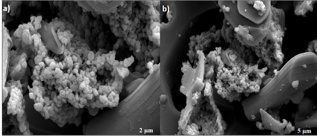
Şekil 4.3: Sol jel yöntemi ile sentezlenen \text{Na}_{0.7}\text{CoO}_2 bileşiğine ait a) 2 \mu\text{m} ve b) 5 \mu\text{m} SEM görüntüleri.
