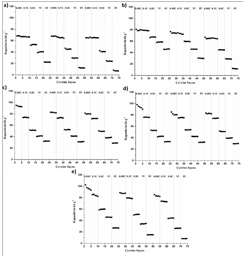
Şekil 4.46: Sol jel yöntemi ile sentezlenen 2-4 V voltaj aralığında a) \text{Na}_{0.5}\text{Mn}_{0.35}\text{Fe}_{0.35}\text{Co}_{0.3}\text{O}_2 b) \text{Na}_{0.6}\text{Mn}_{0.35}\text{Fe}_{0.35}\text{Co}_{0.3}\text{O}_2 c) \text{Na}_{0.7}\text{Mn}_{0.35}\text{Fe}_{0.35}\text{Co}_{0.3}\text{O}_2 d) \text{Na}_{0.8}\text{Fe}_{0.35}\text{Mn}_{0.35}\text{Co}_{0.3}\text{O}_2 e) \text{Na}_{0.9}\text{Fe}_{0.35}\text{Mn}_{0.35}\text{Co}_{0.3}\text{O}_2 numunelerine ait deşarj kapasitesinin akım yoğunluğu ile değişimi.
