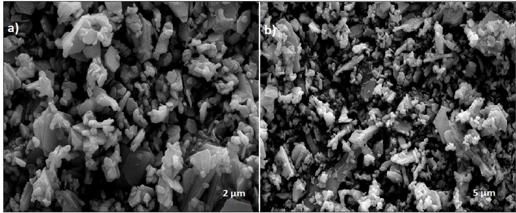
Şekil 4.36: Katı hal yöntemi ile sentezlenen P2 tipi \text{Na}_{0.6}\text{Mn}_{0.35}\text{Fe}_{0.35}\text{Co}_{0.3}\text{O}_2 bileşiğine ait a) 2 μm ve b) 5 μm taramalı elektron mikroskobu (SEM) görüntüleri.
