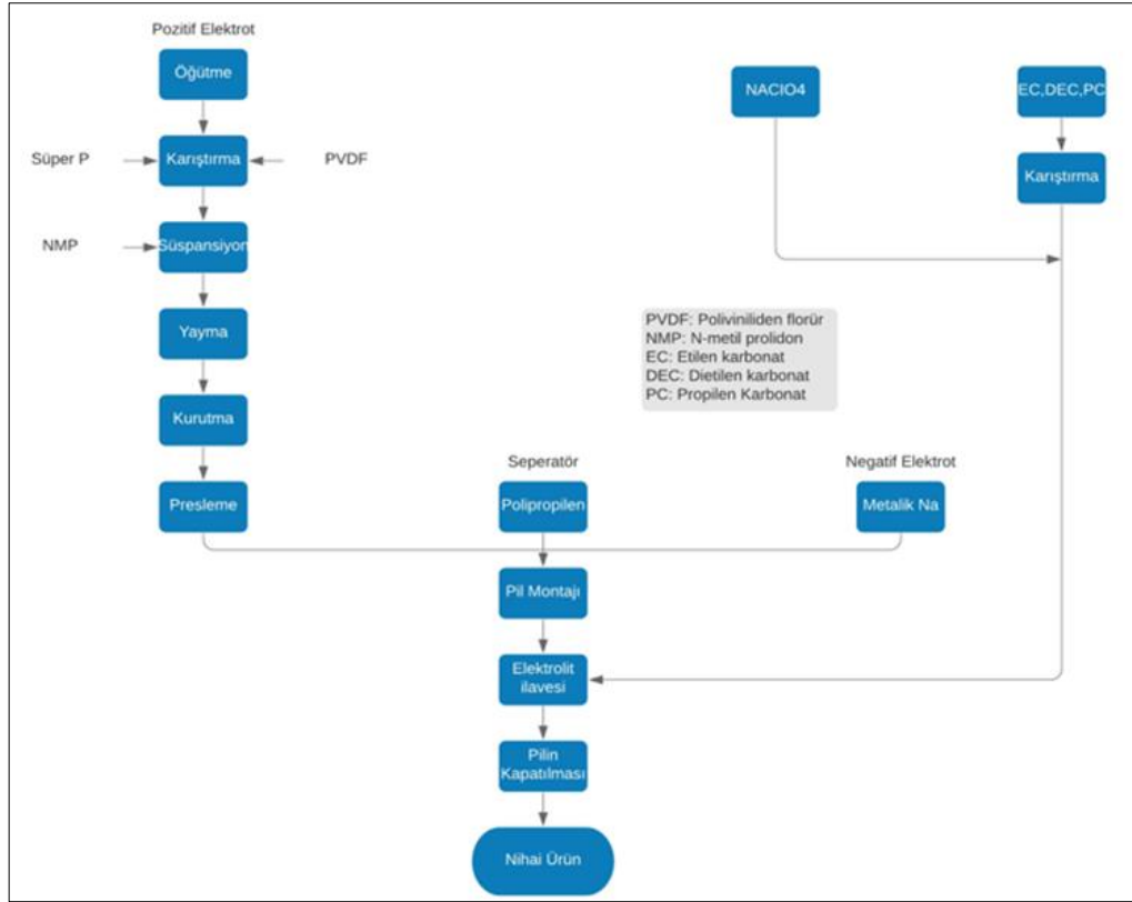
Şekil 3.3. Pil yapım basamakları.
