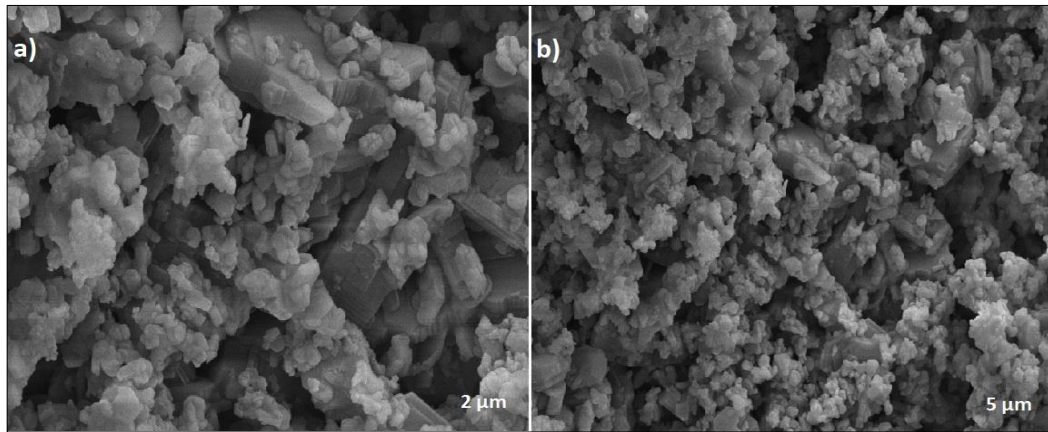
Şekil 4.61: Katı hal yöntemi ile sentezlenen K_{0.05}Na_{0.55}Mn_{0.35}Fe_{0.35}Co_{0.3}O_2 bileşiğine ait a) 2 \mu m ve b) 5 \mu m taramalı elektron mikroskobu (SEM) görüntüleri.
