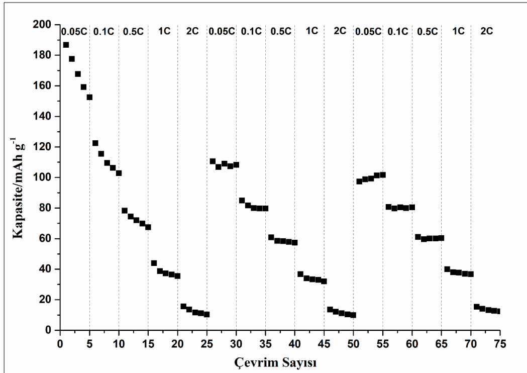
Şekil 4.9: Katı hal yöntemi ile sentezlenen \text{Na}_{0.7}\text{Fe}_{0.5}\text{Mn}_{0.5}\text{O}_2 maddesinin deşarj kapasitesinin akım yoğunluğu ile değişimi.
