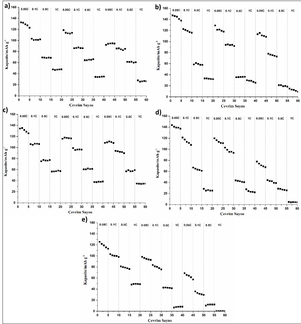
Şekil 4.48: Katı hal yöntemi ile sentezlenen 1.5-4 V voltaj aralığında a) Na 0.5 Mn 0.35 Fe 0.35 Co 0.3 O 2 b) Na 0.6 Mn 0.35 Fe 0.35 Co 0.3 O 2 c) Na 0.7 Mn 0.35 Fe 0.35 Co 0.3 O 2 d) Na 0.8 Mn 0.35 Fe 0.35 Co 0.3 O 2 e) Na 0.9 Mn 0.35 Fe 0.35 Co 0.3 O 2 numunelerine ait deşarj kapasitesinin akım yoğunluğu ile değişimi.
