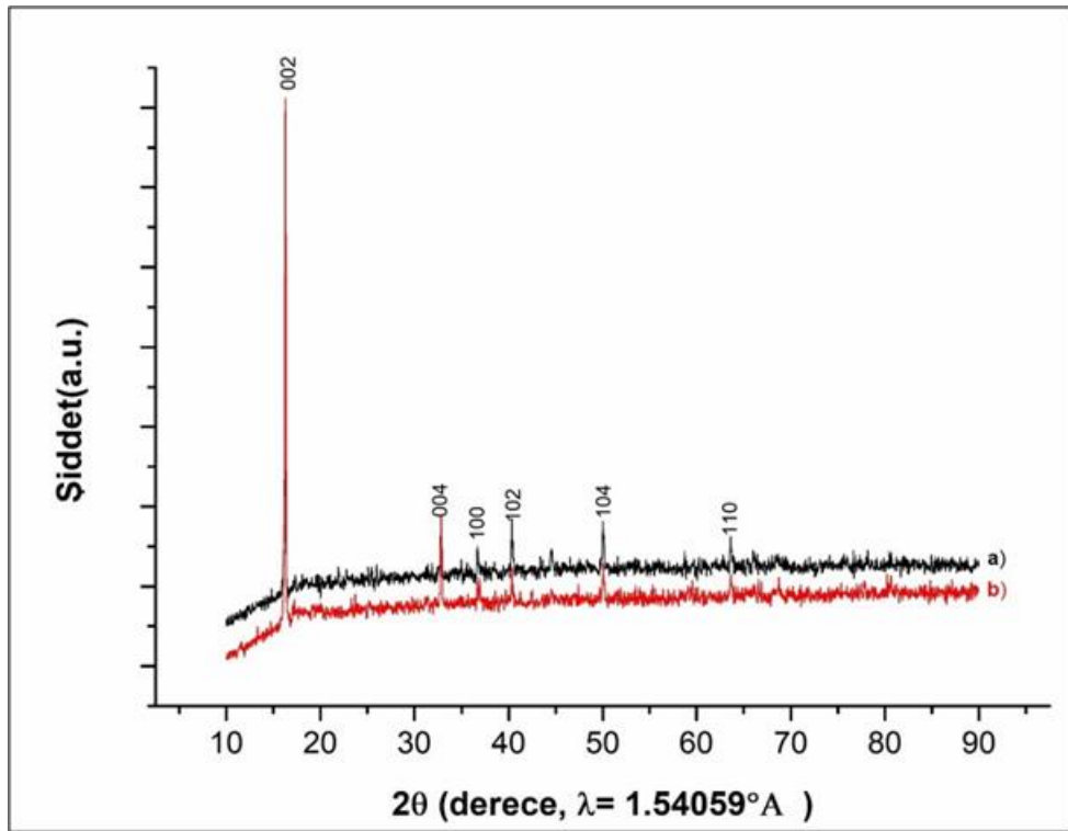
Şekil 4.1: a) Katı hal yöntemi ile sentezlenen ve b) sol-jel yöntemi ile sentezlenen \text{P2-Na}_{0.7}\text{CoO}_2 maddesinin XRD toz desenleri.
