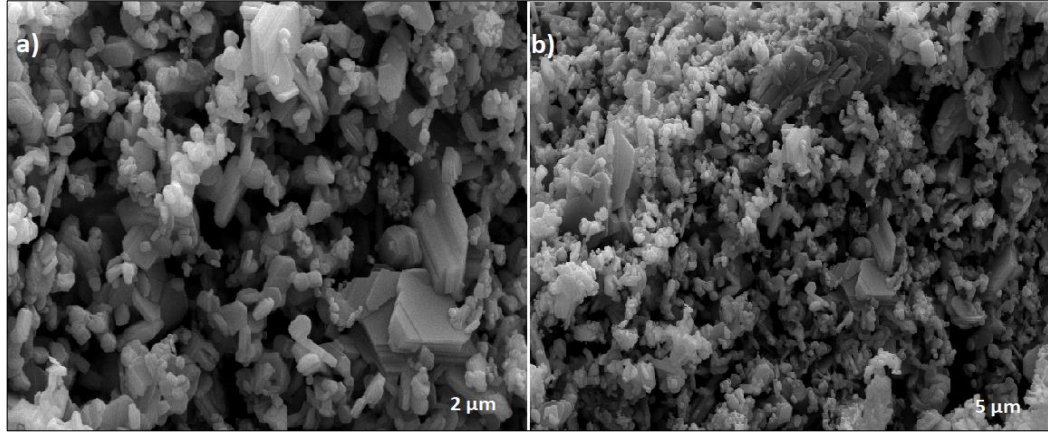
Şekil 4.59: Katı hal yöntemi ile sentezlenen K_{0.005}Na_{0.595}Mn_{0.35}Fe_{0.35}Co_{0.3}O_2 bileşiğine ait a) 2 \mu m ve b) 5 \mu m taramalı elektron mikroskobu (SEM) görüntüleri.
