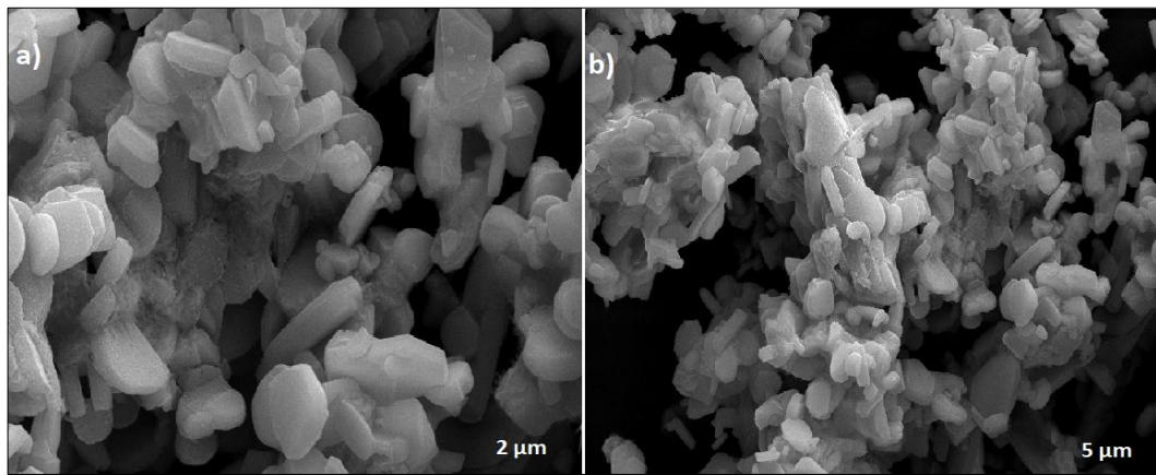
Şekil 4.63: Sol jel yöntemi ile sentezlenen K_{0.005}Na_{0.895}Mn_{0.35}Fe_{0.35}Co_{0.3}O_2 bileşiğine ait a) 2 \mu m ve b) 5 \mu m taramalı elektron mikroskobu (SEM) görüntüleri
