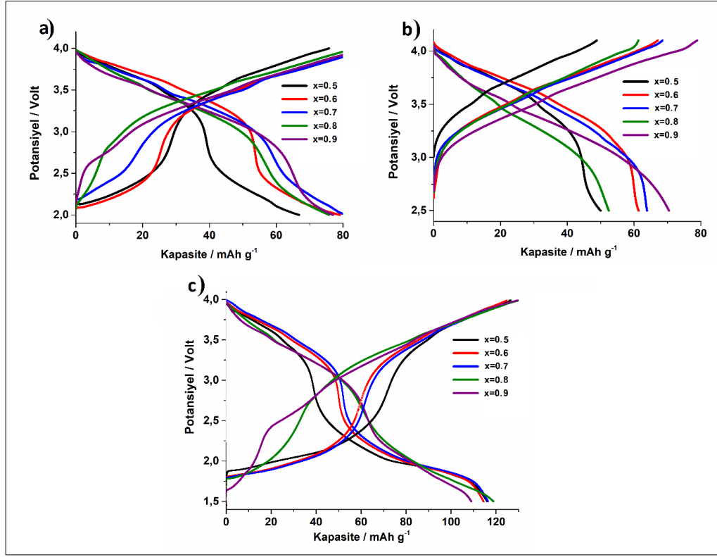
Şekil 4.40: \text{Na}_x(\text{Fe}_{0.35}\text{Mn}_{0.35}\text{Co}_{0.3})\text{O}_2 ( x = 0.5, 0.6, 0.7, 0.8, 0.9 ) numunelerinin a 2-4.0 V, b 2.5-4.1 V ve c 1.5-4 V potansiyel aralığında 0.1C akım yoğunluğunda ilk şarj/deşarj eğrileri.
