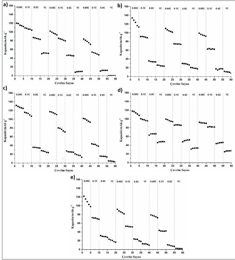
Şekil 4.81: Sol jel yöntemi ile sentezlenen 1.5-4.0 V voltaj aralığında a) \text{Na}_{0.9}\text{Mn}_{0.35}\text{Fe}_{0.35}\text{Co}_{0.3}\text{O}_2 b) \text{K}_{0.005}\text{Na}_{0.895}\text{Mn}_{0.35}\text{Fe}_{0.35}\text{Co}_{0.3}\text{O}_2 c) \text{K}_{0.01}\text{Na}_{0.89}\text{Mn}_{0.35}\text{Fe}_{0.35}\text{Co}_{0.3}\text{O}_2 d) \text{K}_{0.05}\text{Na}_{0.85}\text{Mn}_{0.35}\text{Fe}_{0.35}\text{Co}_{0.3}\text{O}_2 e) \text{K}_{0.1}\text{Na}_{0.8}\text{Mn}_{0.35}\text{Fe}_{0.35}\text{Co}_{0.3}\text{O}_2 numunelerine ait deşarj kapasitesinin akım yoğunluğu ile değişimi.
