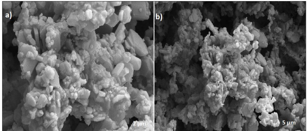
Şekil 4.58: Sol jel yöntemi ile sentezlenen K_{0.1}Na_{0.5}Mn_{0.35}Fe_{0.35}Co_{0.3}O_2 bileşiğine ait a) 2 \mu m ve b) 5 \mu m taramalı elektron mikroskobu (SEM) görüntüleri.
