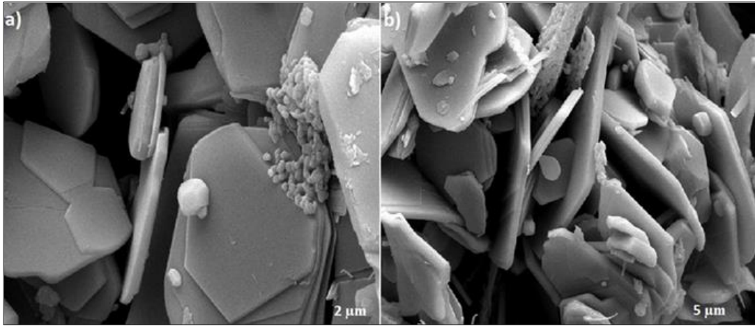
Şekil 4.2: Katı hal yöntemi ile sentezlenen \text{Na}_{0.7}\text{CoO}_2 bileşiğine ait a) 2 \mu\text{m} ve b) 5 \mu\text{m} SEM görüntüleri.
