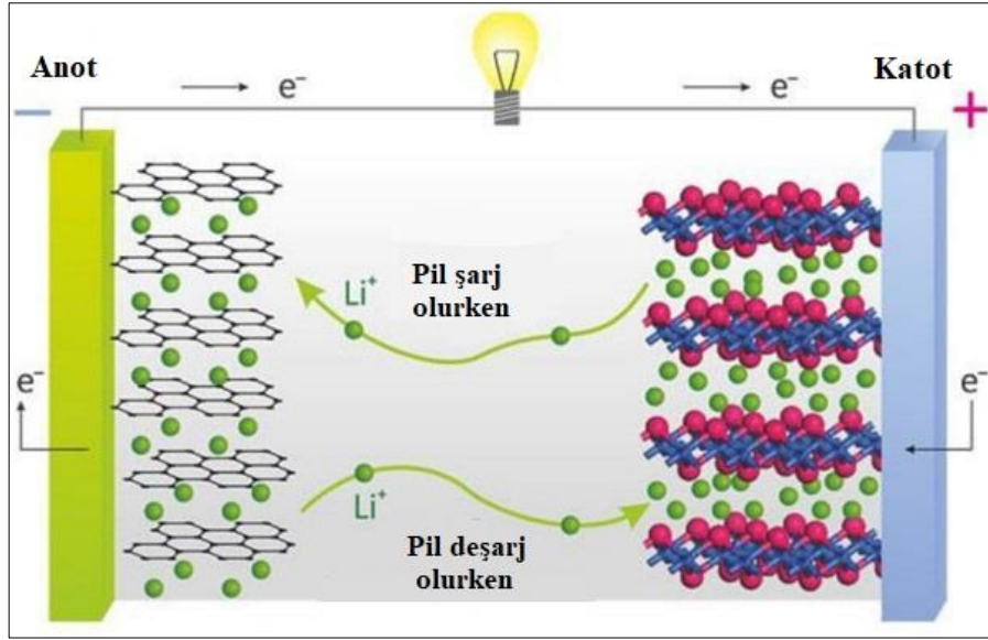
Şekil 2.6: Şarj edilebilir lityum iyon pillerde şarj/deşarj olayının şematik gösterimi.
