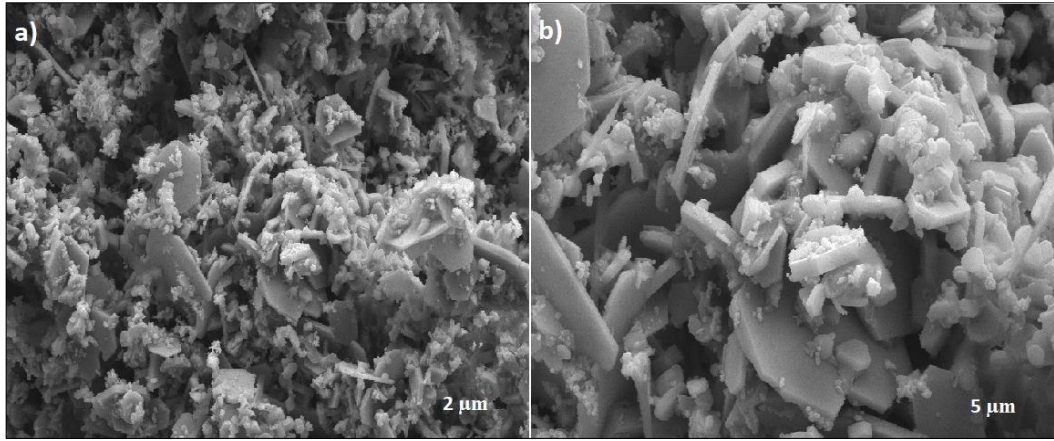
Şekil 4.17: Sol jel yöntemi ile sentezlenen \text{Na}_{0.7}\text{Mn}_{0.25}\text{Fe}_{0.25}\text{Co}_{0.5}\text{O}_2 bileşiğine ait a) 2 μm ve b) 5 μm SEM görüntüleri.
