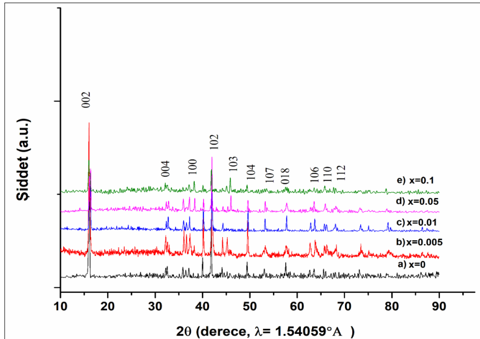
Şekil 4.53: Sol jel yöntemi ile sentezlenen a) Na_{0.9}Mn_{0.35}Fe_{0.35}Co_{0.3}O_2 b) K_{0.005}Na_{0.895}Mn_{0.35}Fe_{0.35}Co_{0.3}O_2 c) K_{0.01}Na_{0.89}Mn_{0.35}Fe_{0.35}Co_{0.3}O_2 d) K_{0.05}Na_{0.85}Mn_{0.35}Fe_{0.35}Co_{0.3}O_2 e) K_{0.1}Na_{0.8}Mn_{0.35}Fe_{0.35}Co_{0.3}O_2 maddelerinin XRD toz desenleri.
