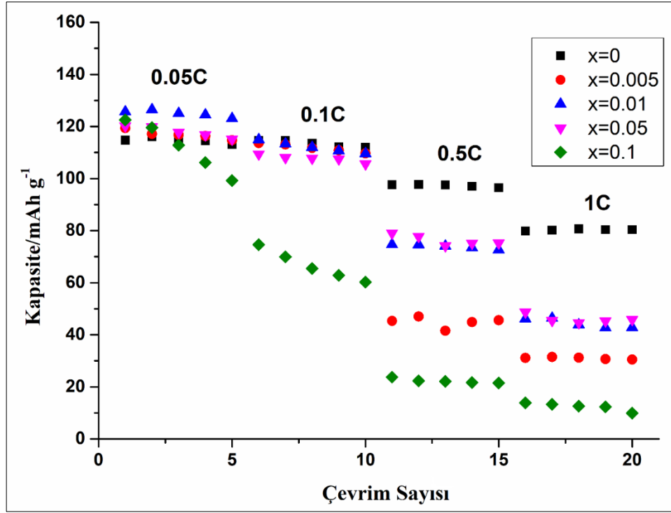
Şekil 4.76: Sol jel yöntemi ile sentezlenen 1.5-4.0 V gerilim aralığında K_xNa_{0.6-x}Mn_{0.35}Fe_{0.35}Co_{0.3}O_2 ( x = 0, 0.005, 0.01, 0.05, 0.1 ) katot aktif malzemelerin farklı C hızlarında hız kapasiteleri.
