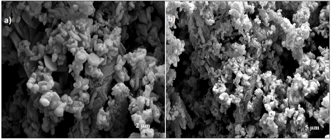
Şekil 4.20: Katı hal yöntemi ile sentezlenen \text{Na}_{0.7}\text{Mn}_{0.35}\text{Fe}_{0.35}\text{Co}_{0.3}\text{O}_2 bileşiğine ait a) 2 \mu\text{m} ve b) 5 \mu\text{m} SEM görüntüleri.
