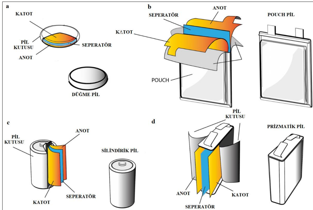
Şekil 2.5: a) Düğme, b) Pouch, c) Silindirik ve d) Prizmatik lityum iyon pilleri.
