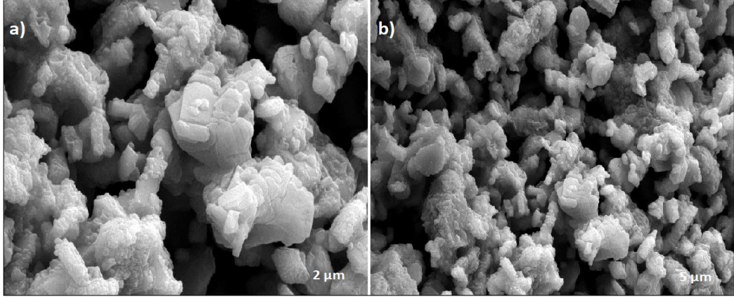
Şekil 4.67: Katı hal yöntemi ile sentezlenen K_{0.005}Na_{0.895}Mn_{0.35}Fe_{0.35}Co_{0.3}O_2 bileşiğine ait a) 2 \mu m ve b) 5 \mu m taramalı elektron mikroskobu (SEM) görüntüleri.
