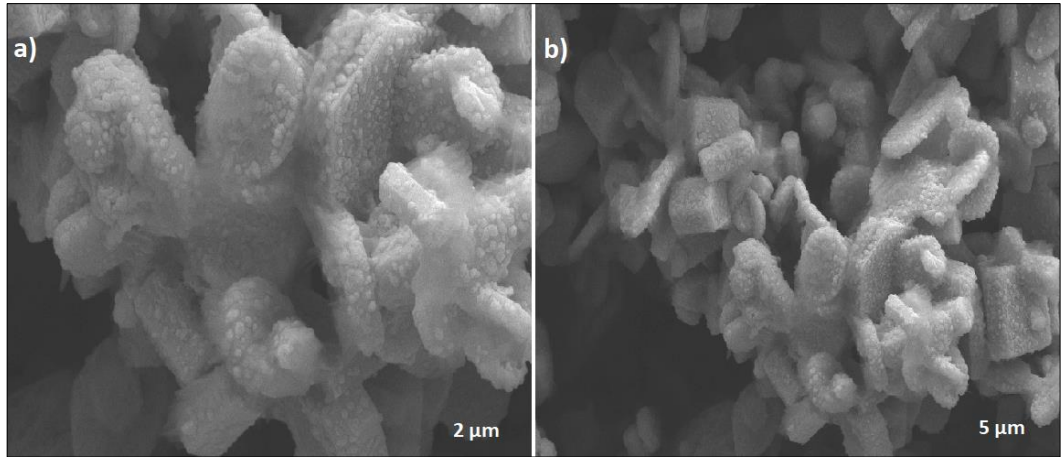
Şekil 4.33: Sol jel yöntemi ile sentezlenen \text{Na}_{0.8}\text{Mn}_{0.35}\text{Fe}_{0.35}\text{Co}_{0.3}\text{O}_2 bileşiğine ait a) 2 μm ve b) 5 μm SEM görüntüleri.
