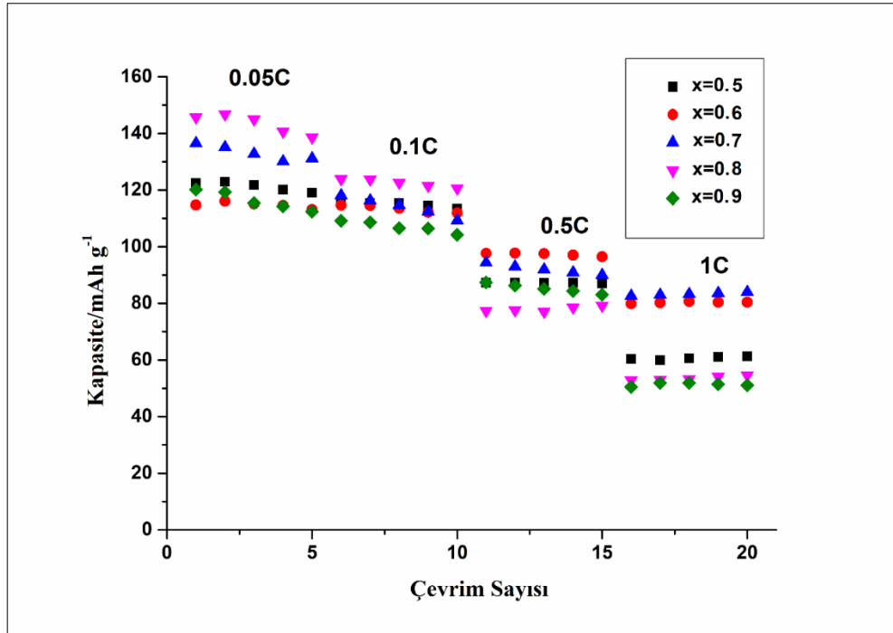
Şekil 4.42: Sol jel yöntemi ile sentezlenen 1.5-4.0 V gerilim aralığında \text{Na}_x(\text{Fe}_{0.35}\text{Mn}_{0.35}\text{Co}_{0.3})\text{O}_2 ( x = 0.5, 0.6, 0.7, 0.8, 0.9 ) katot aktif malzemelerin farklı C hızlarında hız kapasiteleri.
