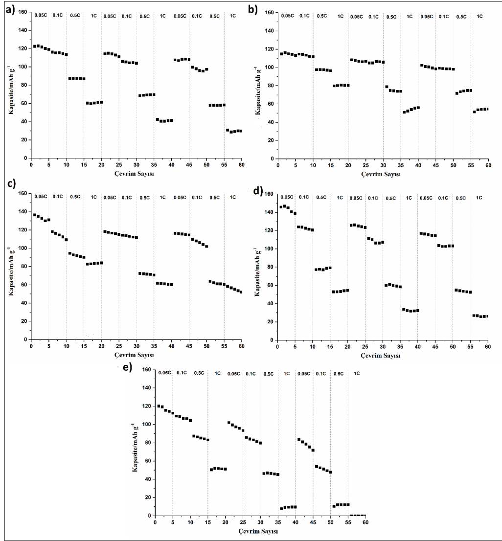
Şekil 4.43: Sol jel yöntemi ile sentezlenen 1.5-4 V voltaj aralığında a) \text{Na}_{0.5}\text{Mn}_{0.35}\text{Fe}_{0.35}\text{Co}_{0.3}\text{O}_2 b) \text{Na}_{0.6}\text{Mn}_{0.35}\text{Fe}_{0.35}\text{Co}_{0.3}\text{O}_2 c) \text{Na}_{0.7}\text{Mn}_{0.35}\text{Fe}_{0.35}\text{Co}_{0.3}\text{O}_2 d) \text{Na}_{0.8}\text{Fe}_{0.35}\text{Mn}_{0.35}\text{Co}_{0.3}\text{O}_2 e) \text{Na}_{0.9}\text{Fe}_{0.35}\text{Mn}_{0.35}\text{Co}_{0.3}\text{O}_2 numunelerine ait deşarj kapasitesinin akım yoğunluğu ile değişimi.
