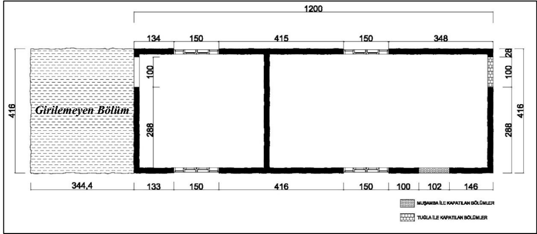
Şekil 5.6: Çerkes konut kültürünü yansıtan konutun plan şeması.
