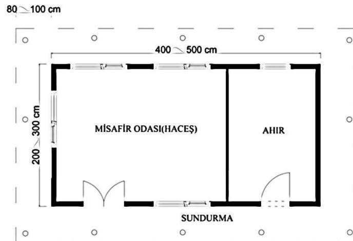
Şekil 7.4: Misafir Odası Modülü.
