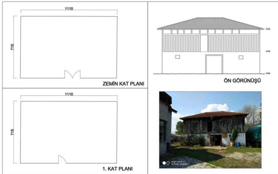
Şekil 5.12: Yığma + ahşap karkas taşıyıcı sistemi olan ahır ve kuruluk örneği.
