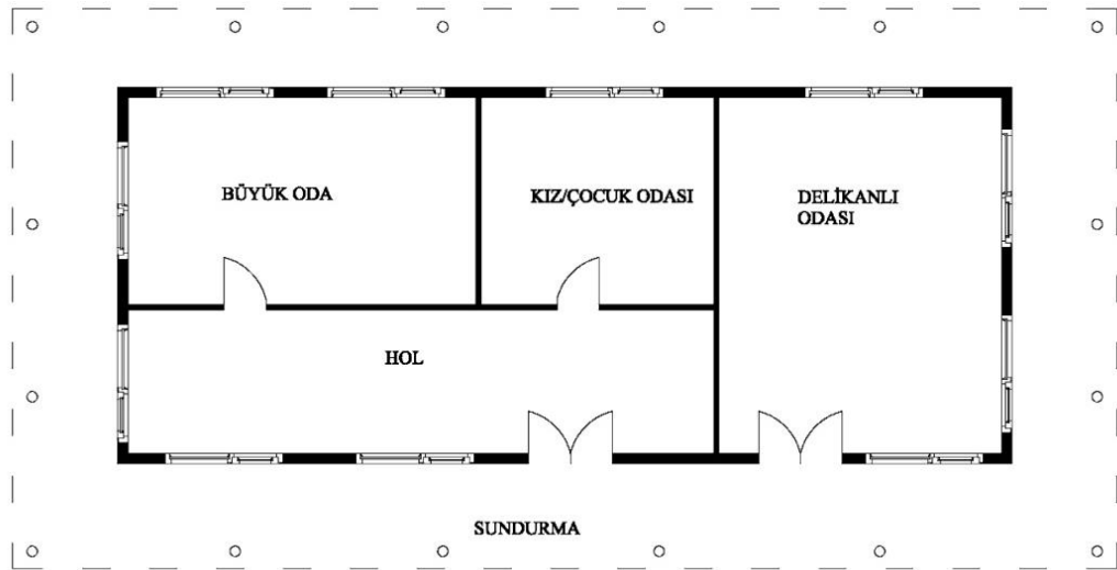
Şekil 4.5: “Çerkes Geleneği Kitabı”ndaki betimlemeler referans alınarak hazırlanmış büyük ev (Vune) Plan Şeması.
