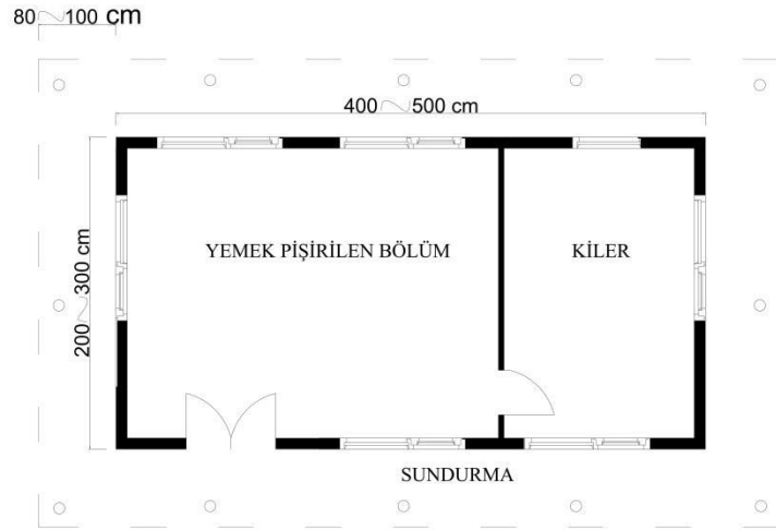
Şekil 7.3: Mutfak Modülü.
