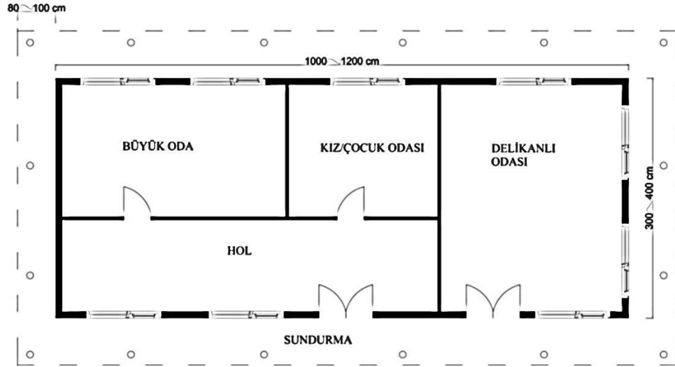
Şekil 7.2: Büyük Ev Modülü.
