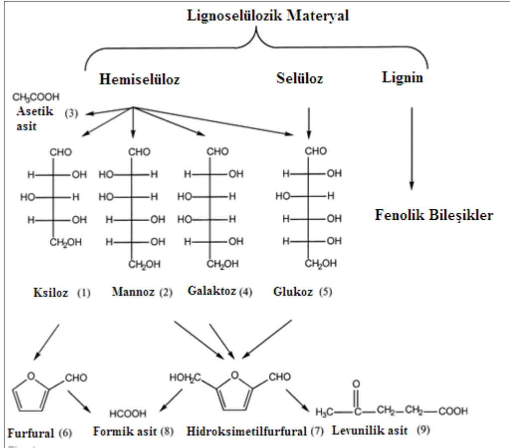
Şekil 2.5: Lignoselülozik materyallerin asit hidroliziyle açığa çıkan inhibitörler.
