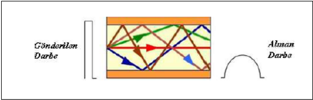
Şekil 4.11: Multimode fiber.
