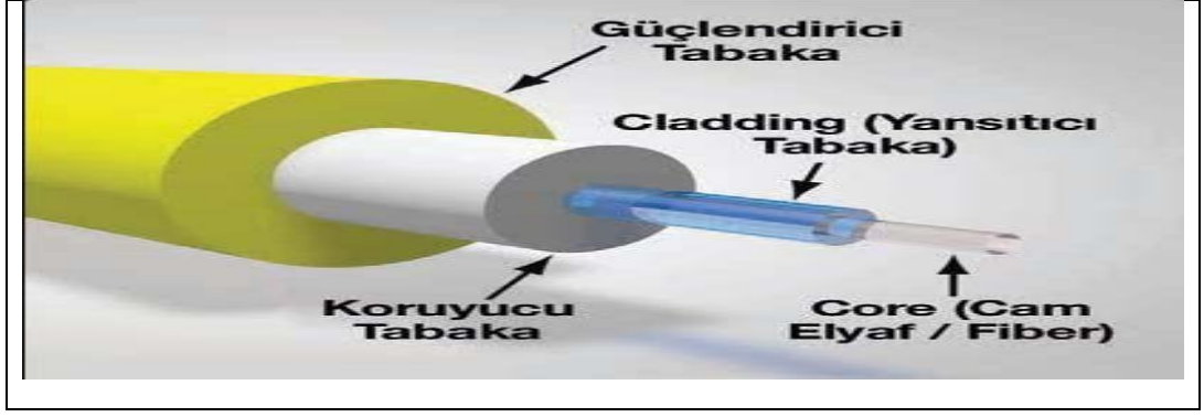
Şekil 4.4: Fiber optik kablo yapısı.
