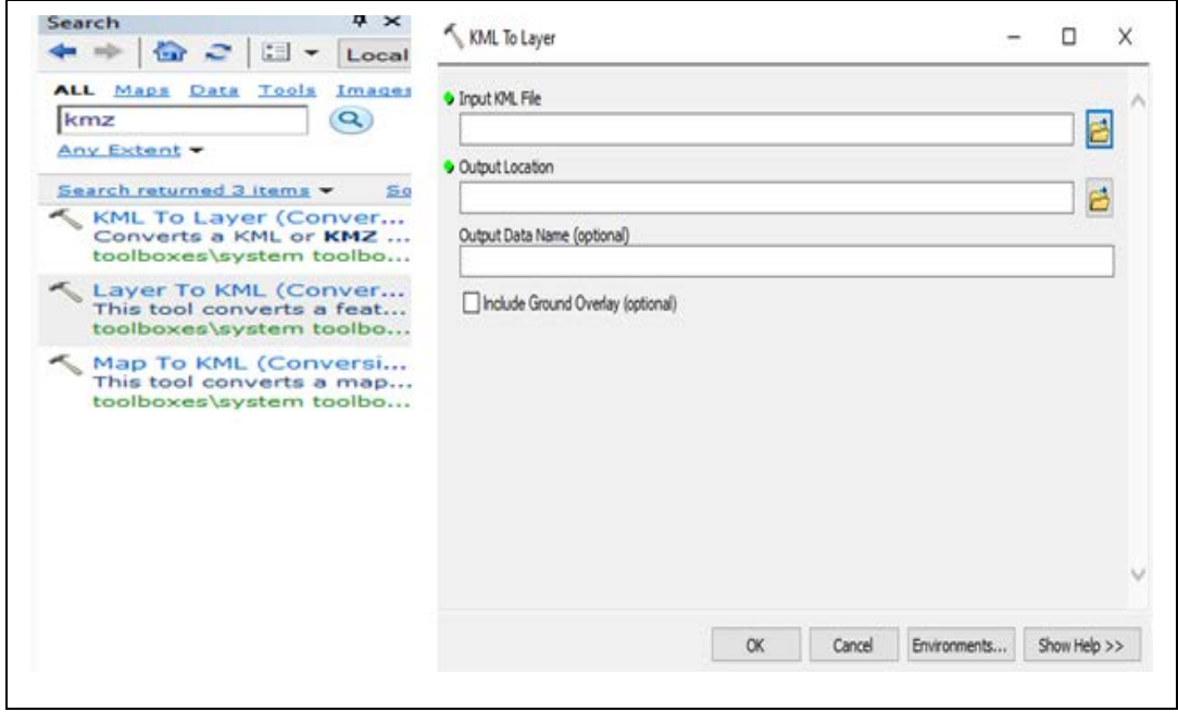
Şekil 5.16: KMZ dönüşümü.
