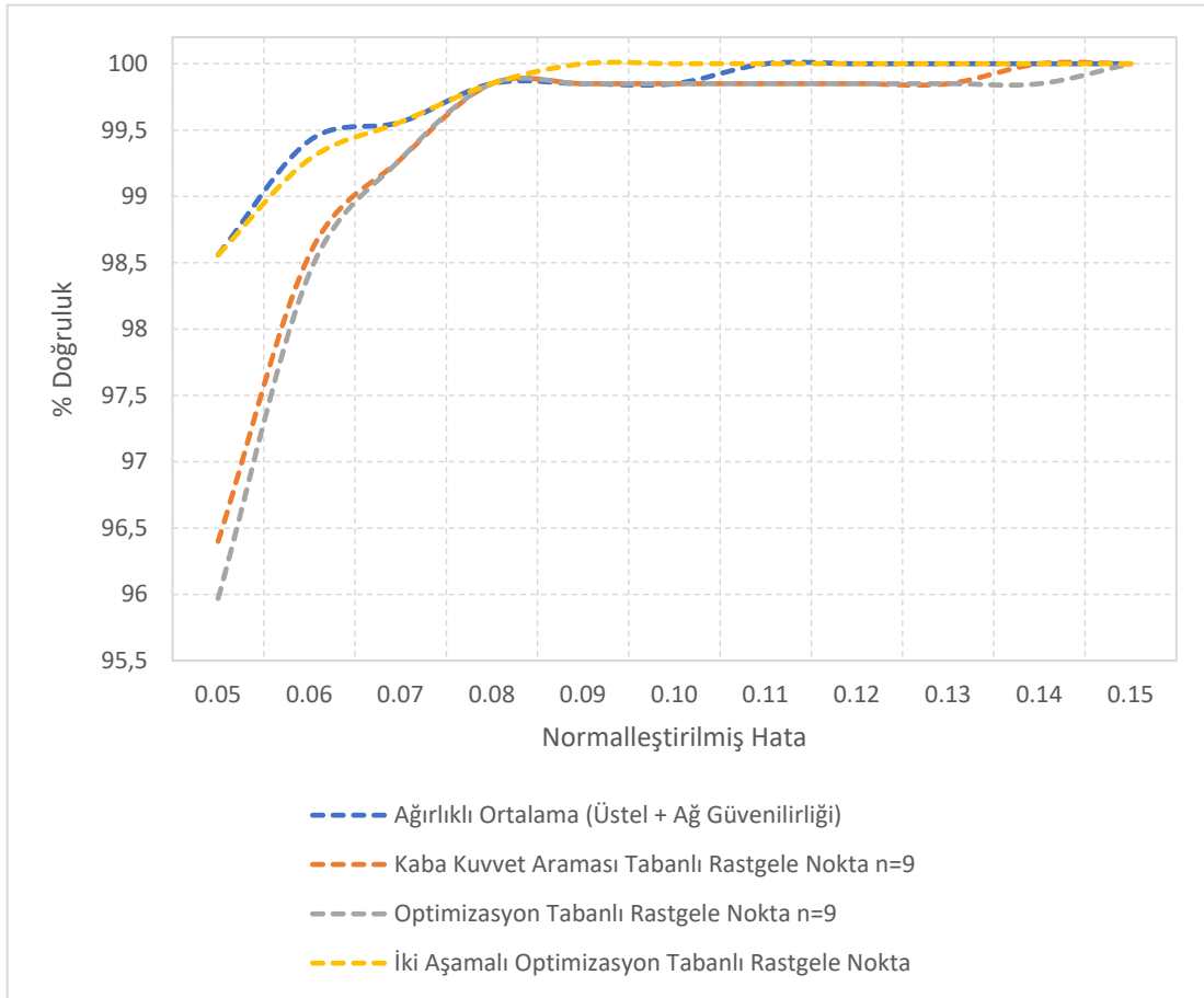
Şekil 5.6: Sistemin farklı test yöntemlerinin doğruluk oranına göre karşılaştırılması.
