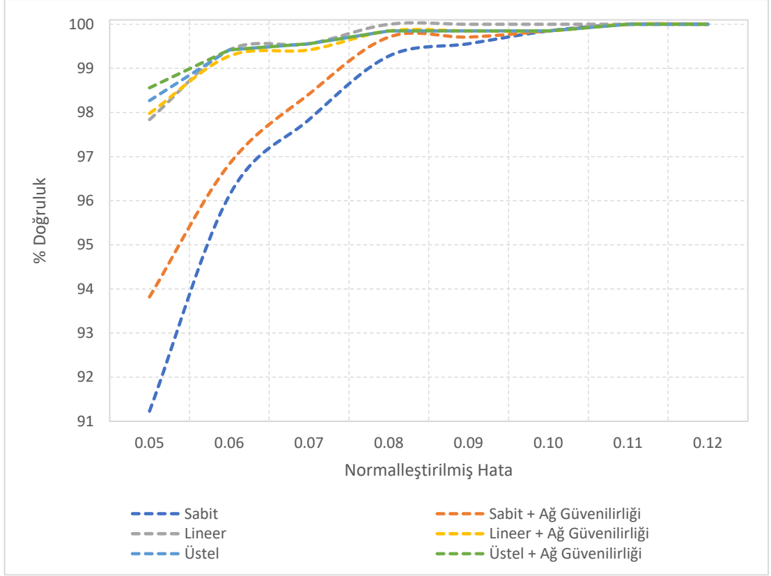
Şekil 5.2: Ağırlıklı ortalama yönteminin farklı parametrelerle gerçekleştirilen deney sonuçlarının karşılaştırılması.
