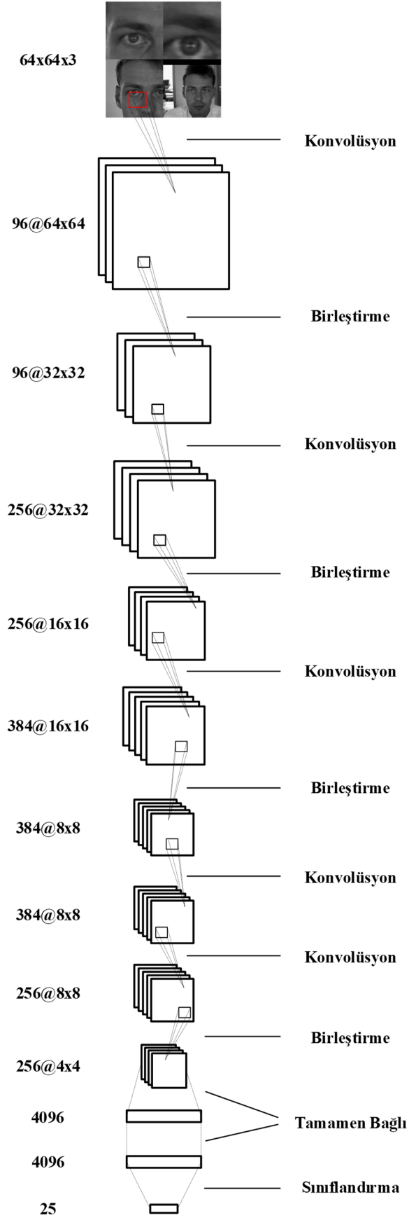
Şekil 3.4: Sistemin eğitiminde kullanılan ağ yapısı.
