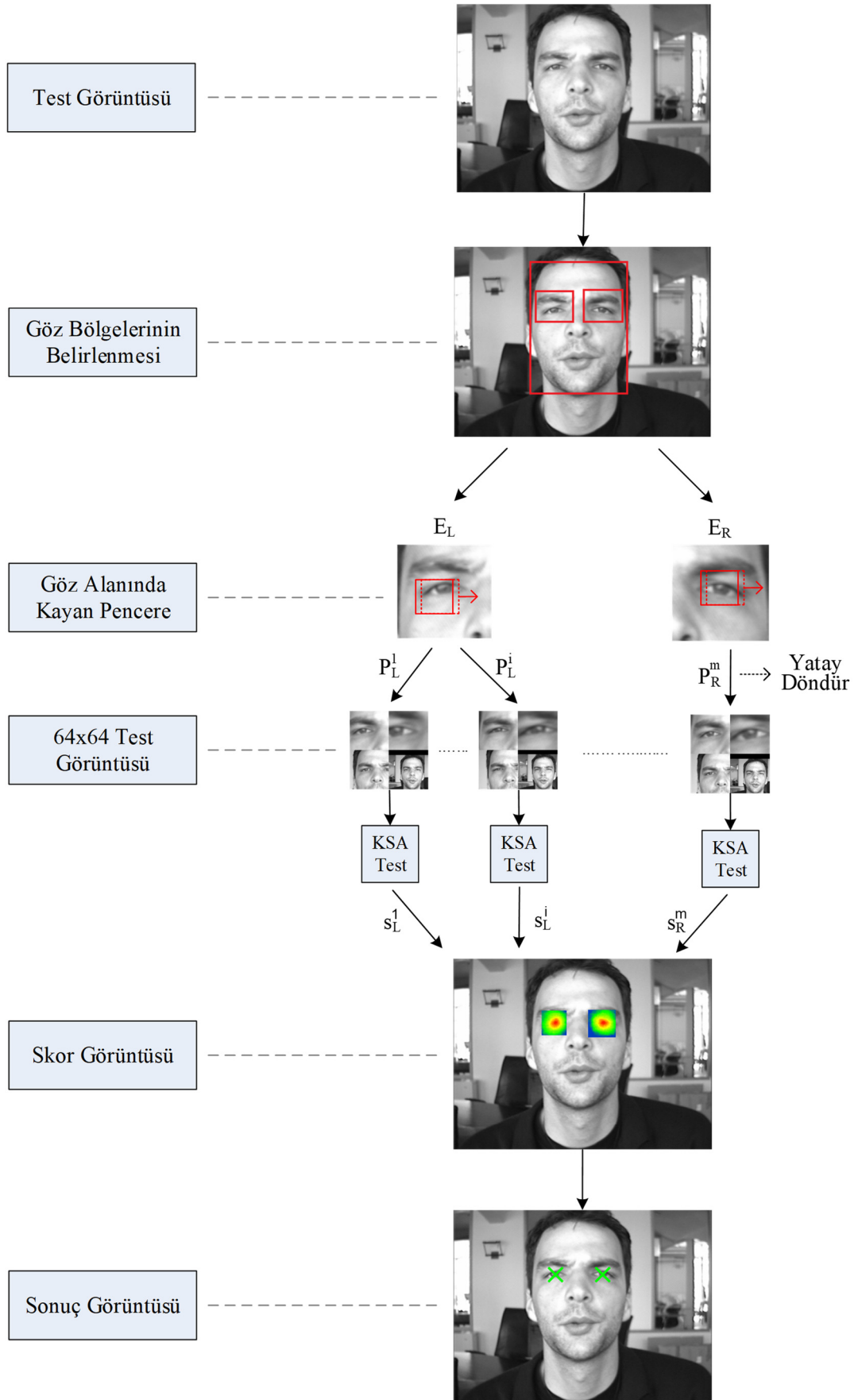
Şekil 4.1: Sistemin ağırlıklı ortalama yöntemi ile çalışan test aşaması.
