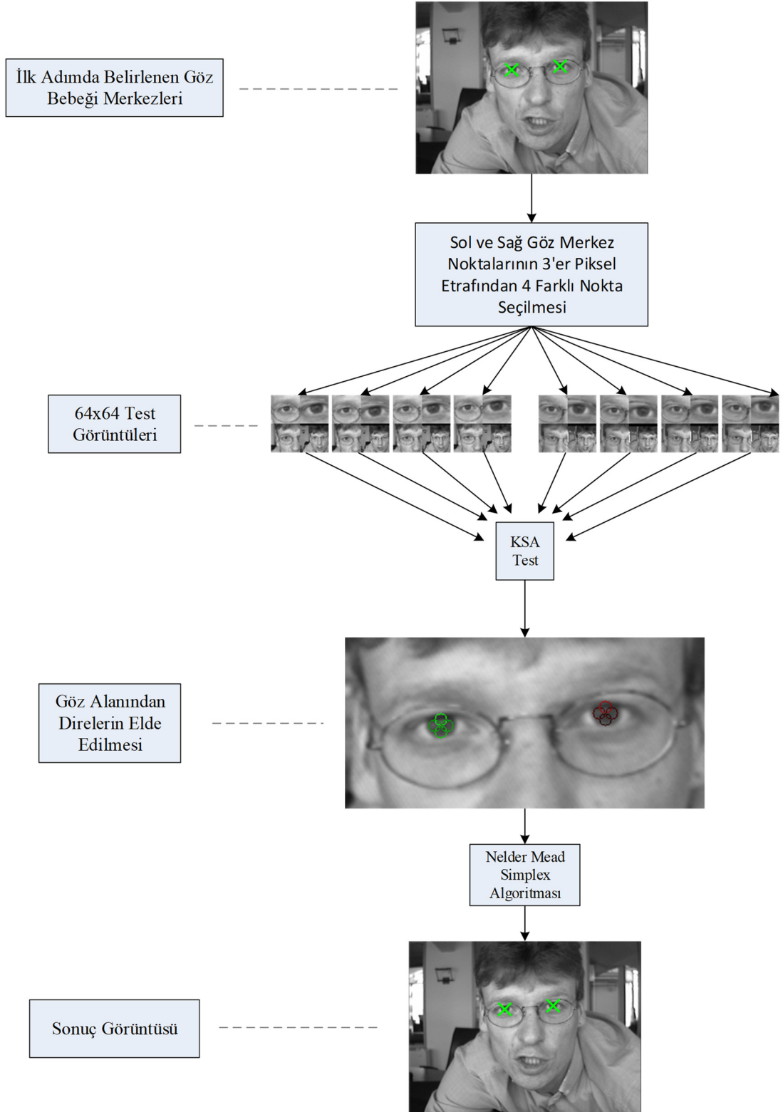
Şekil 4.7: Sistemin iki aşamalı optimizasyon tabanlı rastgele nokta yöntemi ile çalışan test aşamasının ikinci aşaması.
