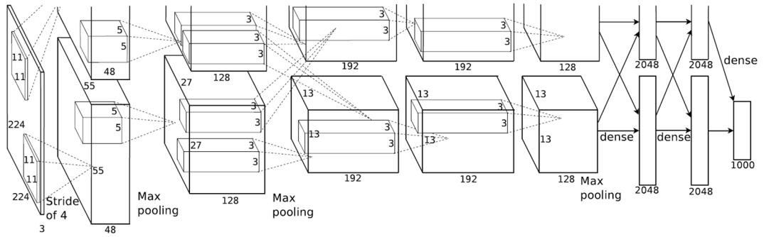
Şekil 3.3: AlexNet ağ yapısı.
