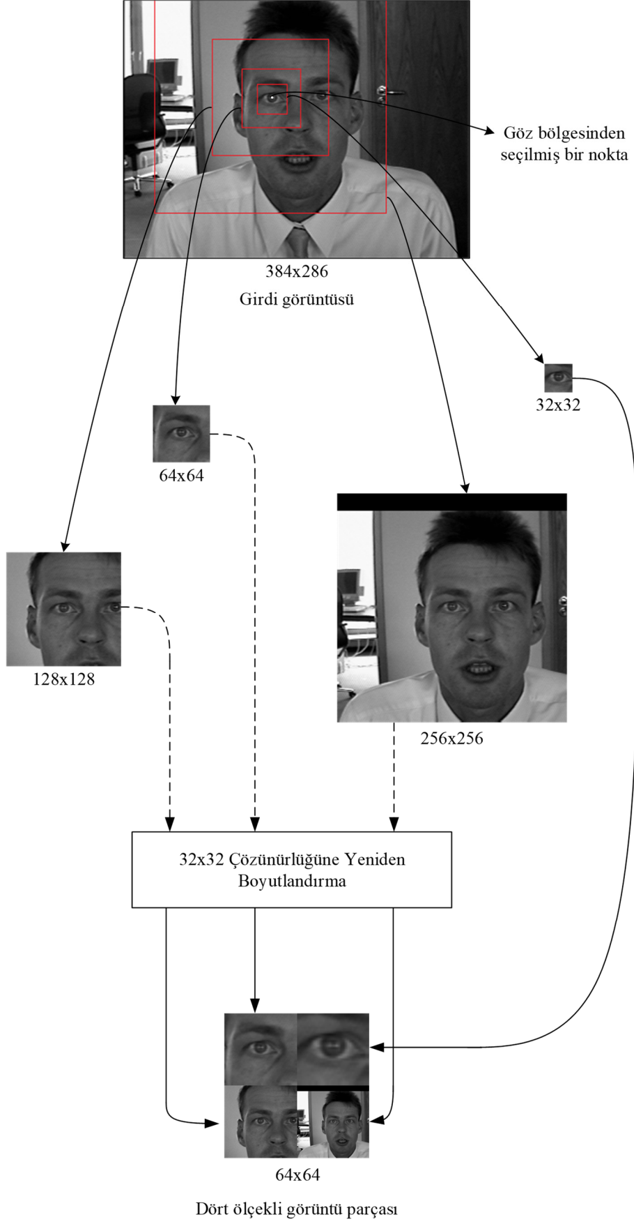
Şekil 3.2: Sıfır etiketi için dört ölçekli görüntü parçası elde etme aşamaları.
