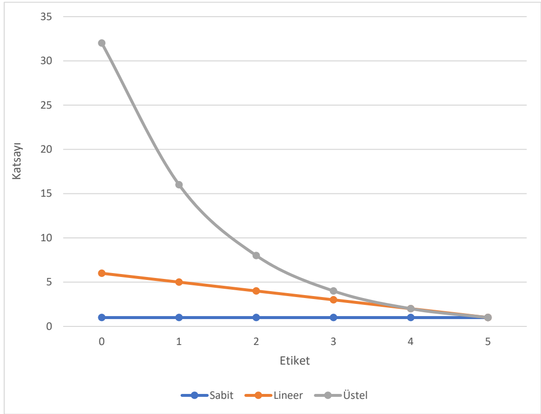
Şekil 4.2: Ağırlıklı ortalama yöntemi için farklı büyüme şekillerine göre etiket katsayı dağılımları.
