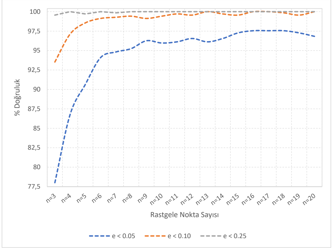
Şekil 5.4: Optimizasyon tabanlı rastgele nokta yöntemi için değişen n değerlerinde elde edilen başarı oranları.
