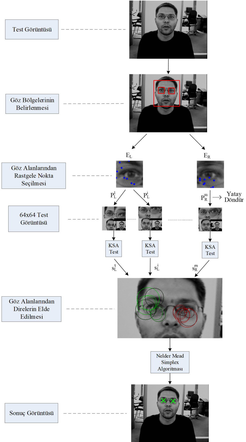
Şekil 4.5: Sistemin optimizasyon tabanlı rastgele nokta yöntemi ile çalışan test aşaması.
