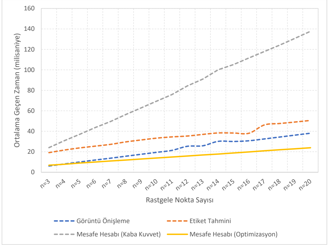
Şekil 5.3: Kaba kuvvet araması ve optimizasyon tabanlı rastgele nokta yöntemleri için her bir adımda n değişkenine göre ortalama geçen süreler.
