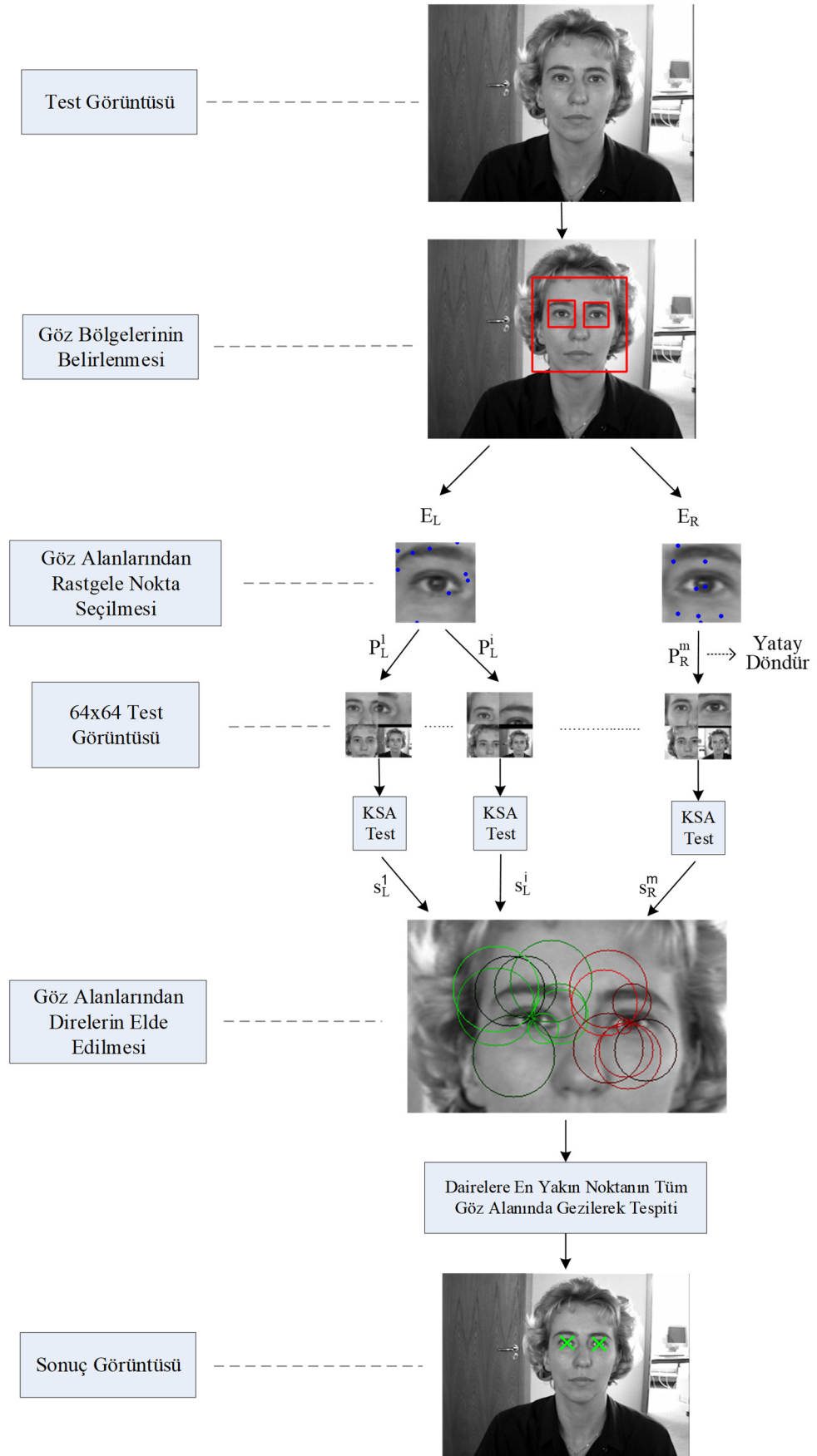
Şekil 4.3: Sistemin kaba kuvvet araması tabanlı rastgele nokta yöntemi ile çalışan test aşaması.
