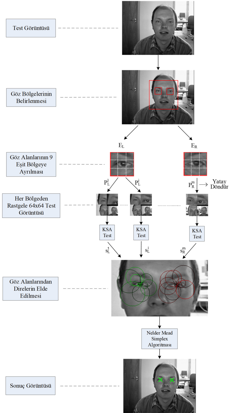
Şekil 4.6: Sistemin iki aşamalı optimizasyon tabanlı rastgele nokta yöntemi ile çalışan test aşamasının birinci aşaması.
