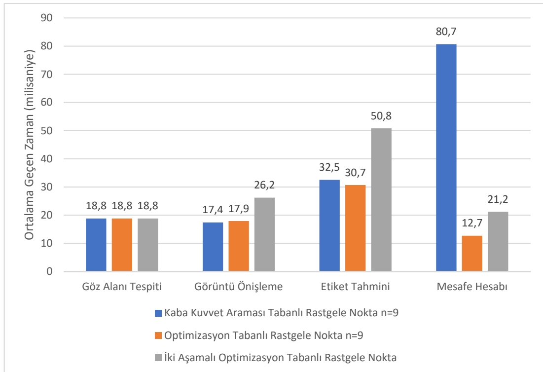
Şekil 5.5: Mesafe hesabı yapılan test yöntemlerinin her bir adımında ortalama geçen zamanın karşılaştırılması.
