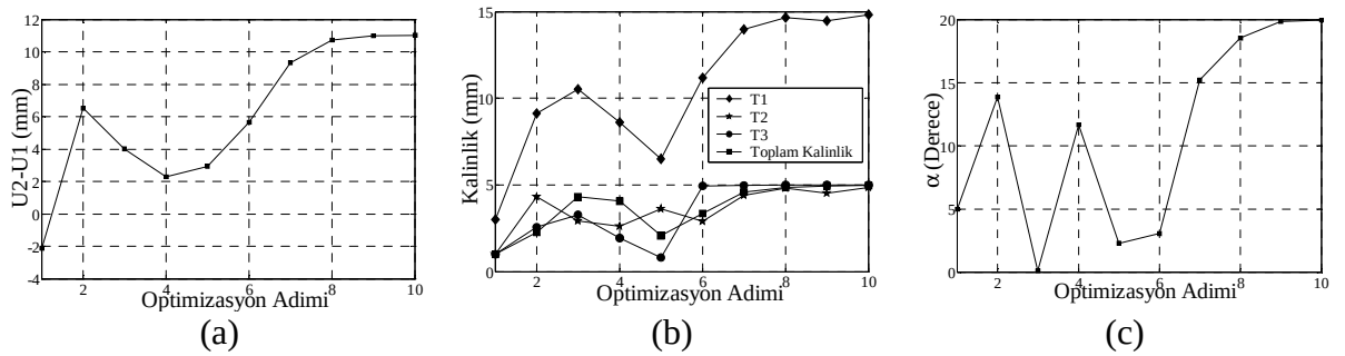
Şekil 7.8. (a) Yeni Başlangıç Değerleri için Amaç Fonksiyonunun, (b) Katman Kalınlıklarının, ve (c) Açının Optimizasyon Adımlarıyla Değişimi (Mermi Hızı 2000 m/s).
