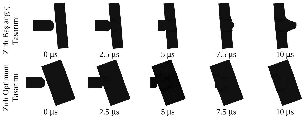
Şekil 7.4. 2000 m/s Hızla Hareket Etmekte Olan Bir Merminin Çarpmasına Maruz Kalan Bir Zırhın Başlangıç ve Optimum Tasarımlarının Deformasyonu.
