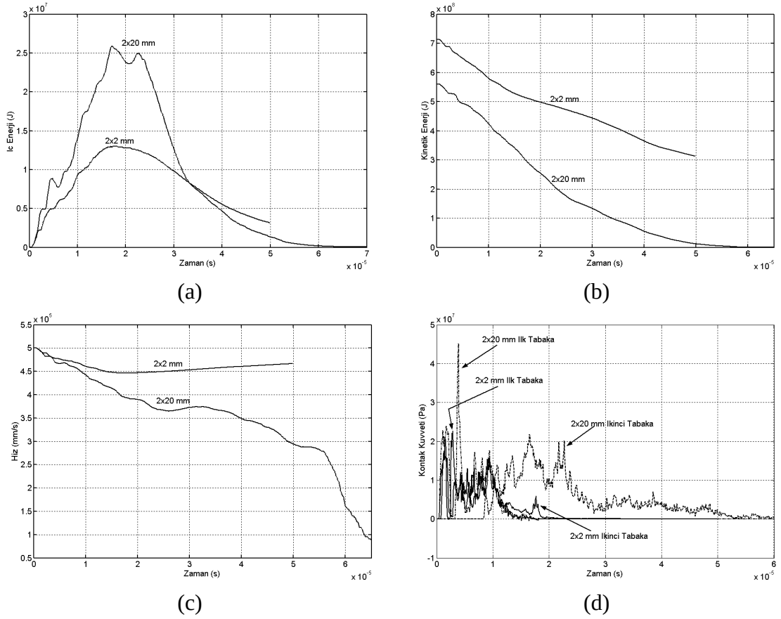
Şekil 5.8. Johnson-Cook Malzeme Modeli ile Çeşitli Kalınlıklarda Mermi için (a) İç Enerji, (b) Kinetik Enerji, (c) Mermi Hızı ve (d) Temas Kuvveti Değişimleri.
