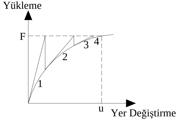
Şekil 1.4. Bir Yükleme Adımı için 4 İterasyonluk Tam Bir Newton-Raphson Analizi.
