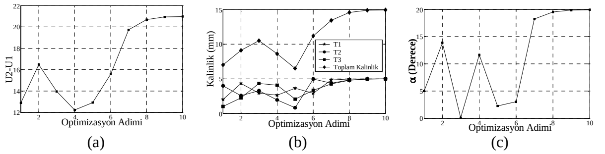
Şekil 7.1. (a) Amaç Fonksiyonunun, (b) Katman Kalınlıklarının, ve (c) Açının Optimizasyon Adımlarıyla Değişimi (Mermi Hızı 1000 m/s).
