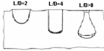
Şekil 4.5. Yarı Sonsuzluktaki Hedeflerde Çok Yüksek Hızlardaki Çarpma Karakteristikleri.
