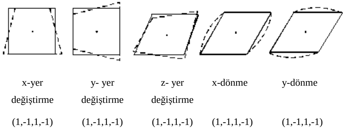
Şekil 2.4. Elemanlar için Kum Saati Modları.
