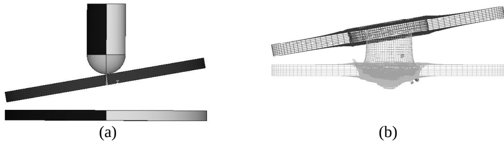
Şekil 5.9. (a) Birbirine 10^\circ Açıyla Duran Levhaların Geometrisi (b) Oluşan Hasar.
