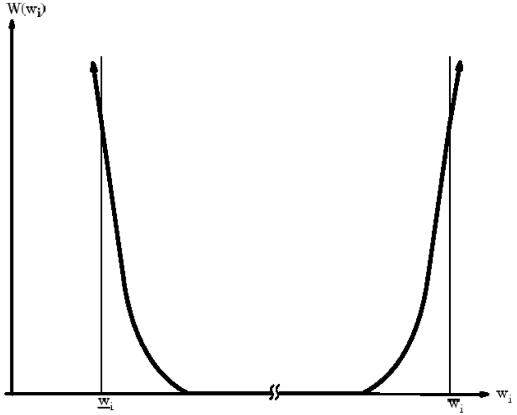
Şekil 3.3. Genişletilmiş Dahili Hata Fonksiyonlarının Durum Değişkenleri Uzayında Değişimleri.
