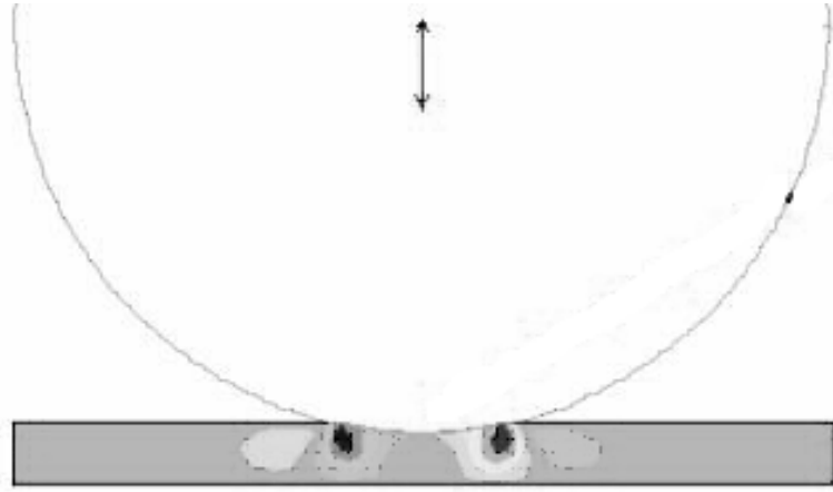
Şekil 1.13. İki Cismin Temasa Geçmesi ile Birlikte Gerilme Dağılımındaki Değişim.
