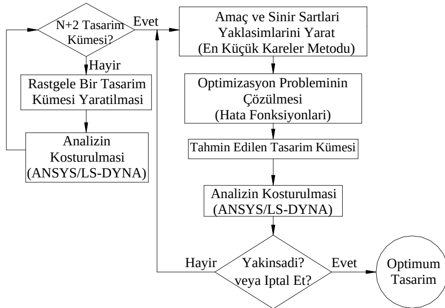
Şekil 6-1: ANSYS Tasarım Optimizasyonu Modülü ile Yaklaşık Optimizasyon Prosesi.
