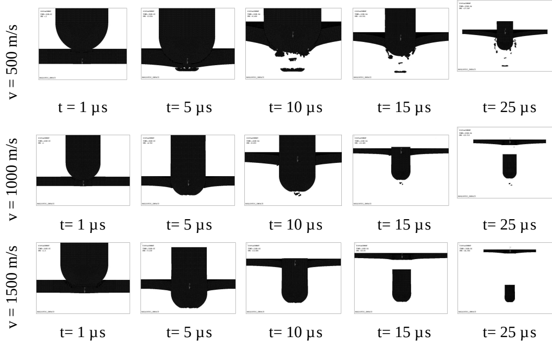
Şekil 5.3 . Plastik Kinematik Sertleşme Modeli ile Çeşitli Hızlarda Levhada Oluşan Hasar.
