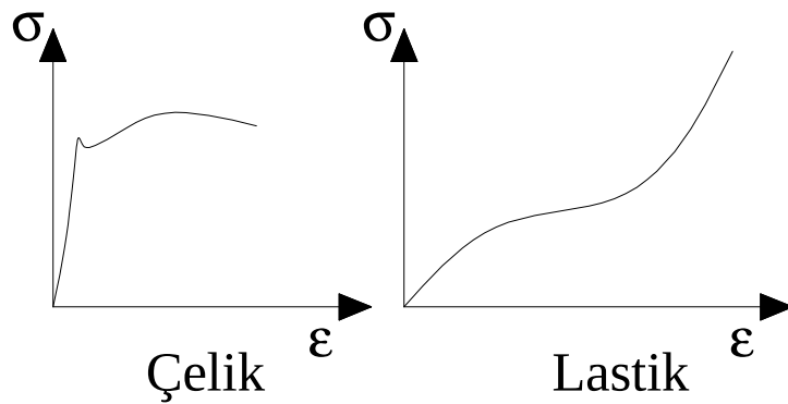
Şekil 1.12. Çelik ve Lastik için Gerilme-Gerinim Eğrileri.
