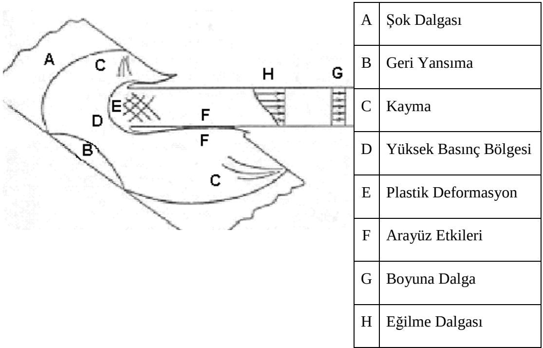
Şekil 4.2. Uzun Çubuk Penetrasyonu.
