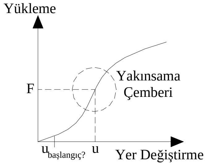
Şekil 1.7. Yakınsama Çemberi.
