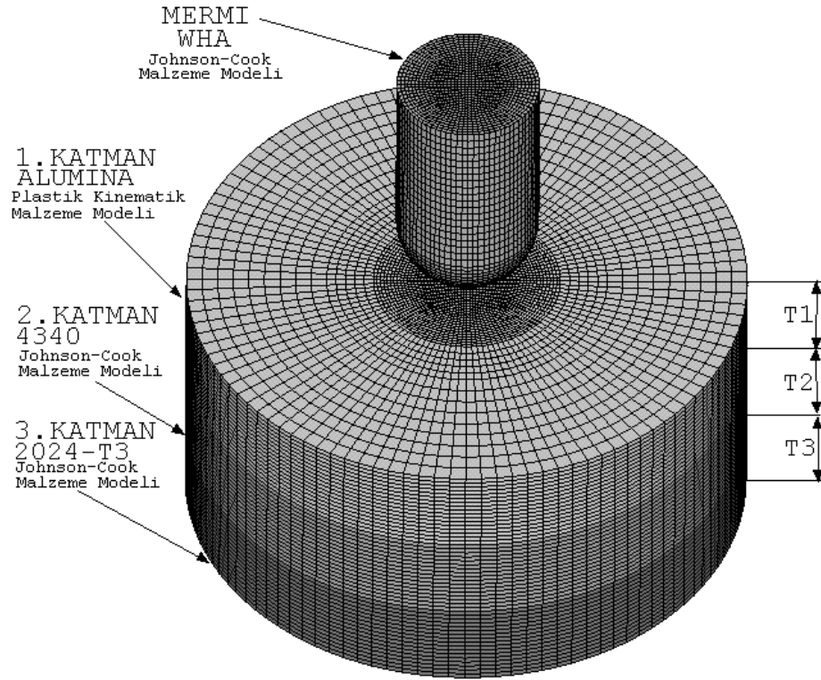
Şekil 6-2 : Zırhın ve Merminin Sonlu Elemanlar Modeli.
