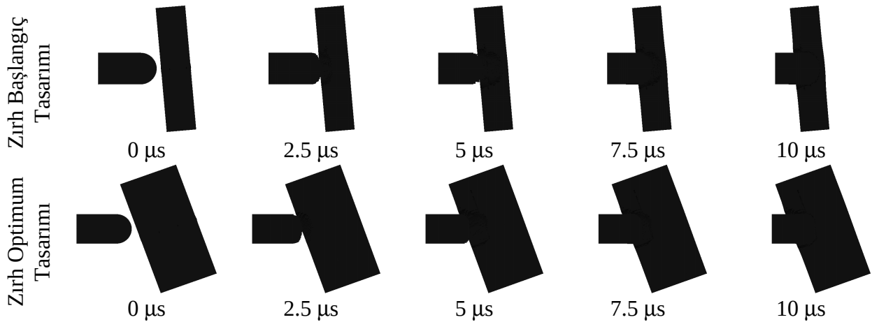
Şekil 7.2. 1000 m/s Hızla Hareket Etmekte Olan Bir Merminin Çarpmasına Maruz Kalan Bir Zırhın Başlangıç ve Optimum Tasarımlarının Deformasyonu.
