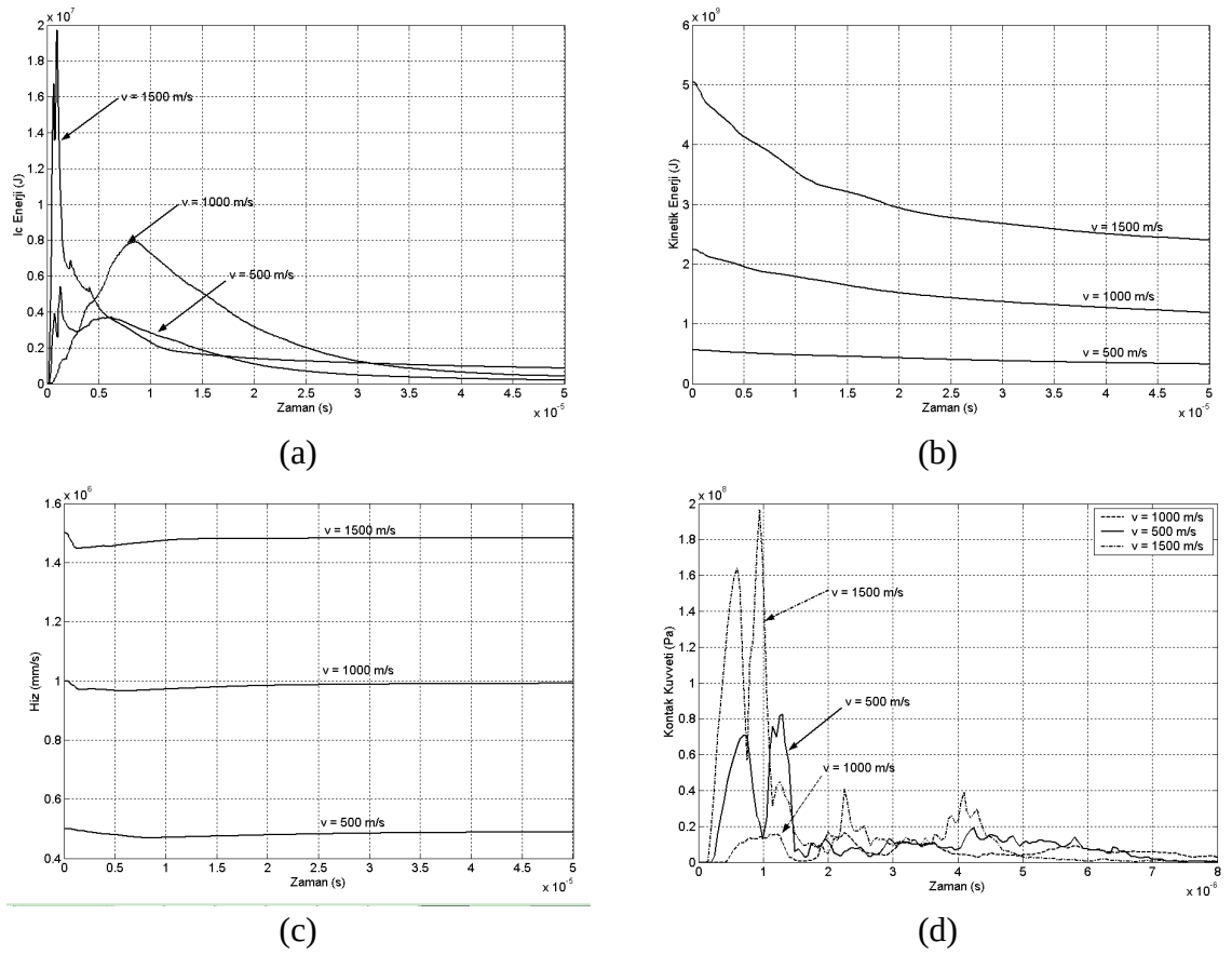
Şekil 5.6. Johnson-Cook Malzeme Modeli ile Çeşitli Hızlarda Mermi için (a) İç Enerji, (b) Kinetik Enerji, (c)Mermi Hızı ve (d) Temas Kuvveti Değişimleri.
