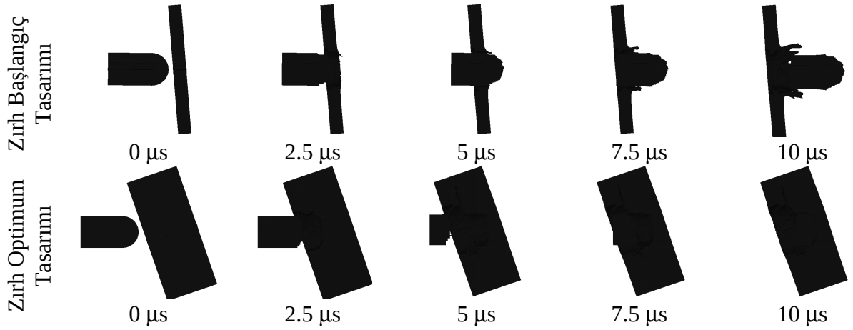
Şekil 7.9. Yeni Başlangıç Değerleri için 2000 M/S Hızla Hareket Etmekte Olan Bir Merminin Çarpmasına Maruz Kalan Bir Zırhın Başlangıç ve Optimum Tasarımlarının Deformasyonu.
