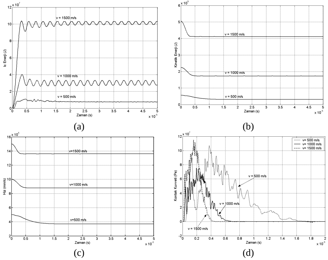
Şekil 5.4. Plastik Kinematik Sertleşme Modeli ile Çeşitli Hızlarda Mermi için (a) iç enerji, (b) Kinetik Enerji, (c) Mermi Hızı ve (d) Temas Kuvveti Değişimleri.
