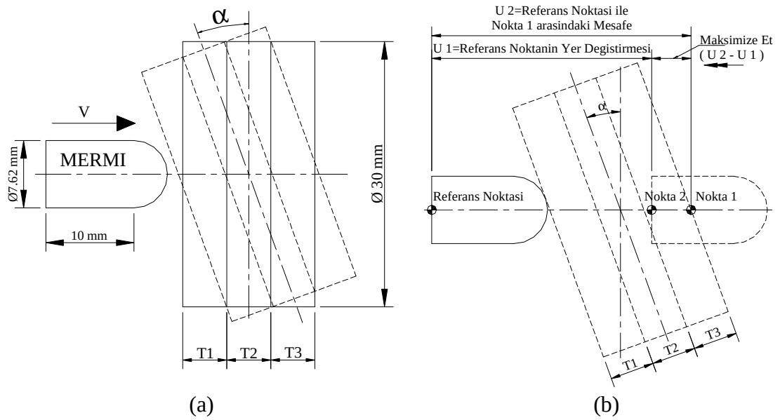
Şekil 6.3. (a) Tasarım Değişkenleri (b) Zırhta Penetrasyonun Ölçümü .
