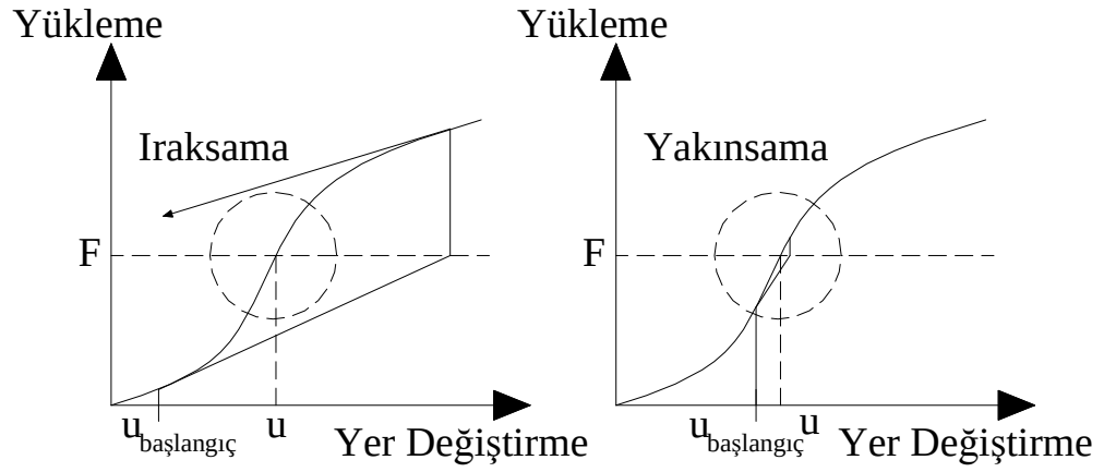
Şekil 1.8. Yakınsama ve Iraksamanın Başlangıç Noktası ile İlişkisi.
