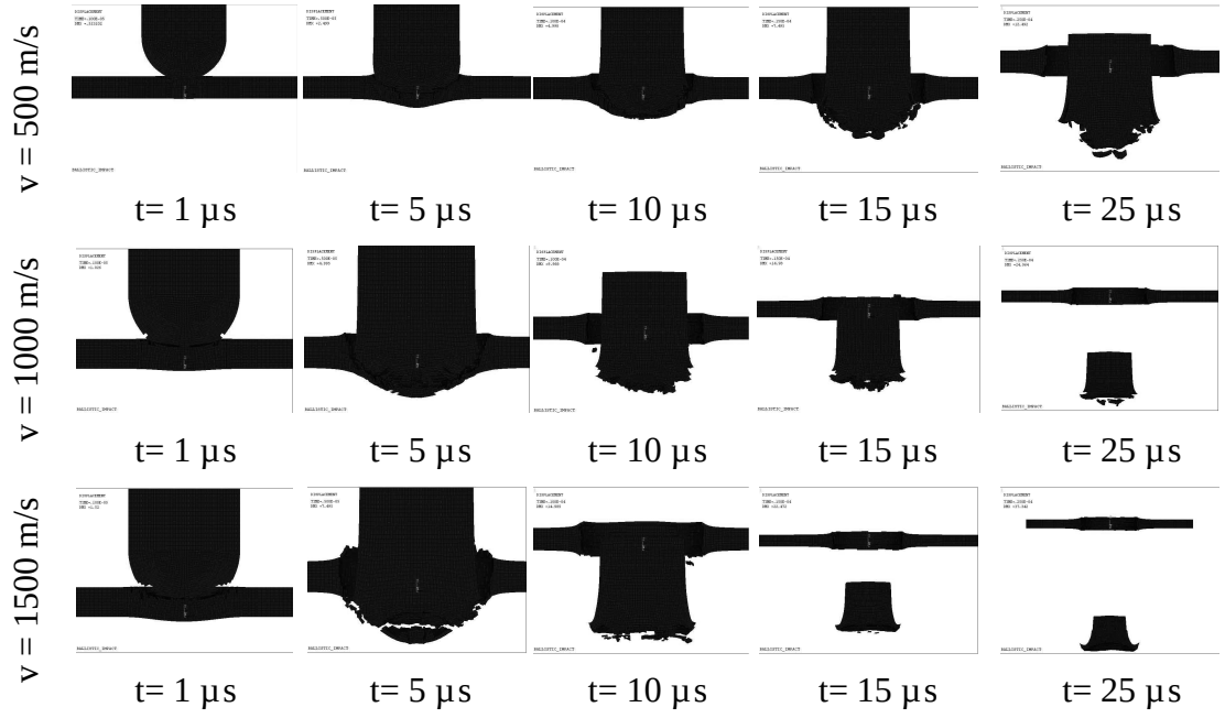
Şekil 5.5. Johnson-Cook Malzeme Modeli ile Çeşitli Hızlarda Levhada Oluşan Hasar.
