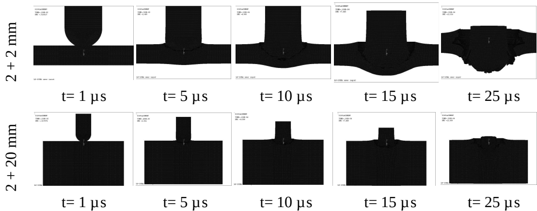
Şekil 5.7. Johnson-Cook Malzeme Modeli ile Çeşitli Kalınlıklar için Levhada Oluşan Hasar.
