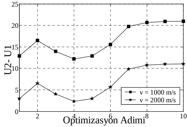
Şekil 7.5. Amaç Fonksiyonunun Çarpışma Hızı ile Değişimi.
