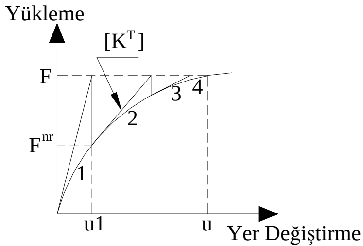
Şekil 1.5. Newton-Raphson Metodu ile Yakınsama.
