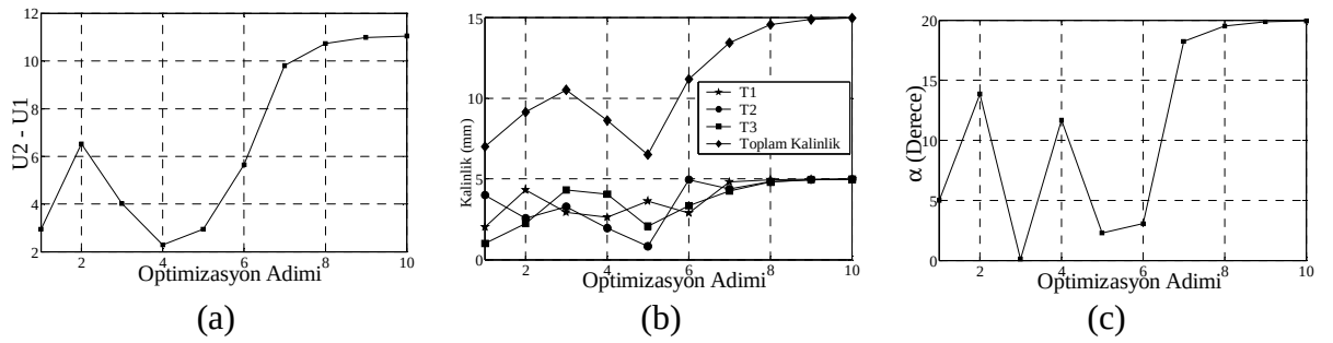
Şekil 7.3. (a) Amaç Fonksiyonunun, (b) Katman Kalınlıklarının, ve (c) Açının Optimizasyon Adımlarıyla Değişimi (Mermi Hızı 2000 m/s).
