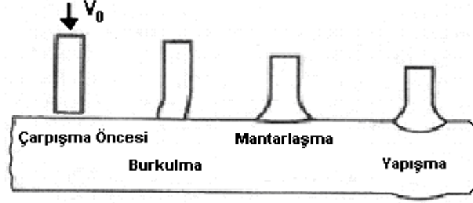
Şekil 4.4. Düşük Hızlardaki Çarpma Karakteristikleri.
