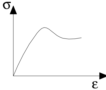
Şekil 1.3. Malzemedeki Doğrusal Olmayan Davranış.
