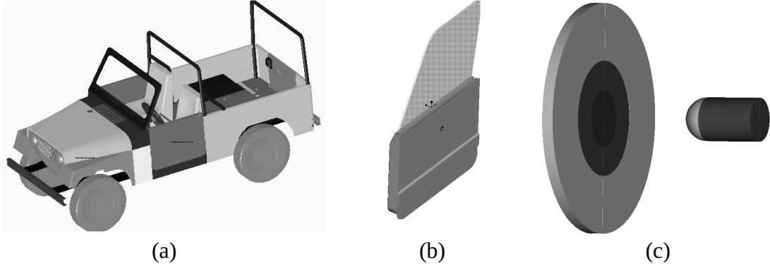
Şekil 5.1. (a) Araç Yandan Görünüşü, (b) Kapı (c) Kapı Üzerinde Dairesel Bir Kesit ve Mermi.
