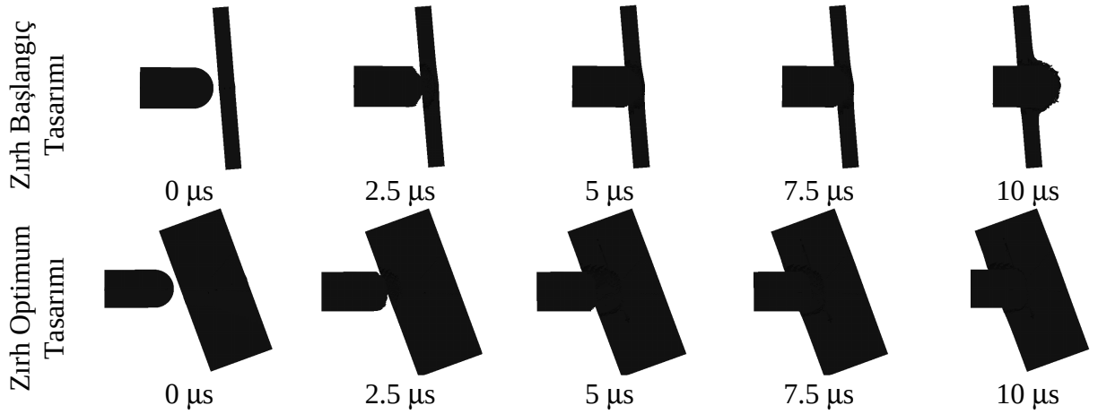
Şekil 7.7. Yeni Başlangıç Değerleri için 1000 M/S Hızla Hareket Etmekte Olan Bir Merminin Çarpmasına Maruz Kalan Bir Zırhın Başlangıç ve Optimum Tasarımlarının Deformasyonu.
