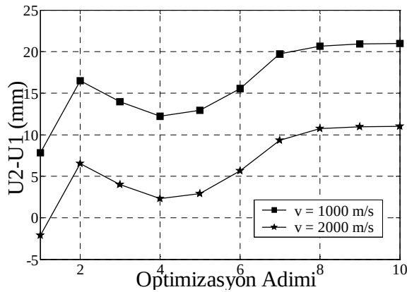
Şekil 7.10. Yeni Başlangıç Değerleri için Amaç Fonksiyonunun Çarpışma Hızı ile Değişimi.
