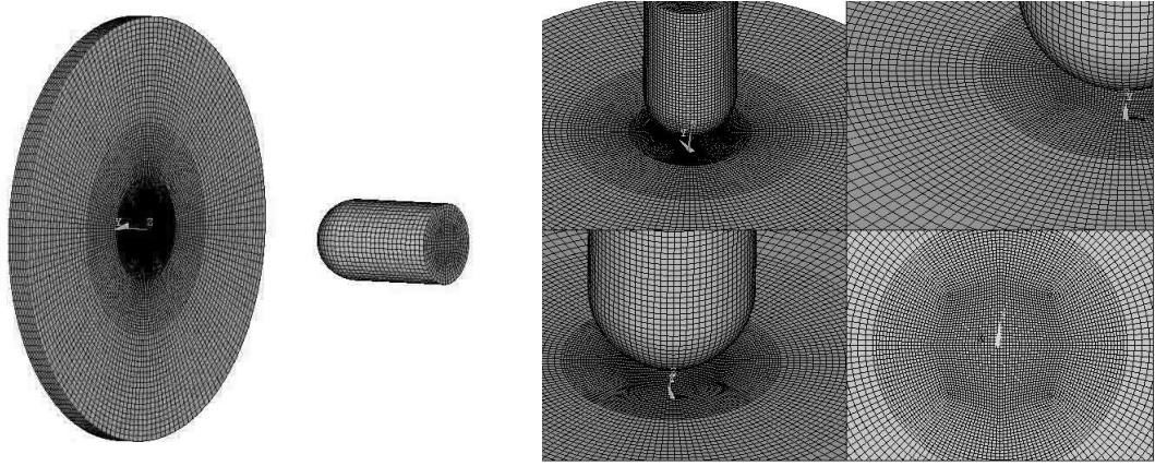
Şekil 5.2. Üzerinden Alınan Dairesel Kesit ve Merminin Sonlu Elemanlar Modeli.
