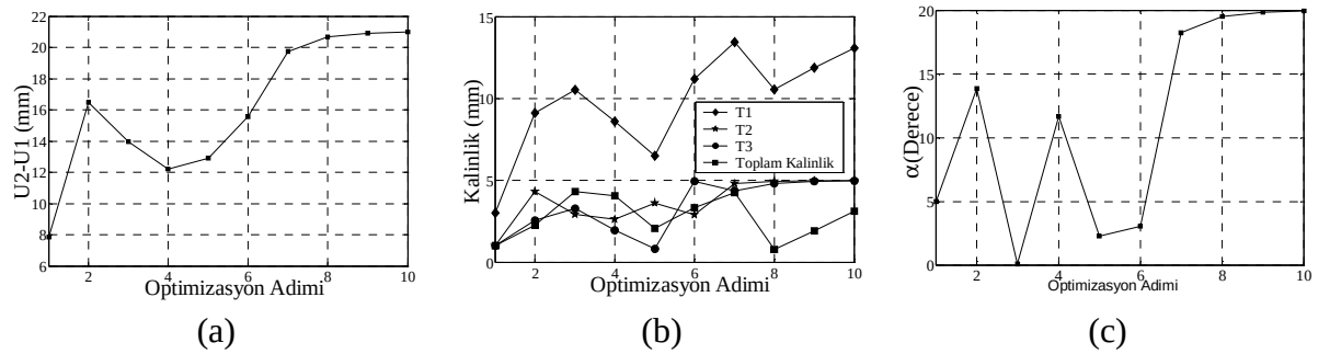
Şekil 7.6. (a) Yeni Başlangıç Değerleri için Amaç Fonksiyonunun, (b) Katman Kalınlıklarının, ve (c) Açının Optimizasyon Adımlarıyla Değişimi (Mermi Hızı 1000 m/s).
