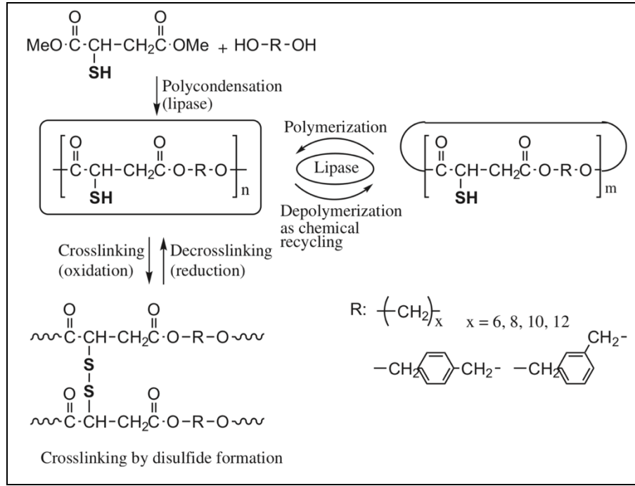
Şekil 2.19: Merkaptoları içeren poliesterin sentez reaksiyonu.
