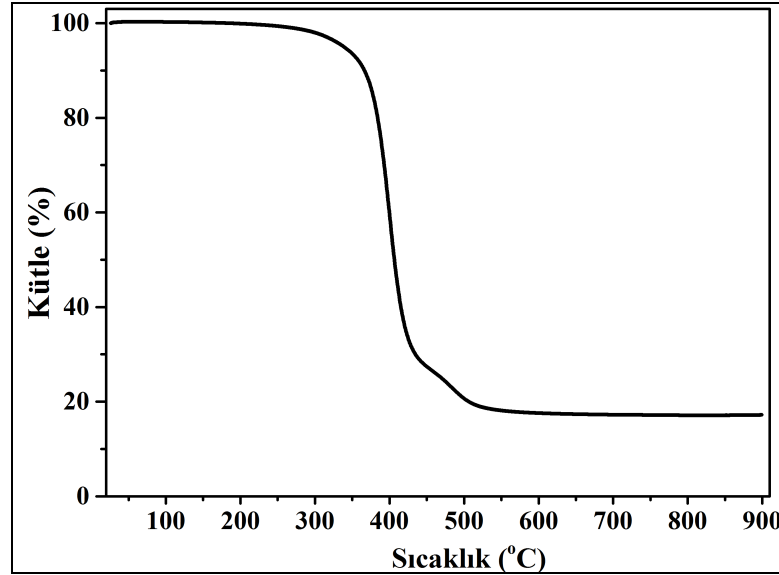
Şekil 5.16: GE-ICS sorbentinin TGA termogramı.
