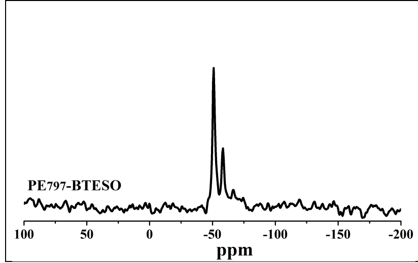
Şekil 5.13: PE797-BTESO polimerinin ^{29}\text{Si} CPMAS NMR spektrumu.
