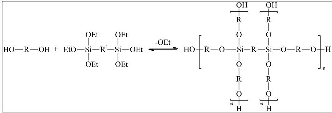
Şekil 2.37: Alkoksisisilanların çapraz bağlanma reaksiyonu.
