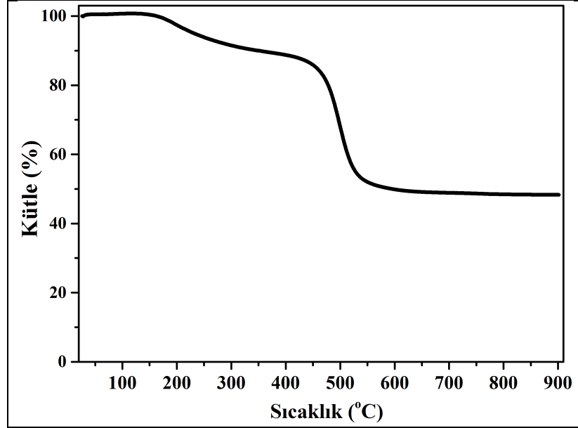
Şekil 5.6: EG-BTESO polimerinin TGA termogramı.
