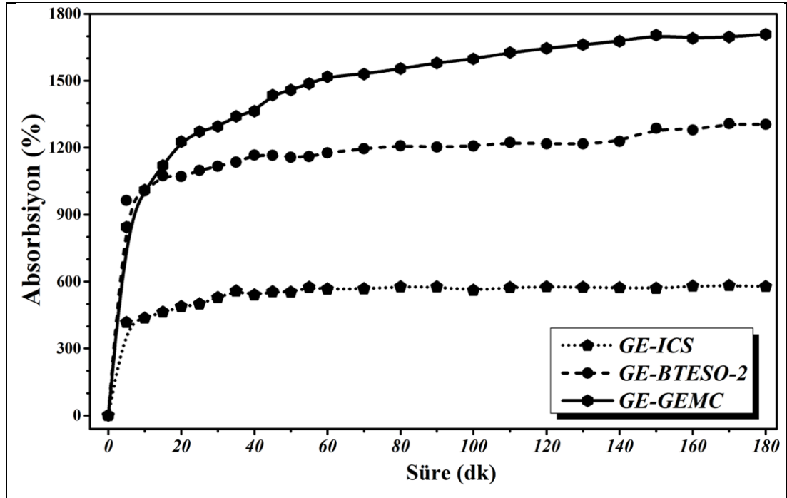
Şekil 6.17: GE esaslı sorbentlerin absorpsiyon kinetik grafiği.
