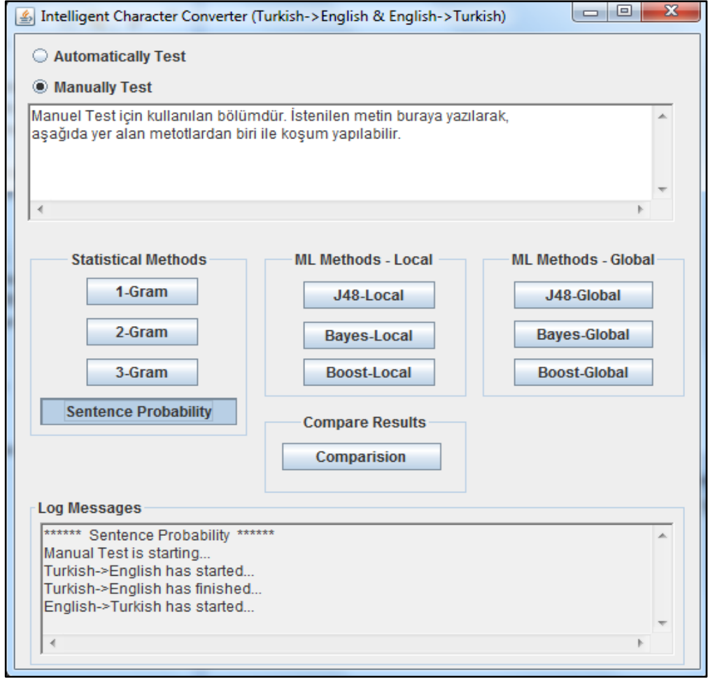
Şekil 7.6: Manuel test.
