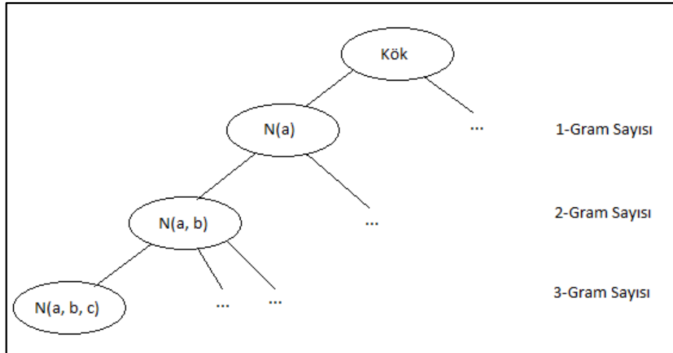
Şekil 5.1: N-Gram ağacı.
